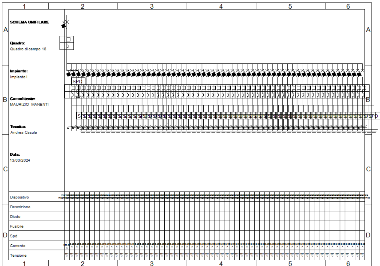
Fig. 23: Schema unifilare quadro "Quadro di campo 18"
