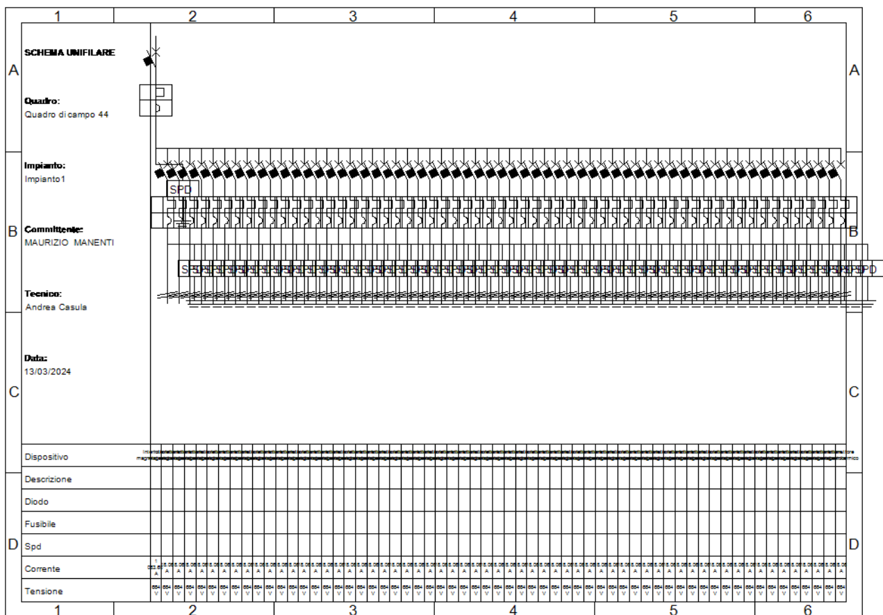
Fig. 49: Schema unifilare quadro "Quadro di campo 44"
