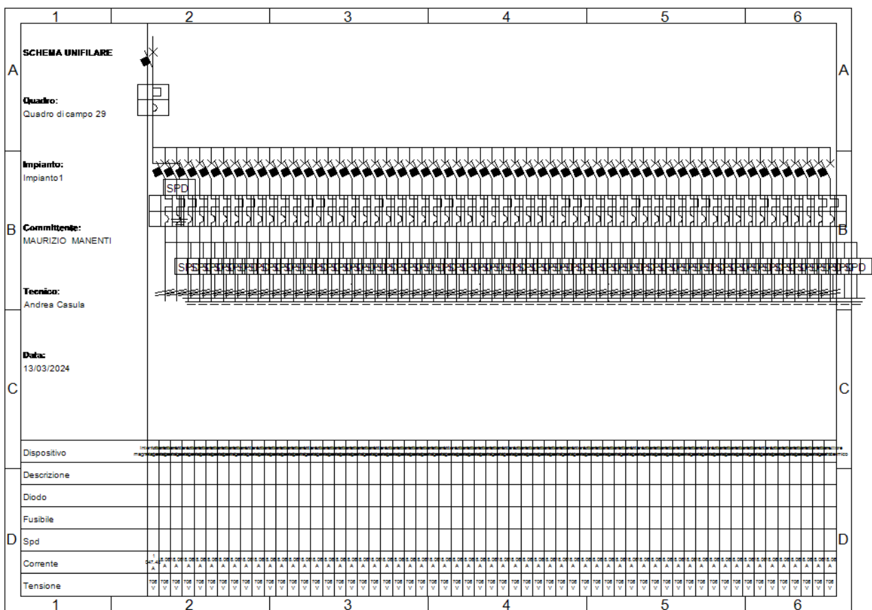
Fig. 34: Schema unifilare quadro "Quadro di campo 29"
