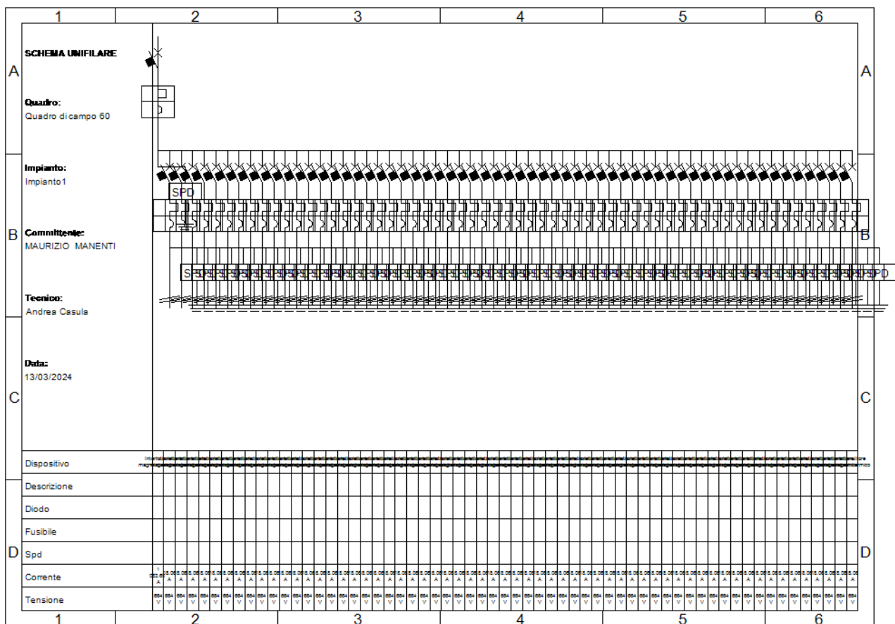
Fig. 65: Schema unifilare quadro "Quadro di campo 60"
