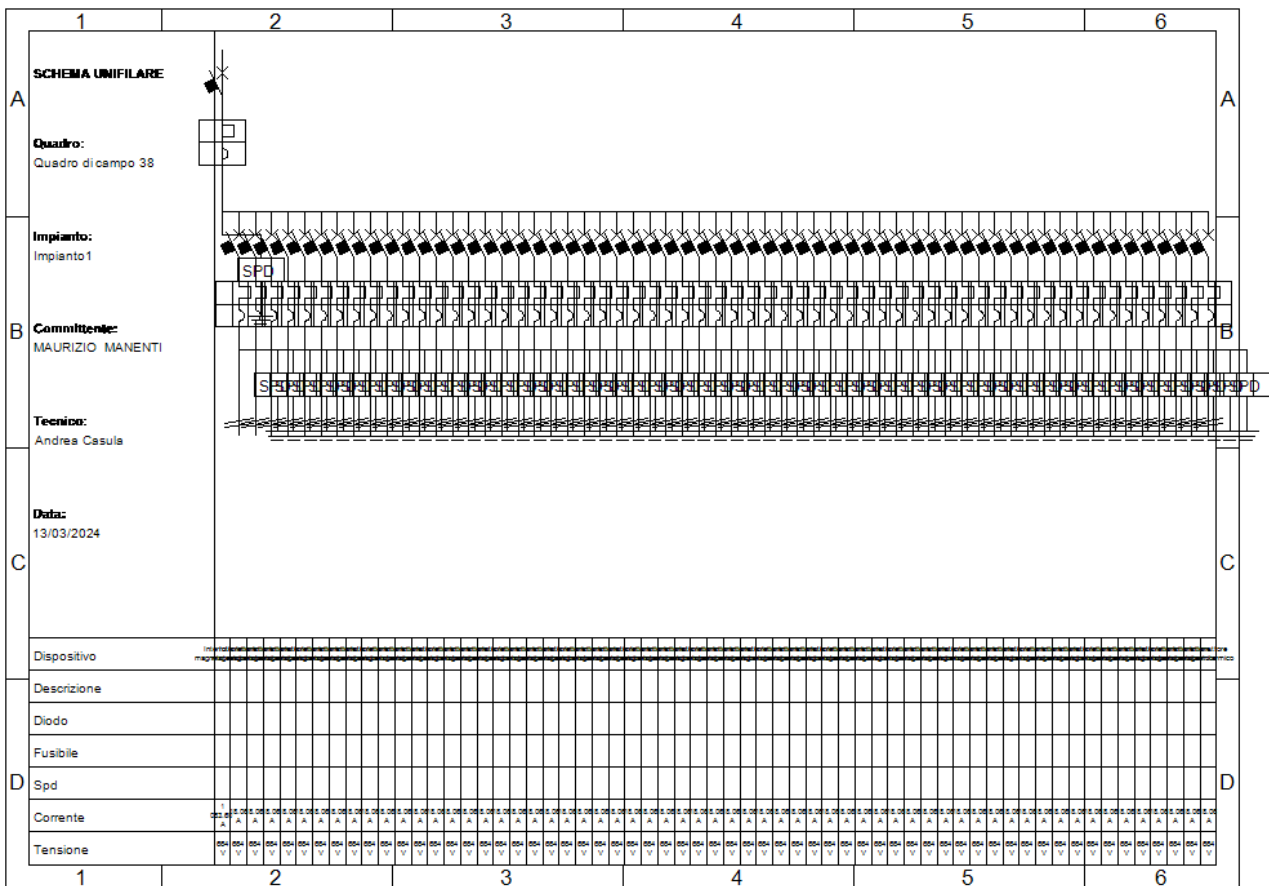
Fig. 43: Schema unifilare quadro "Quadro di campo 38"
