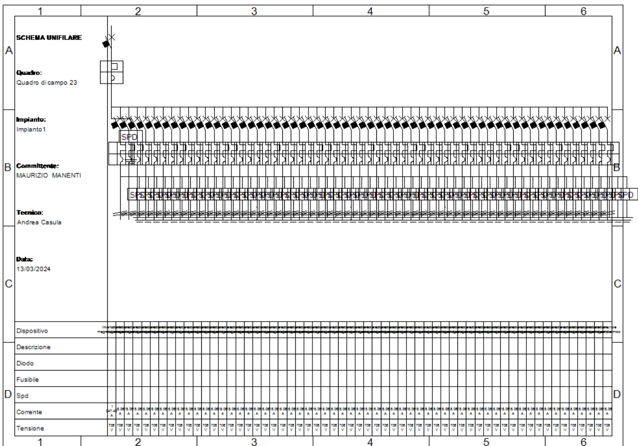
Fig. 28: Schema unifilare quadro "Quadro di campo 23"
