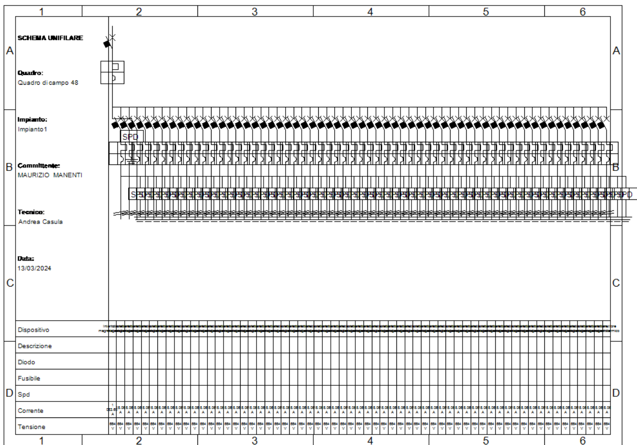
Fig. 53: Schema unifilare quadro "Quadro di campo 48"
