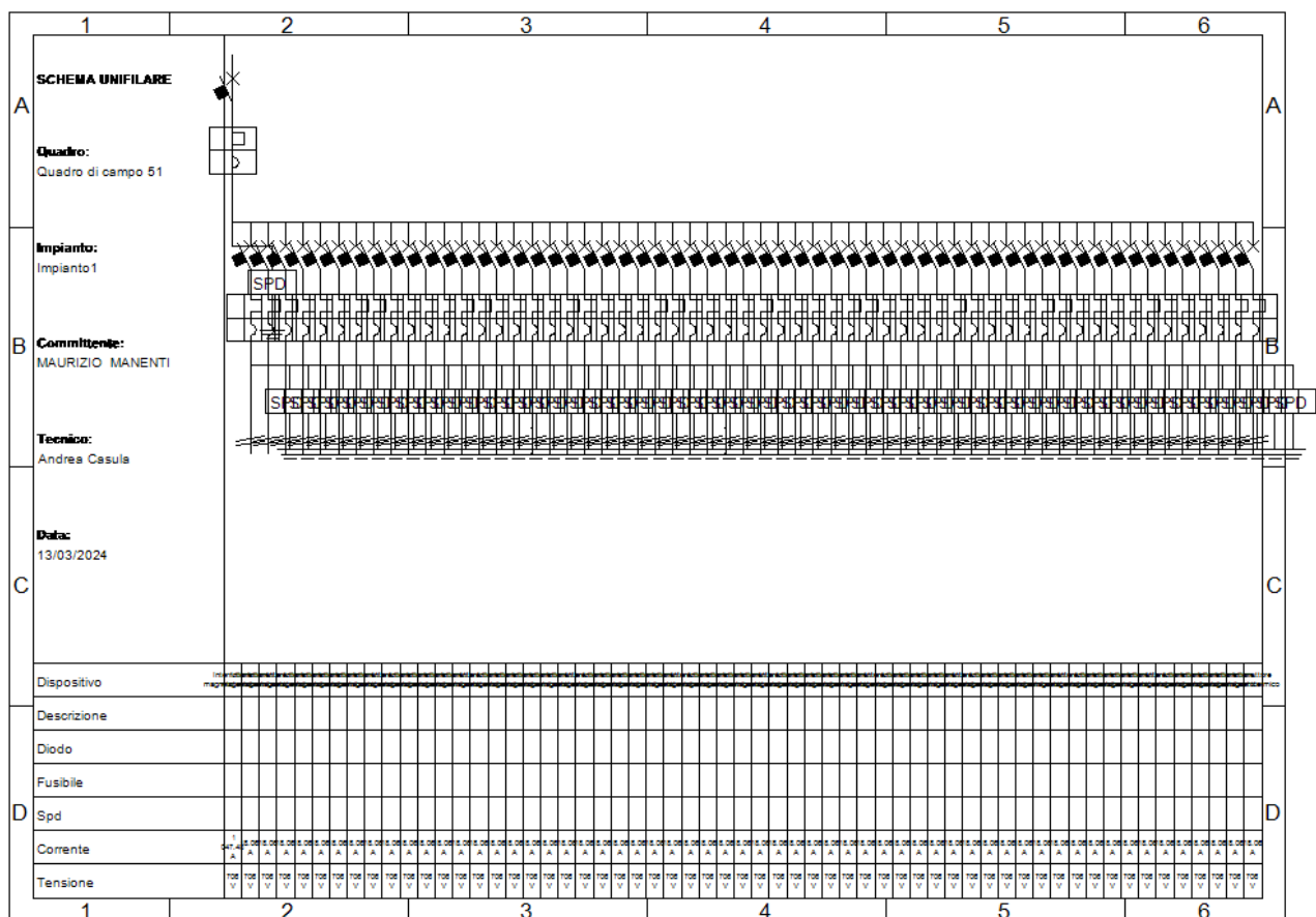
Fig. 56: Schema unifilare quadro "Quadro di campo 51"
