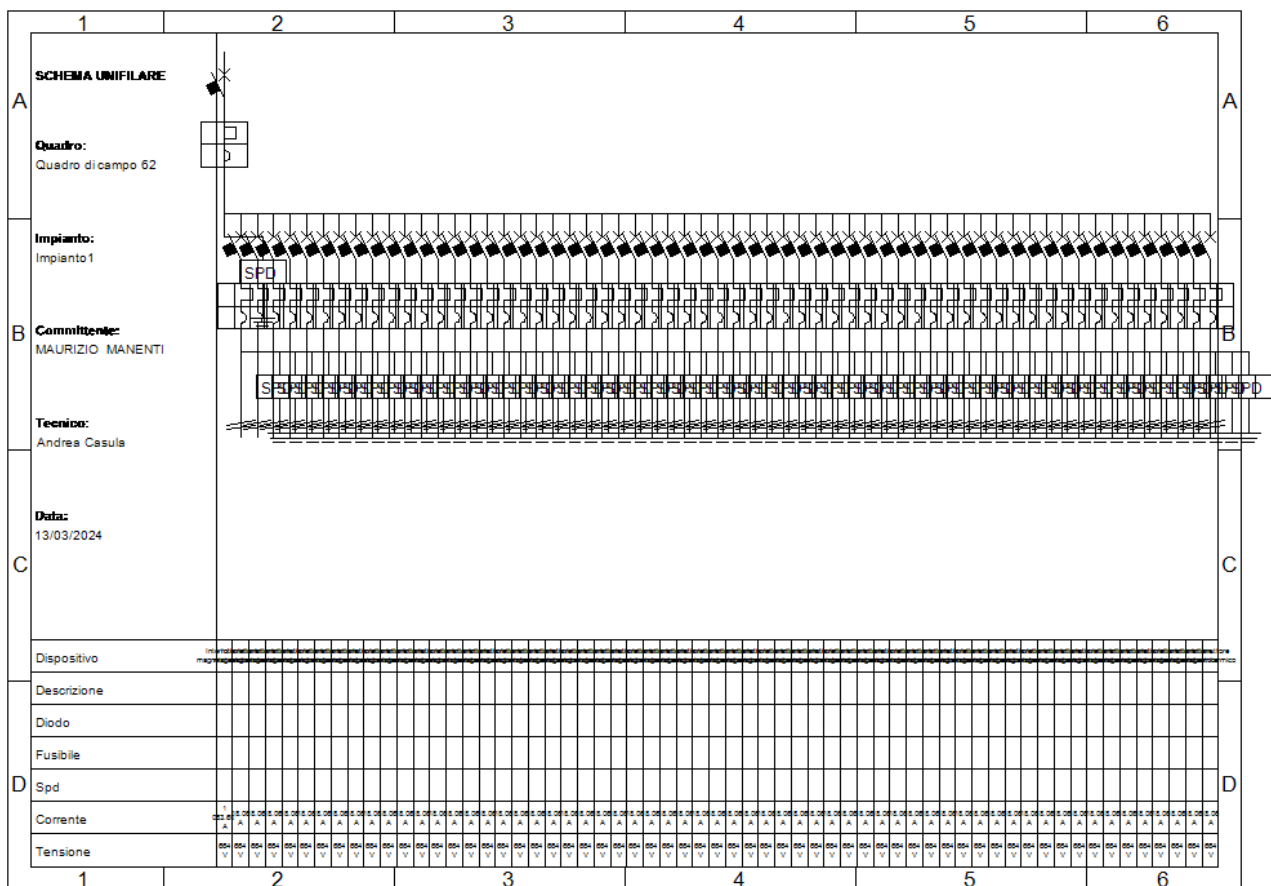
Fig. 67: Schema unifilare quadro "Quadro di campo 62"
