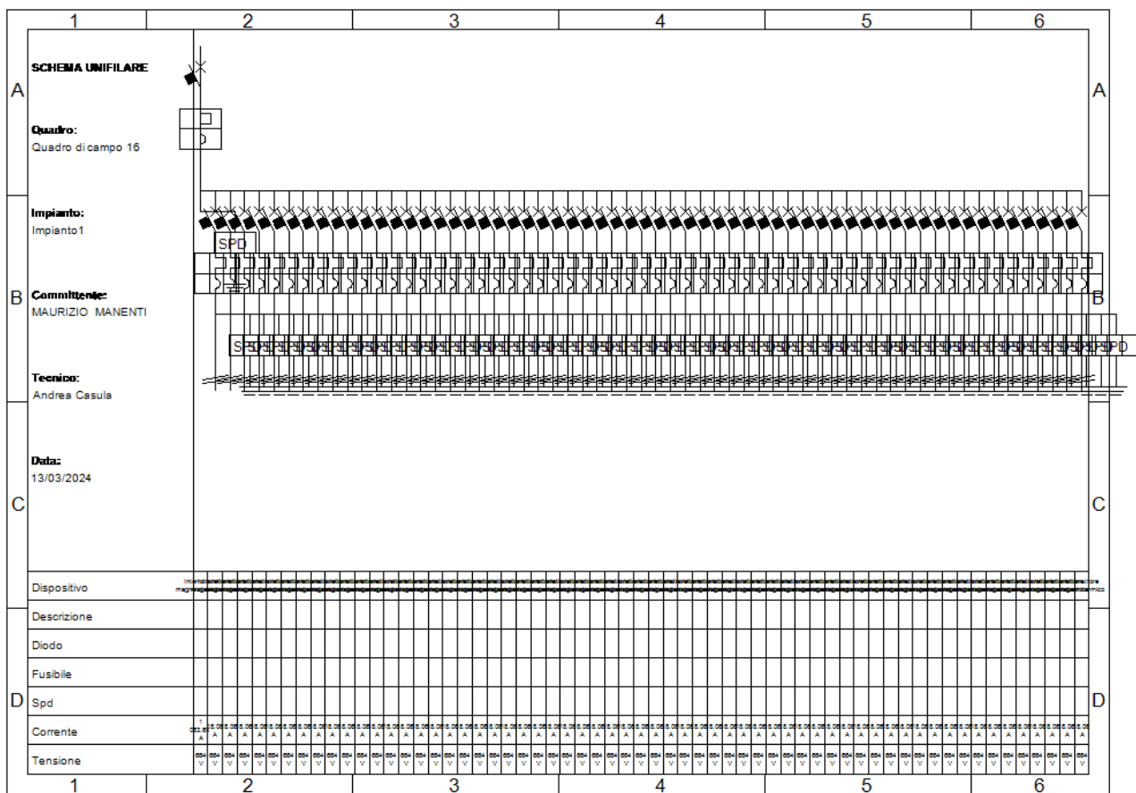
Fig. 21: Schema unifilare quadro "Quadro di campo 16"
