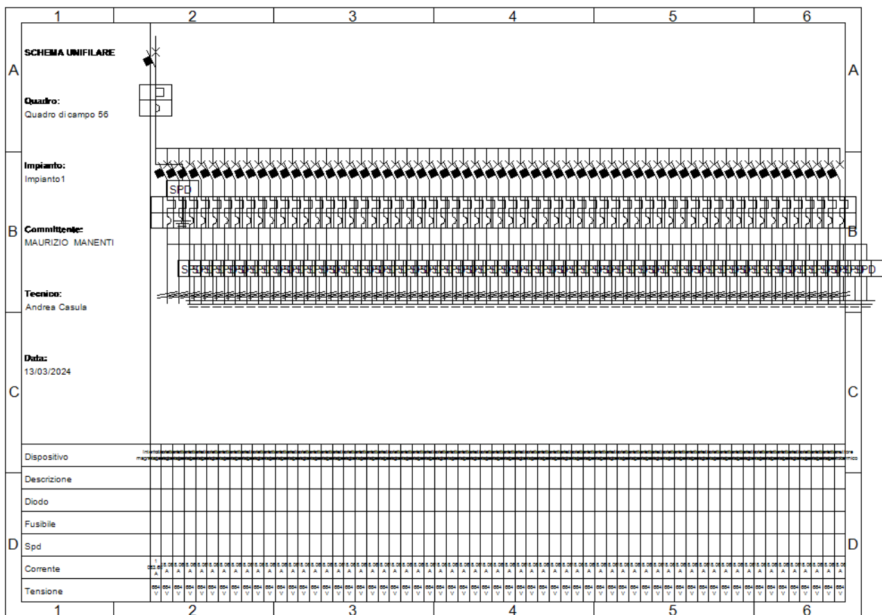
Fig. 61: Schema unifilare quadro "Quadro di campo 56"
