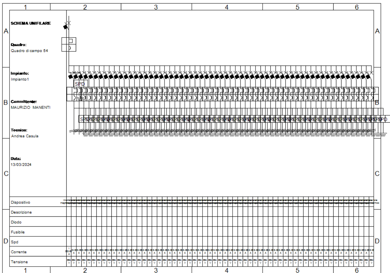
Fig. 59: Schema unifilare quadro "Quadro di campo 54"
