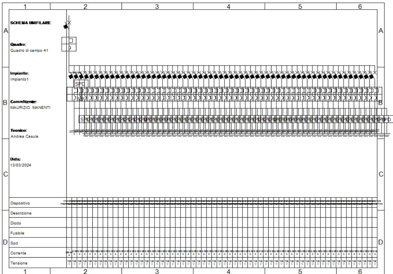
Fig. 46: Schema unifilare quadro "Quadro di campo 41"
