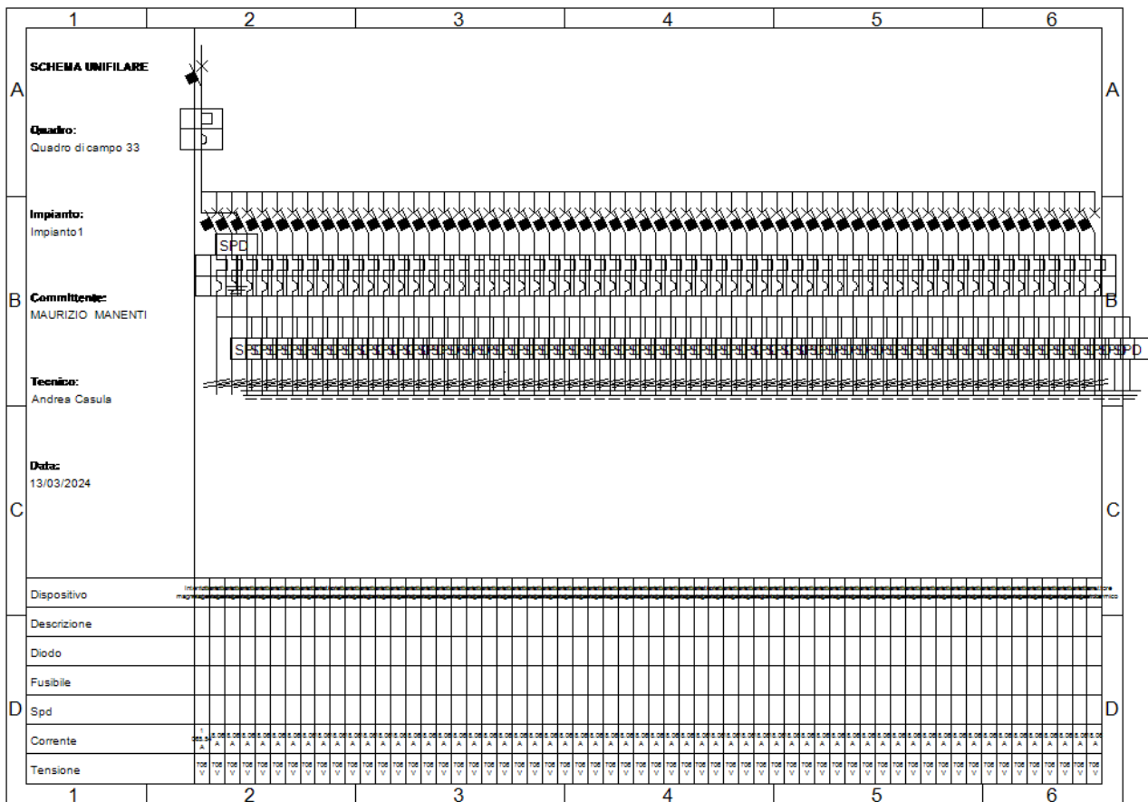
Fig. 38: Schema unifilare quadro "Quadro di campo 33"
