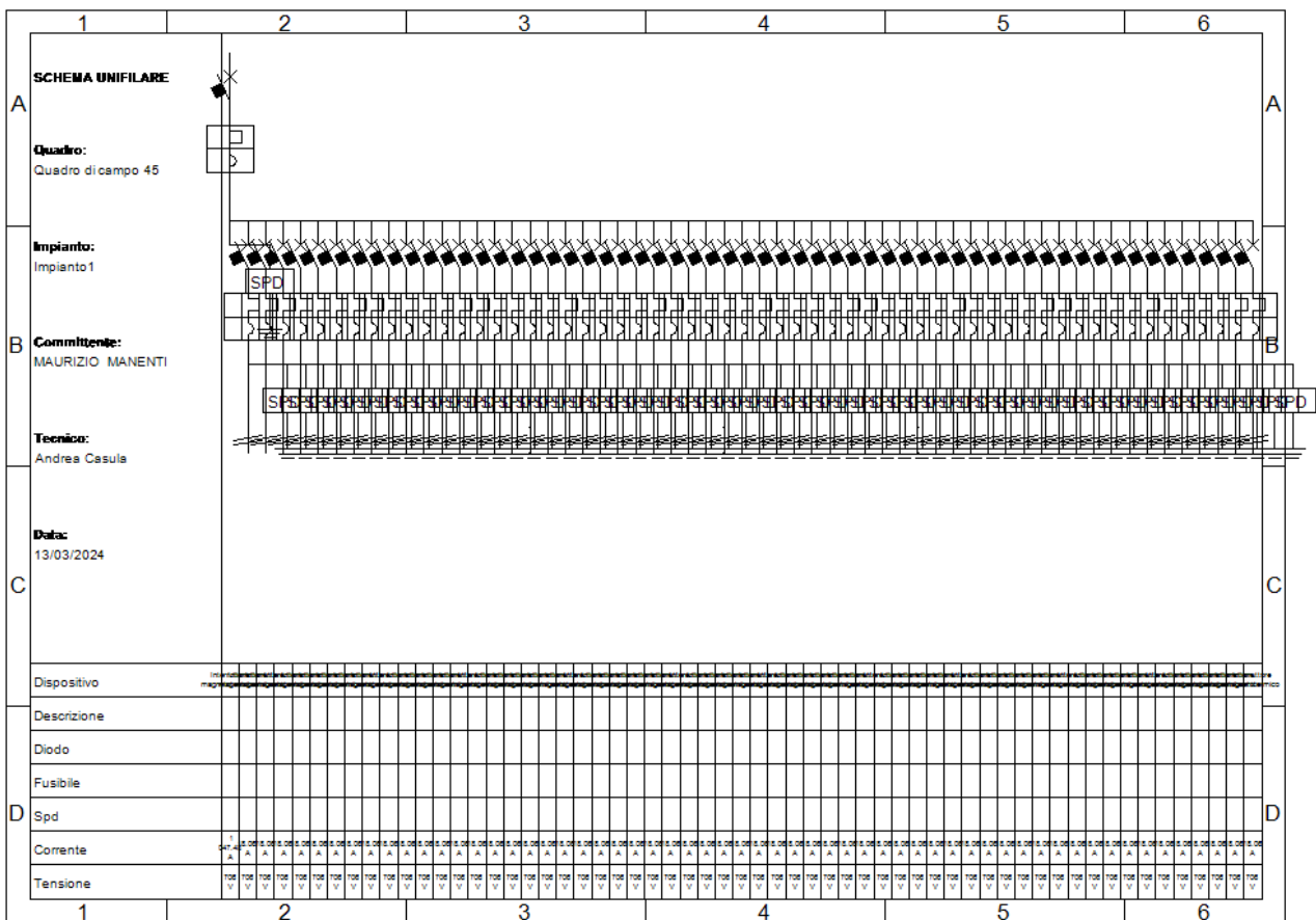
Fig. 50: Schema unifilare quadro "Quadro di campo 45"
