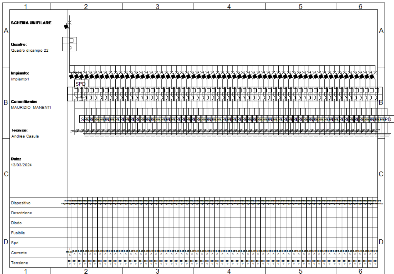
Fig. 27: Schema unifilare quadro "Quadro di campo 22"
