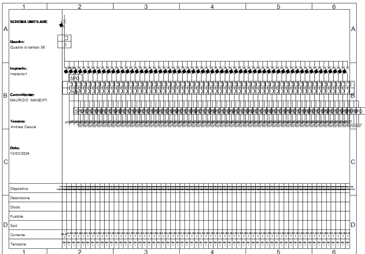
Fig. 41: Schema unifilare quadro "Quadro di campo 36"
