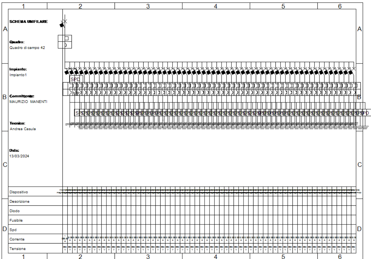
Fig. 47: Schema unifilare quadro "Quadro di campo 42"
