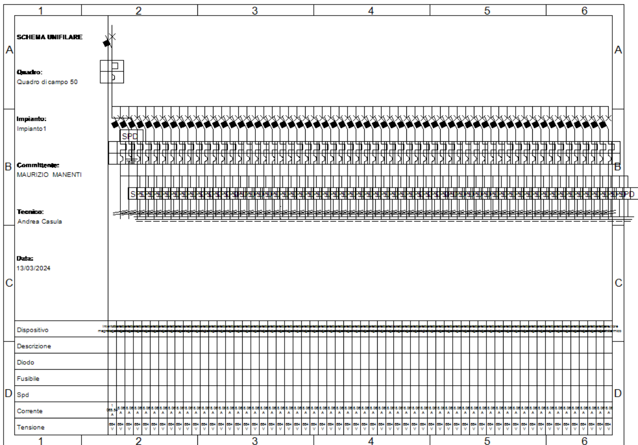
Fig. 55: Schema unifilare quadro "Quadro di campo 50"
