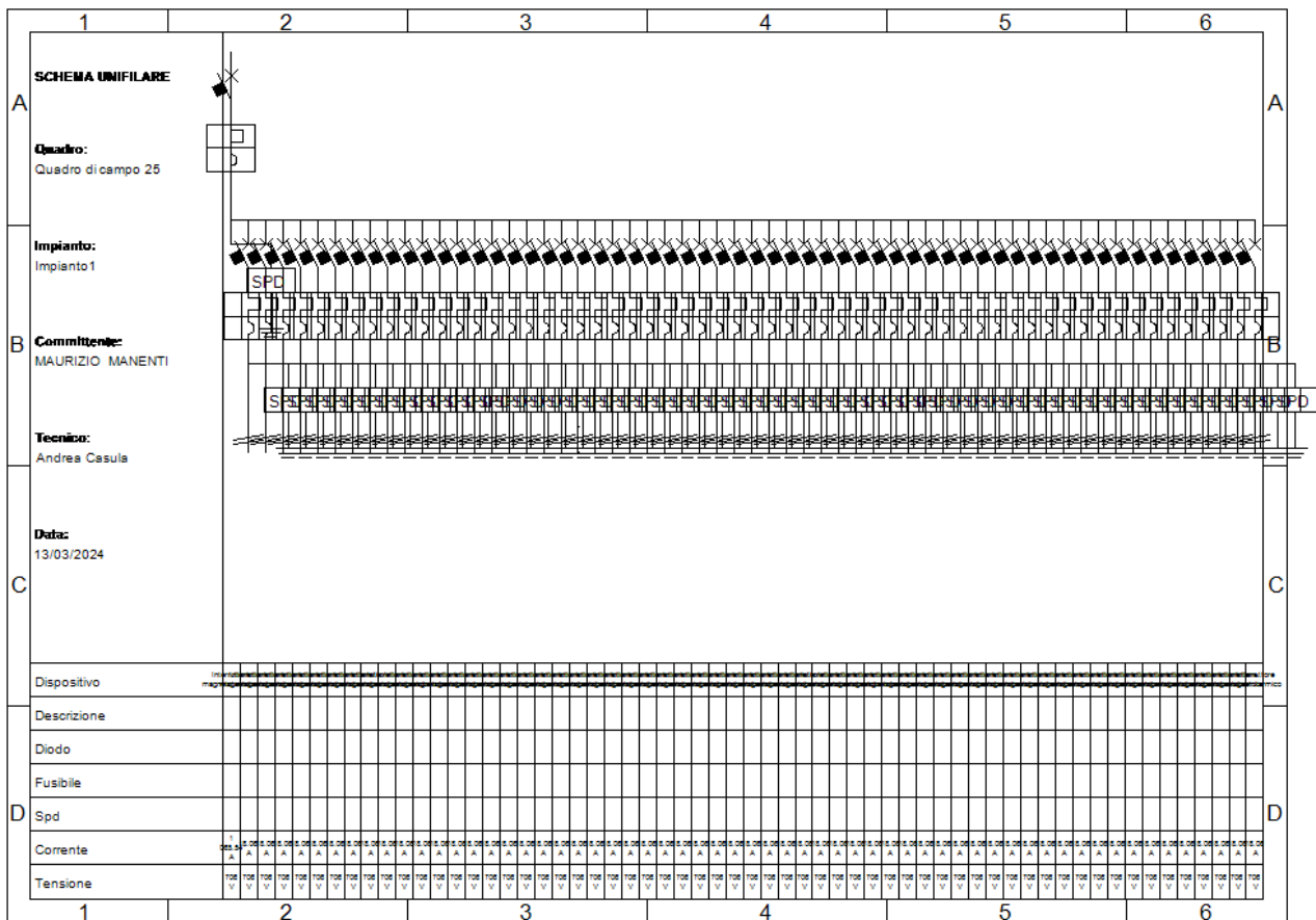
Fig. 30: Schema unifilare quadro "Quadro di campo 25"
