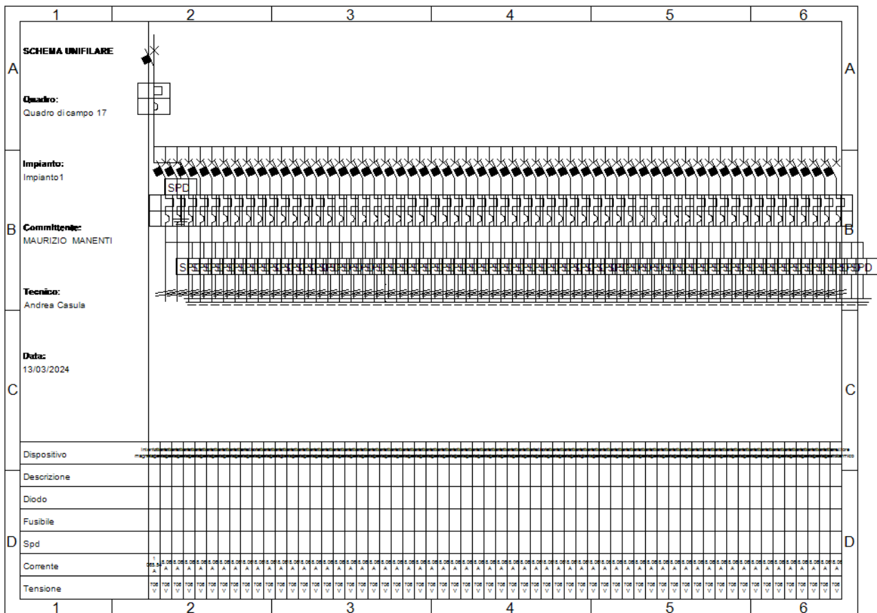
Fig. 22: Schema unifilare quadro "Quadro di campo 17"
