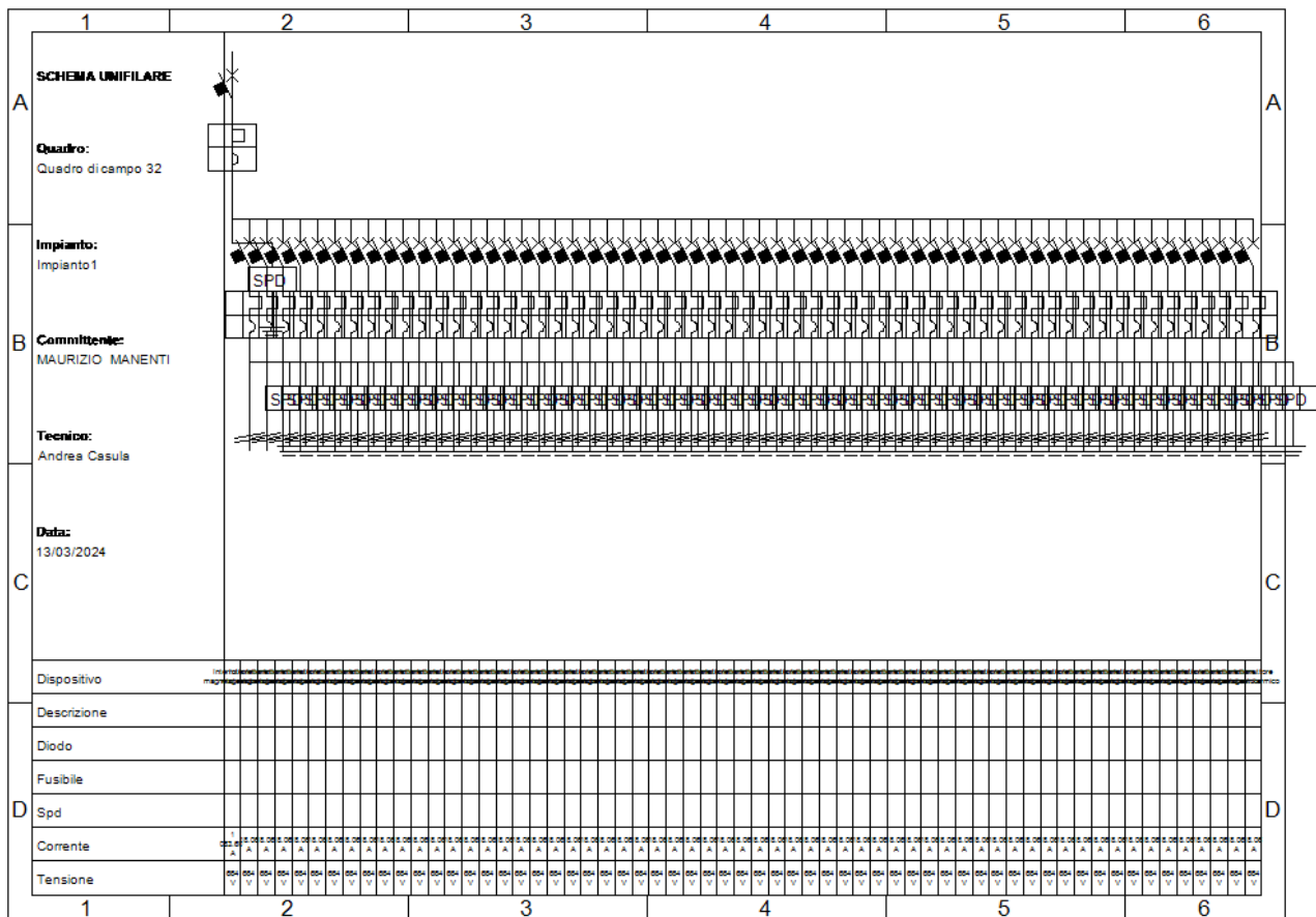
Fig. 37: Schema unifilare quadro "Quadro di campo 32"
