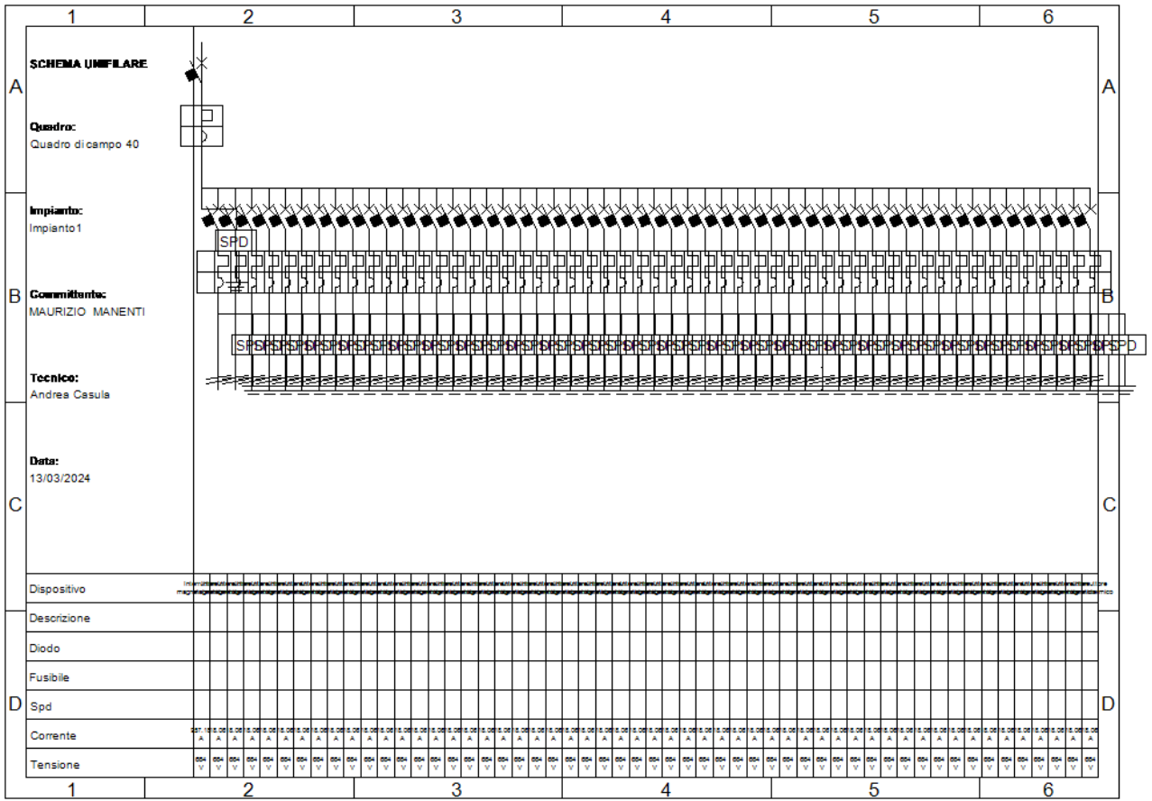
Fig. 45: Schema unifilare quadro "Quadro di campo 40"
