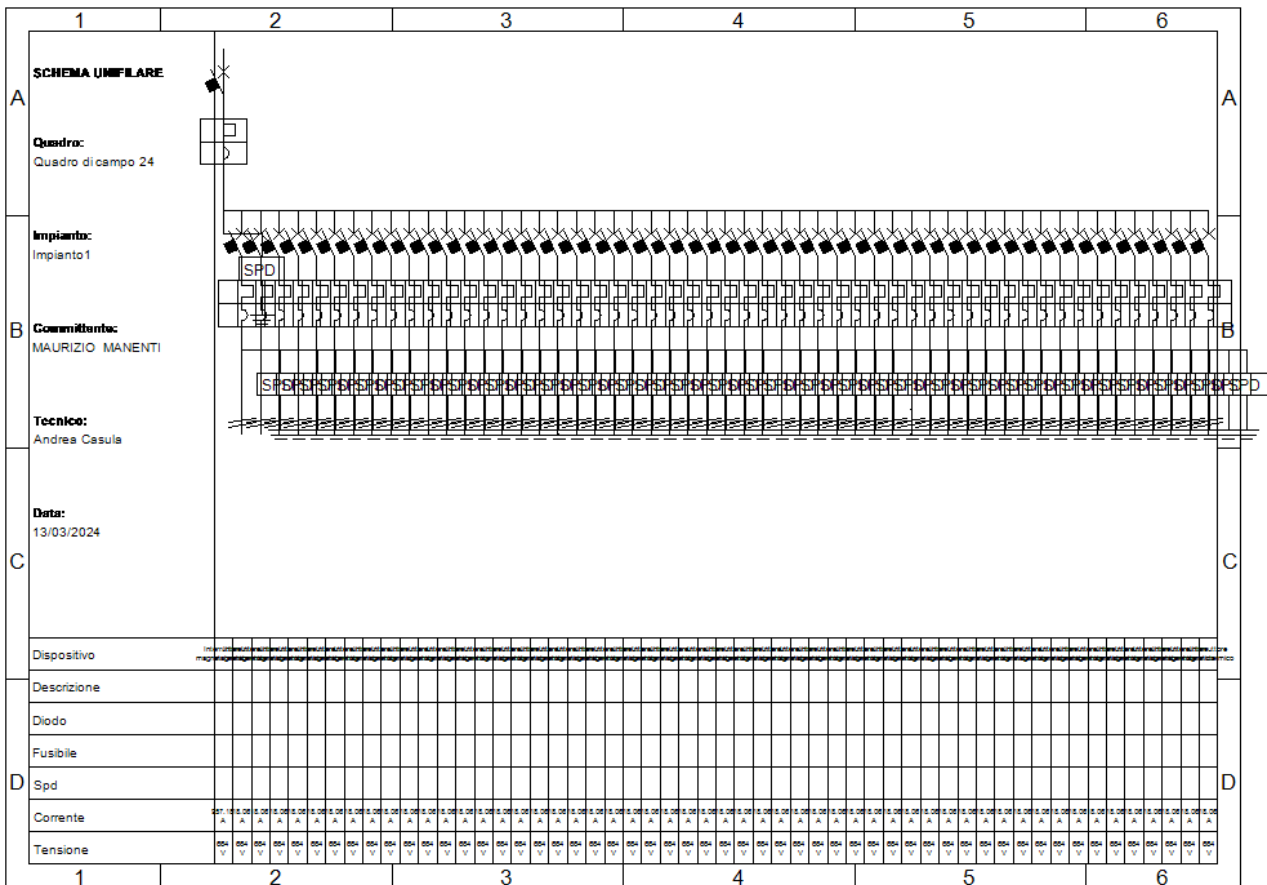
Fig. 29: Schema unifilare quadro "Quadro di campo 24"
