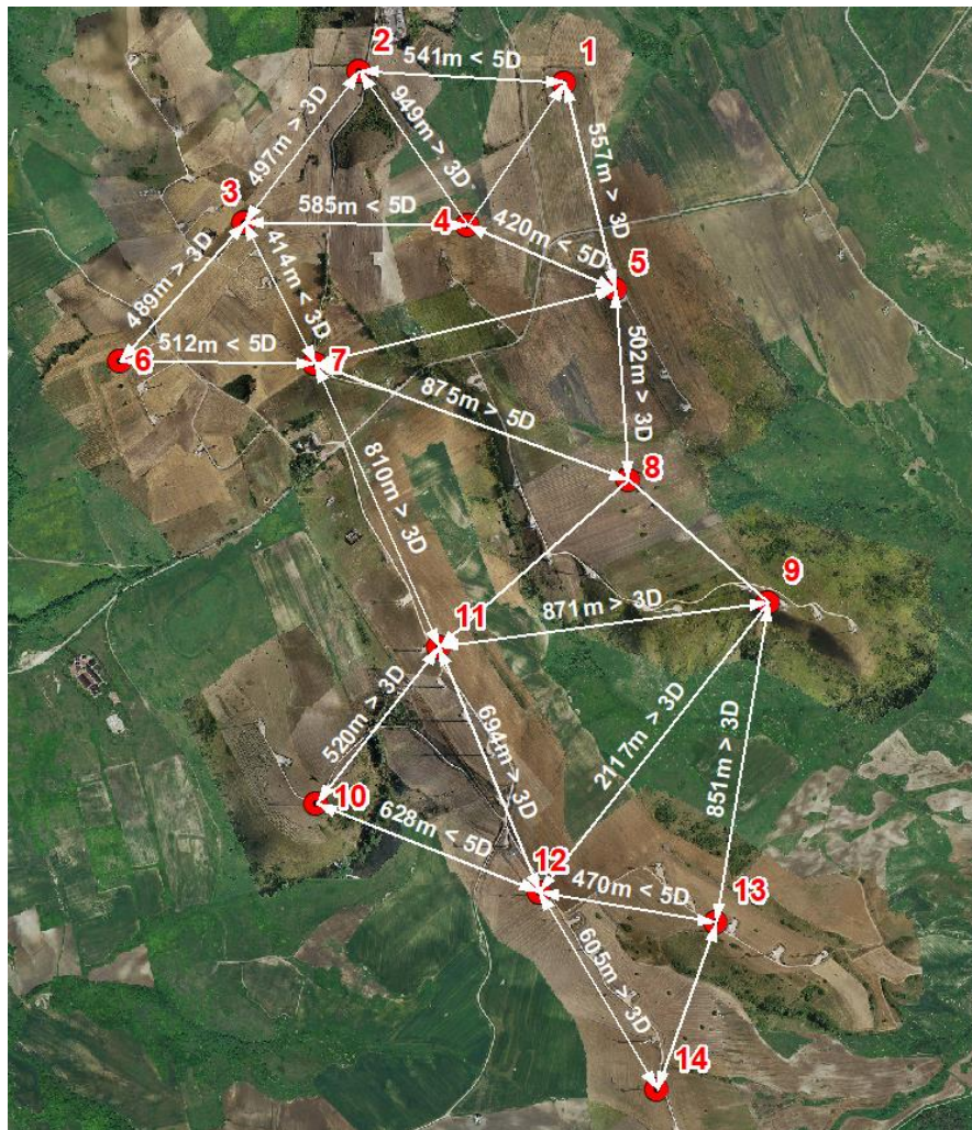
Figura 4 – Schema layout con indicazione delle interdistanze tra le turbine di progetto
