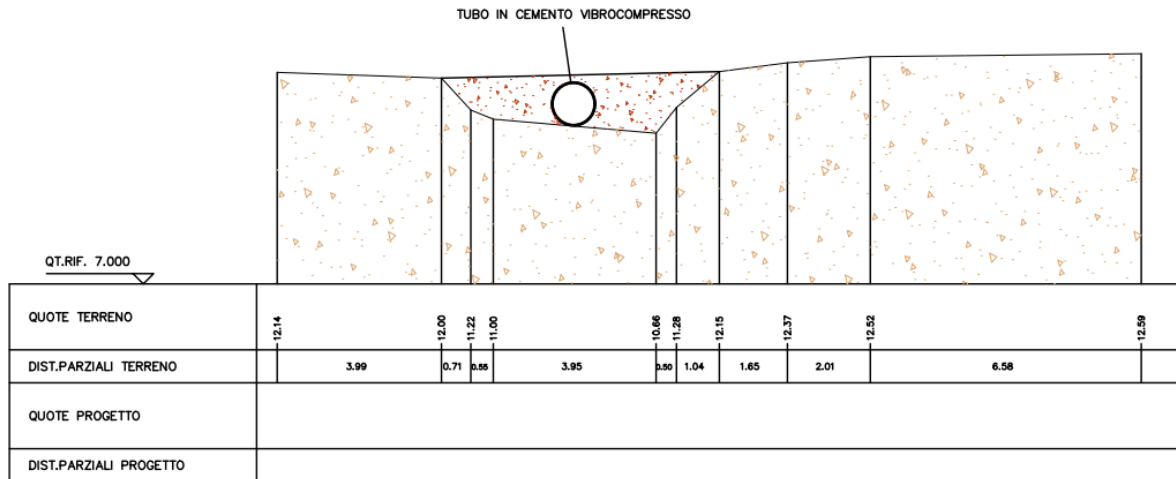
Sezione A-A'
