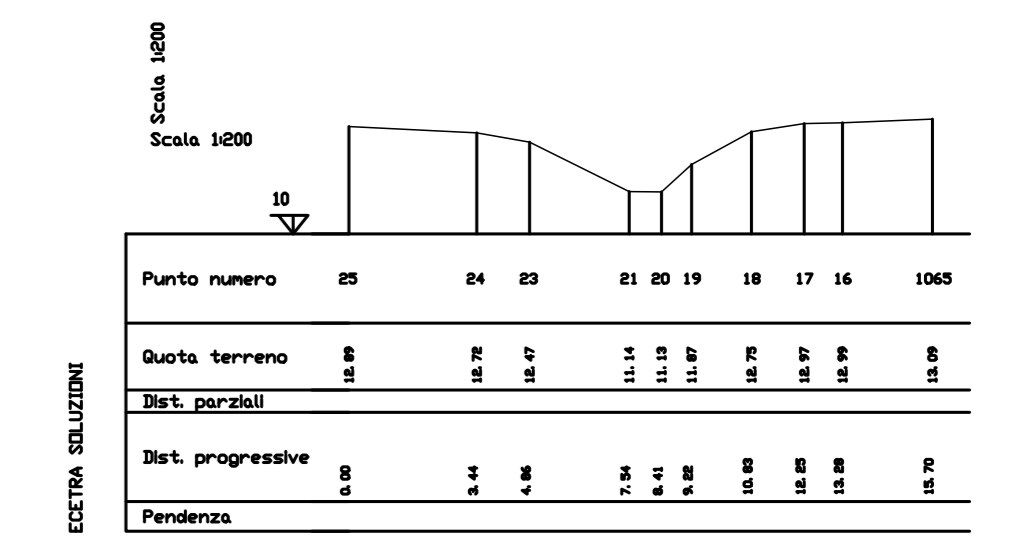
SEZIONE_1 fosso esistente
