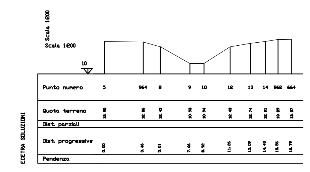
SEZIONE_2 fosso esistente
