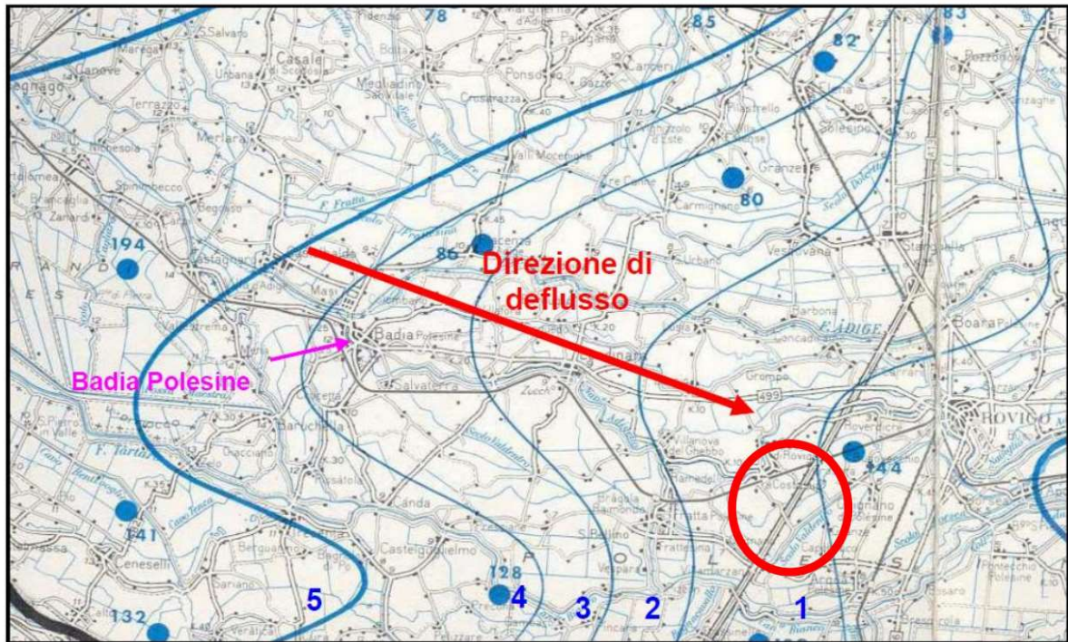
Figura 40 Particolare della Carta Isofreatica redatta a cura della Regione Veneto in base ai rilevamenti del dicembre 1983 (Linee isofreatiche equidistanti 1 metro sul livello medio del mare).
