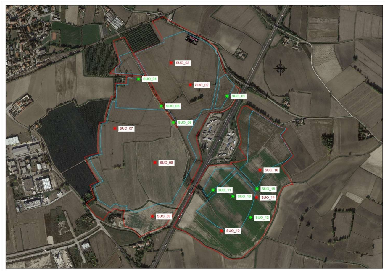
Figura 74 Ubicazione dei punti di campionamento nell'area sotto i pannelli (stazioni con punto rosso) e nelle aree di servizio (stazioni con punto verde) del monitoraggio ante-operam
