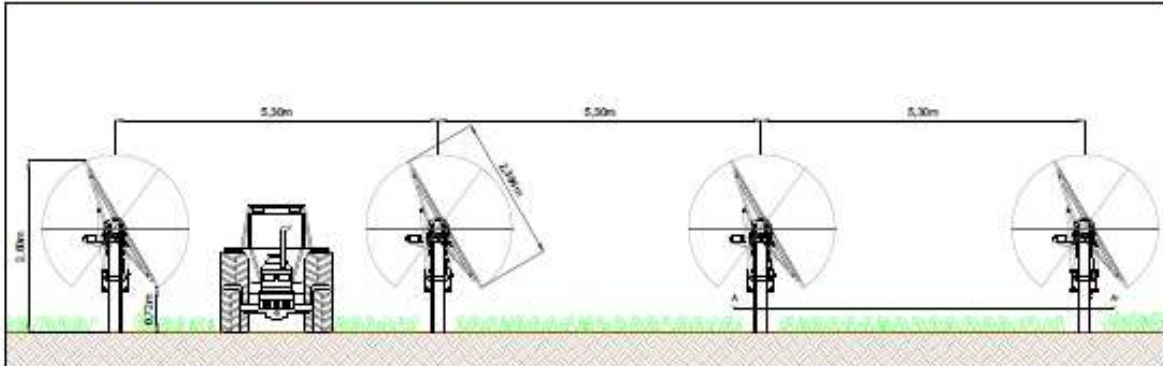
PARTICOLARE STRUTTURE VISTA FRONTALE - Scala 1:50
