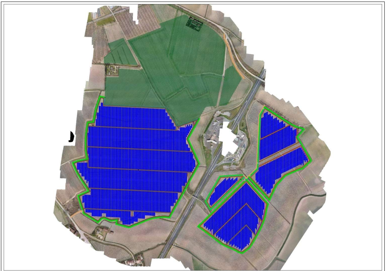
Figura 30 Layout generale dell'impianto
