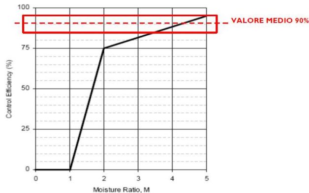
Figura 49 Andamento dell'efficienza di abbattimento delle emissioni in funzione del contenuto di umidità del suolo (Fonte: Linee Guida valutazione emissioni ARPAT)
