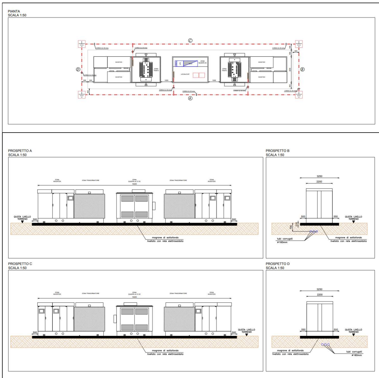
Figura 31 Layout degli inverter
