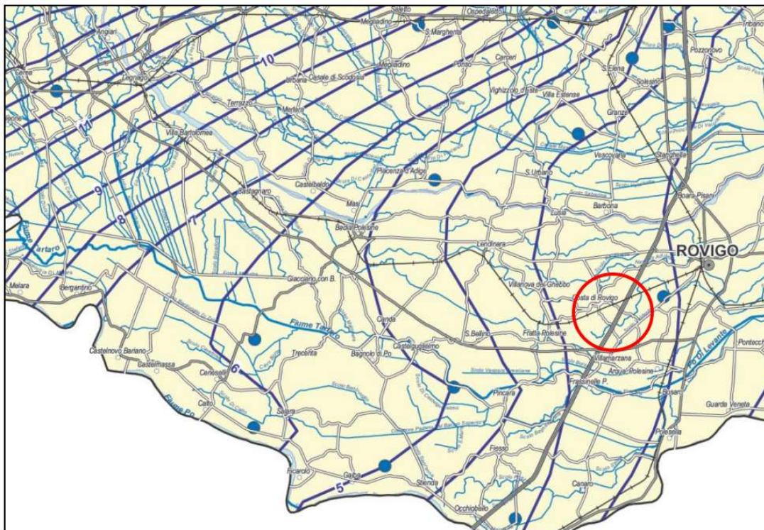
Figura 39 Curve isofreatiche - porzione ovest della provincia di Rovigo
