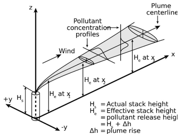
Figura 50 Modello di diffusione gaussiana
