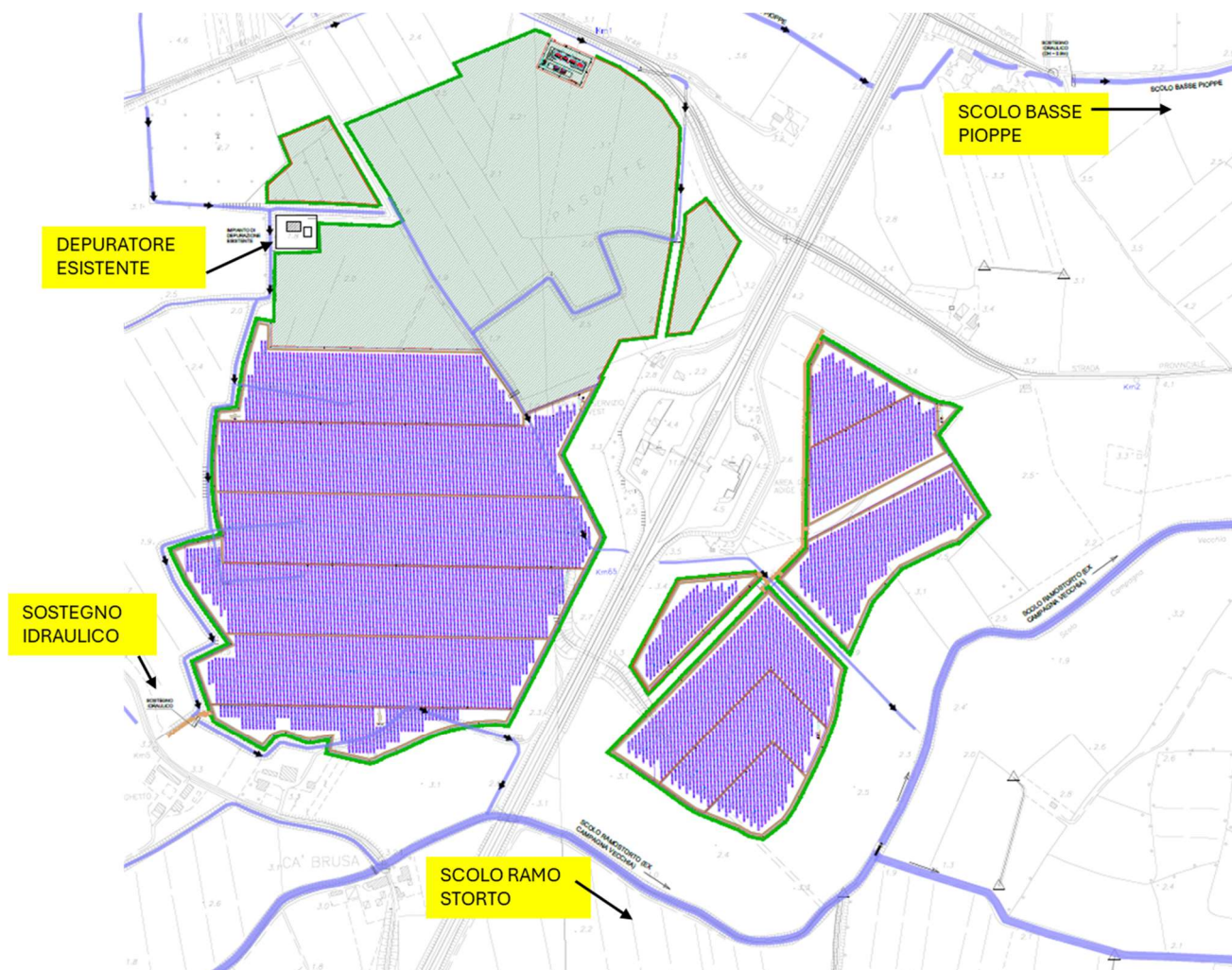
Figura 57 Estratto Tav. Corografia (in allegato al progetto) con indicazione degli scoli privati e dei canali consortili limitrofi
