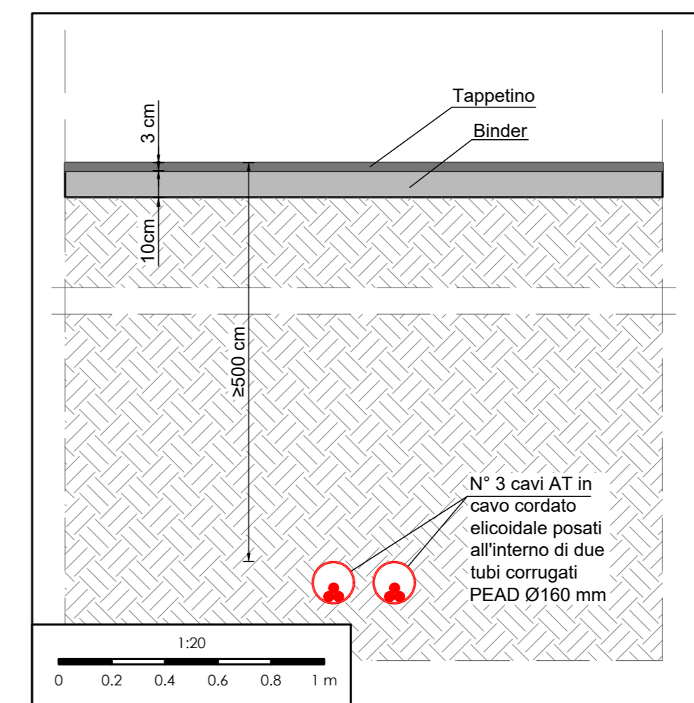
Particolare costruttivo su sede stradale Trivellazione Orizzontale Controllata - Scala 1:20
