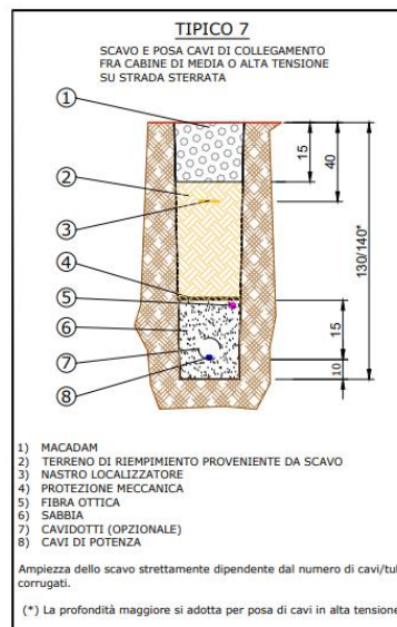
Fig. 8 – Tipici scavi e posa cavi
