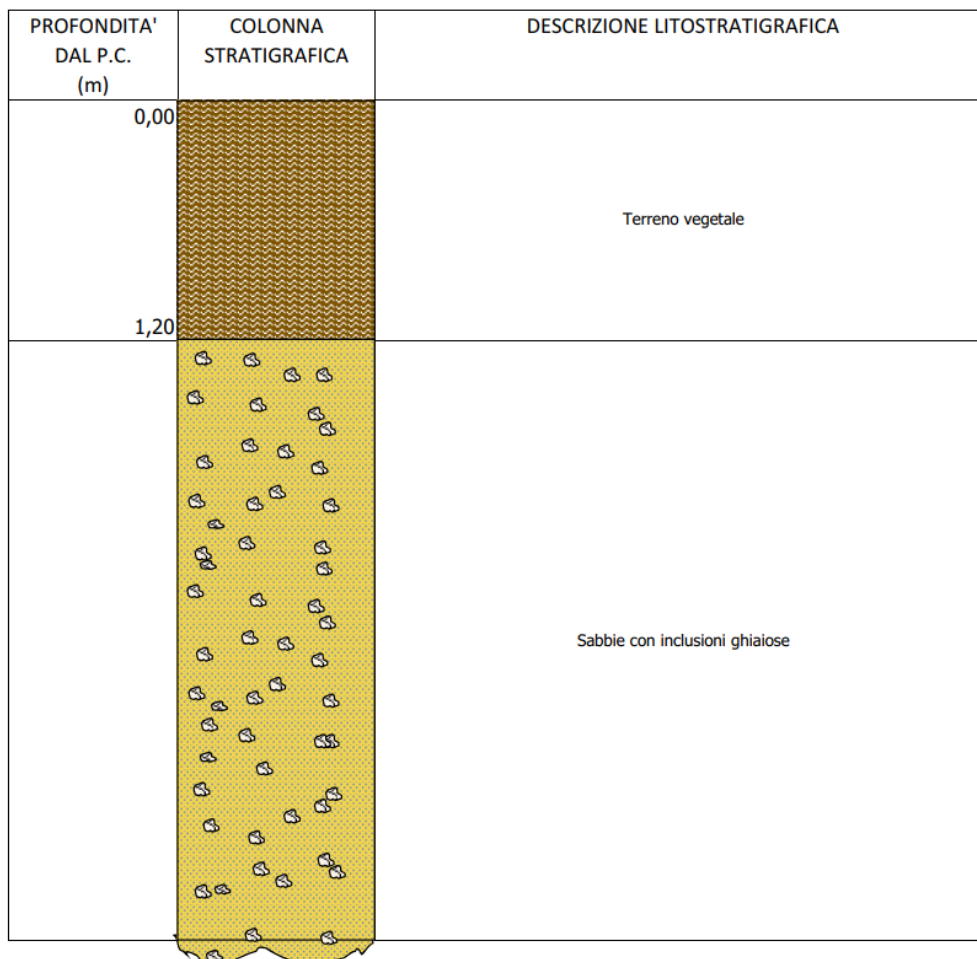
Fig. 6 - COLONNA STRATIGRAFICA: Aree di impianto Nord
