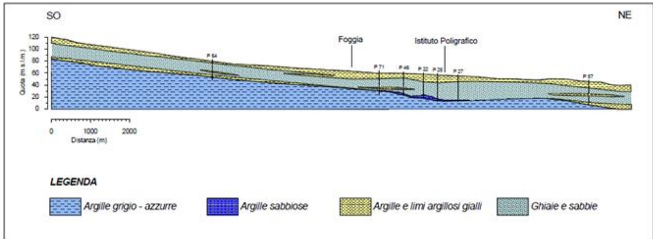
Fig. 5 – Sezione geolitologica del Tavoliere in corrispondenza del tratto medio-basso del bacino idrografico del Torrente Cervaro (da Sollitto, 2006)
