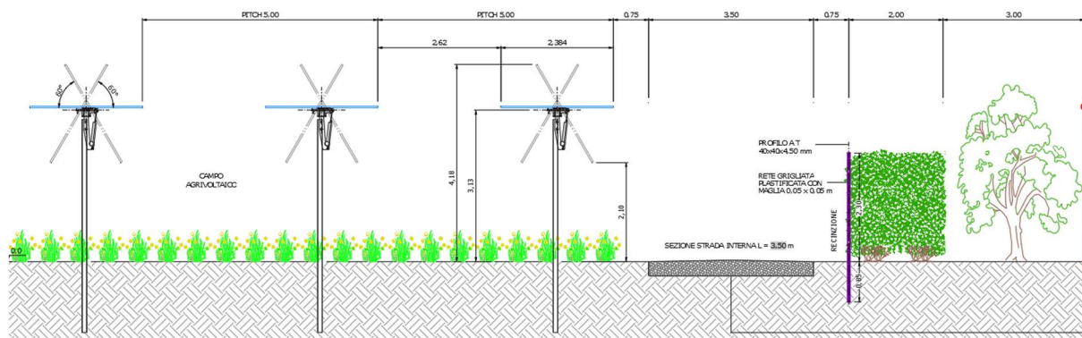
Fig. 2 – Piantumazione tra le file di tracker
