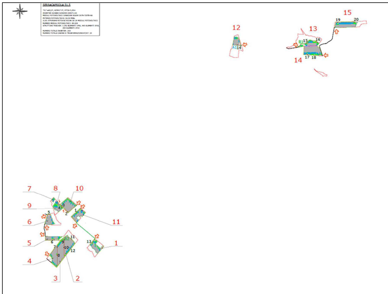
Immagine 2: Planimetria dell'impianto
