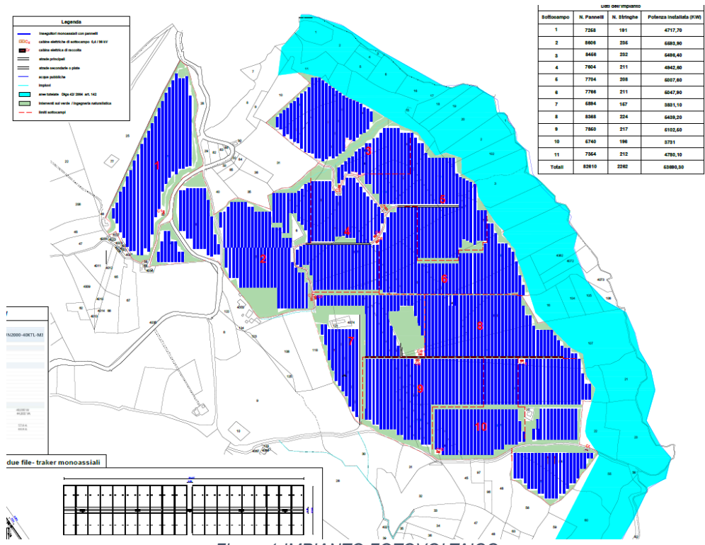
Figura 1 IMPIANTO FOTOVOLTAICO
