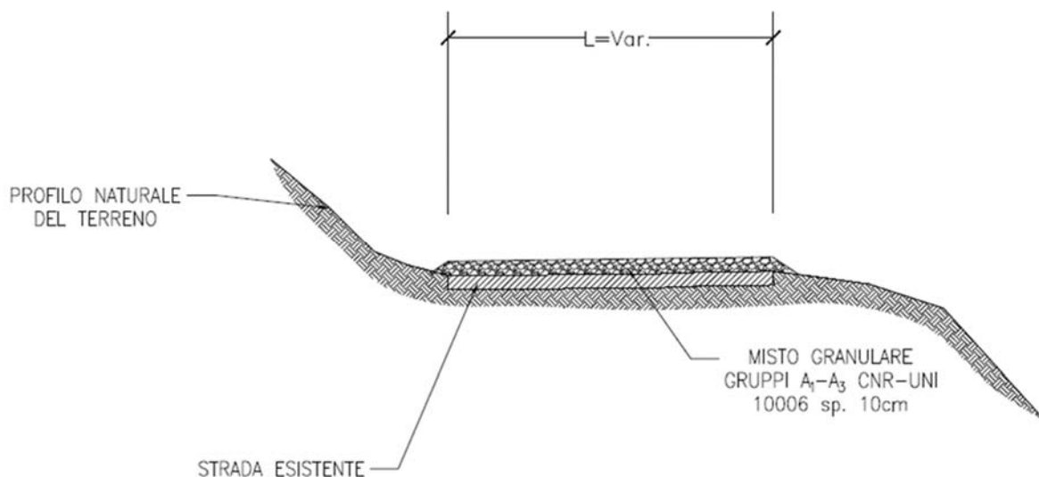
Figura 8: Sezione tipo: ricarica in misto granulare
