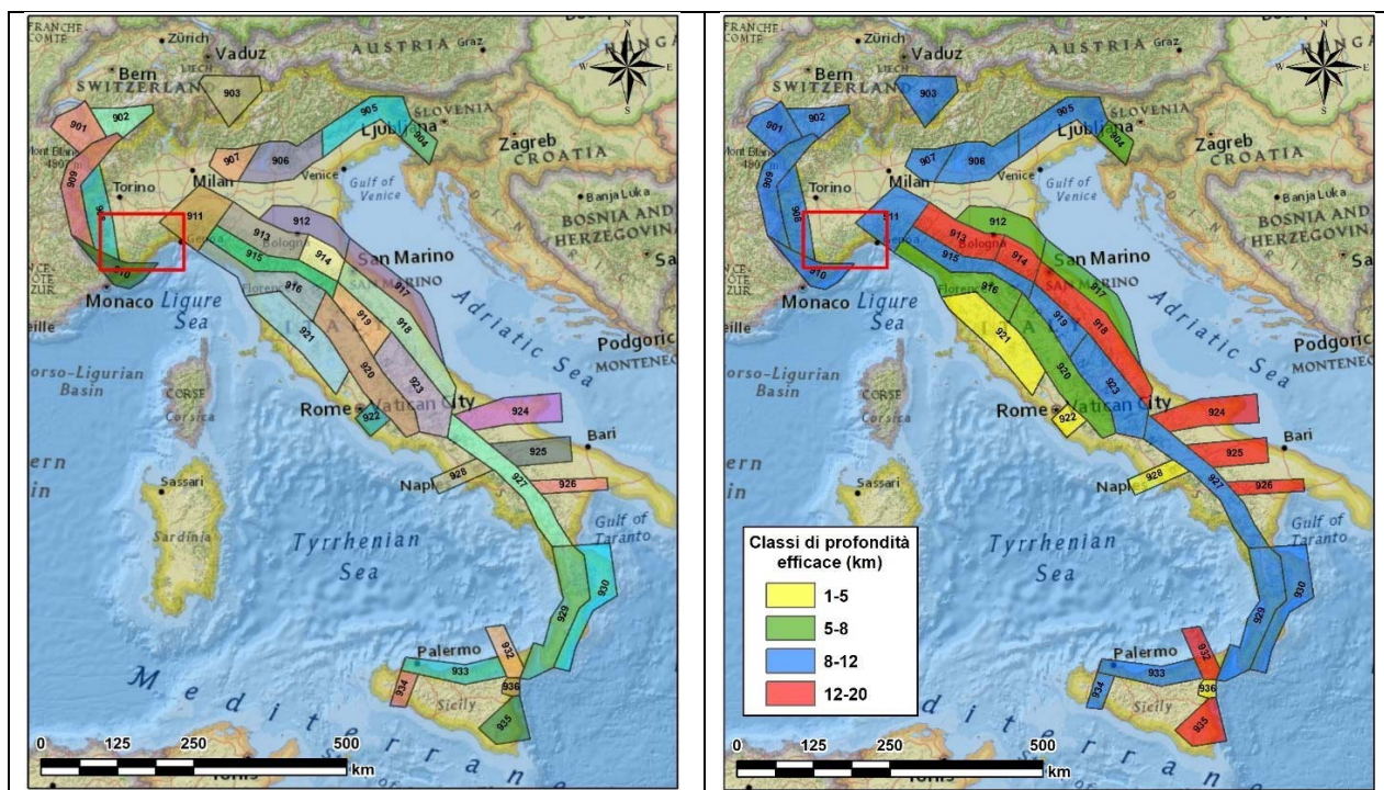
Zonazione sismogenetica ZS9
