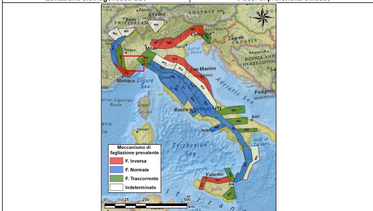
Meccanismo di fagliazione prevalente
