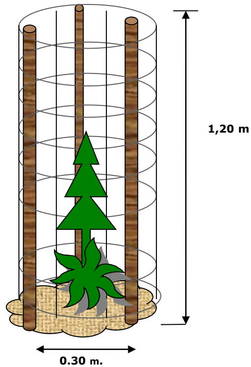
Fig. 7/1 Es. Protezione in rete plastica 1,20 m
