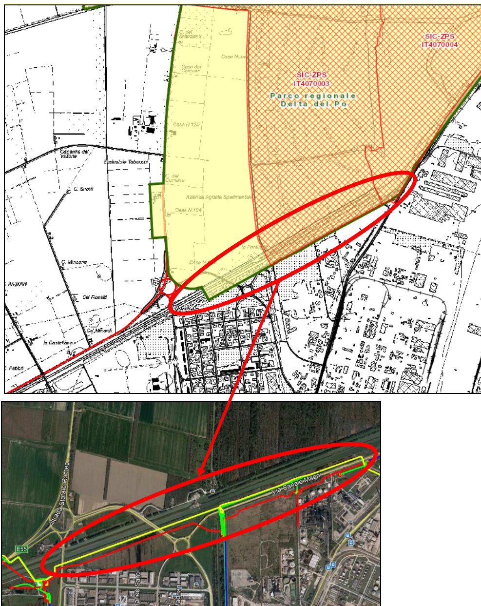
Figura 2/3 – Stralcio Parchi, Aree Protette e Natura 2000 - Geoportale emilia romagna e stralcio foto satellitare (in rosso metanodotti In progetto, in verde metanodotti In dismissione, in blu metanodotti esistenti)
