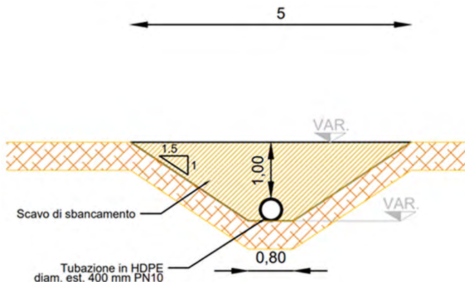
Figura 2-2 - Sezione tipologica dello scavo
