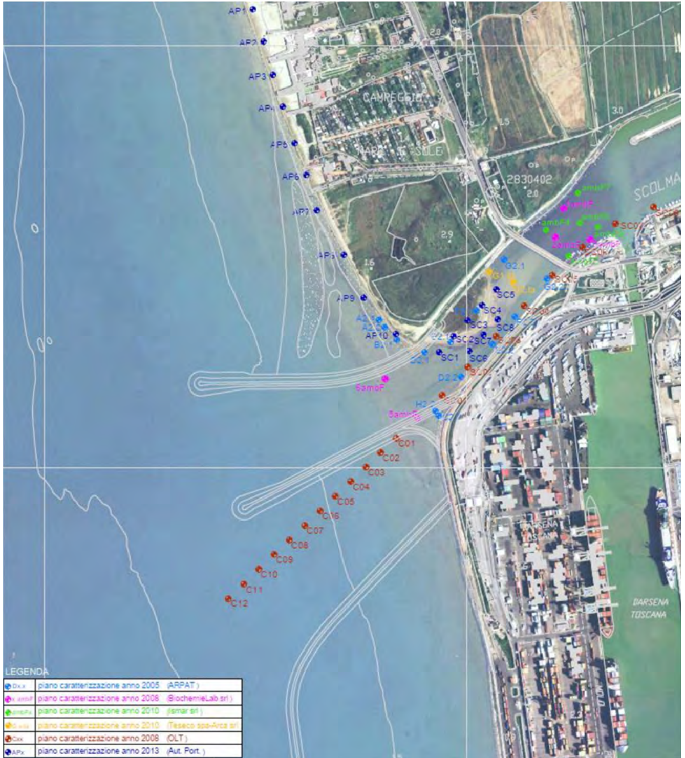
Figura 3-2 - Caratterizzazioni precedenti alla realizzazione dell'armatura di foce
