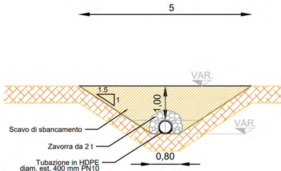
Figura 2-3 - Sezione tipologica dello scavo con gabbione
