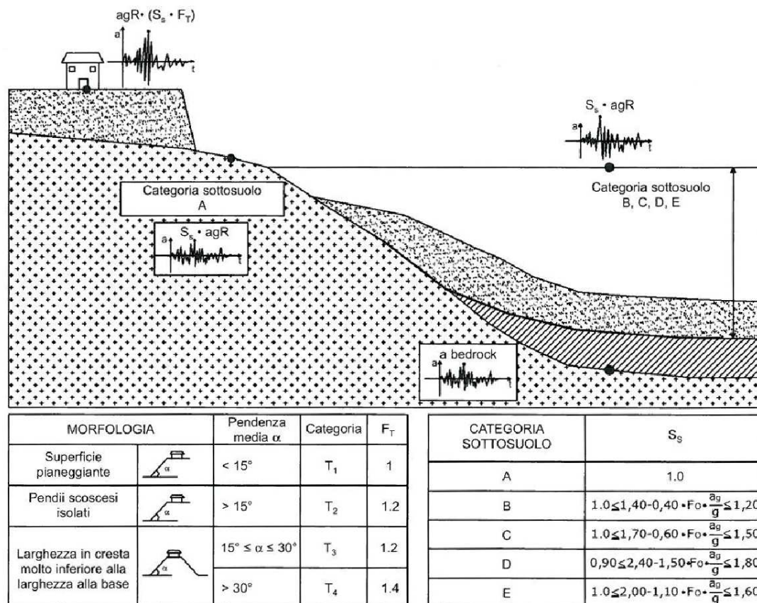
Figura 8 - Rappresentazione schematica del significato delle accelerazioni, delle classi di categoria di suolo e del fattore topografico (da Microsism - procedure automatiche di microzonazione sismica, Giulio Riga)
