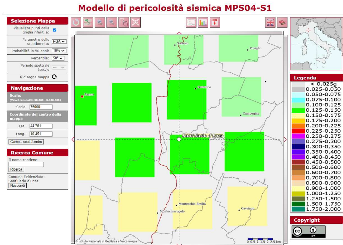
Figura 7 - Stralcio della mappa interattiva di pericolosità sismica del territorio. I punti visualizzati si riferiscono a: parametro dello scuotimento a(g) ; probabilità di superamento del 10% in 50 anni.
