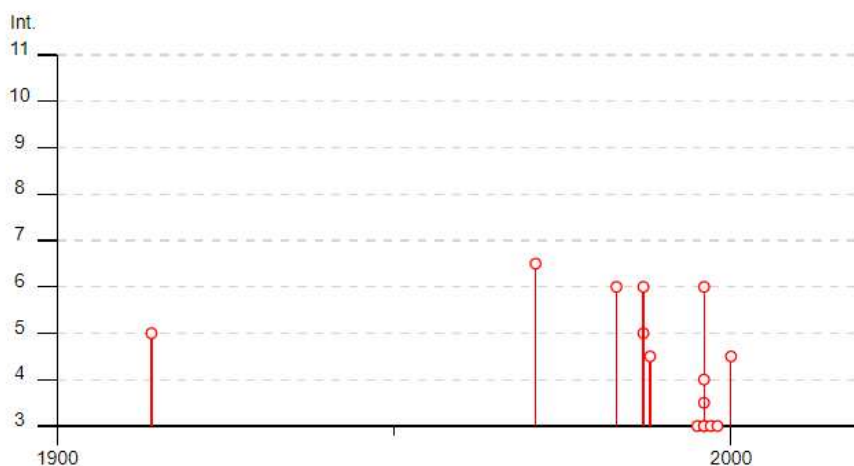
Figura 4 - Rappresentazione grafica della storia sismica del Comune di Sant'Ilario d'Enza (RE)
