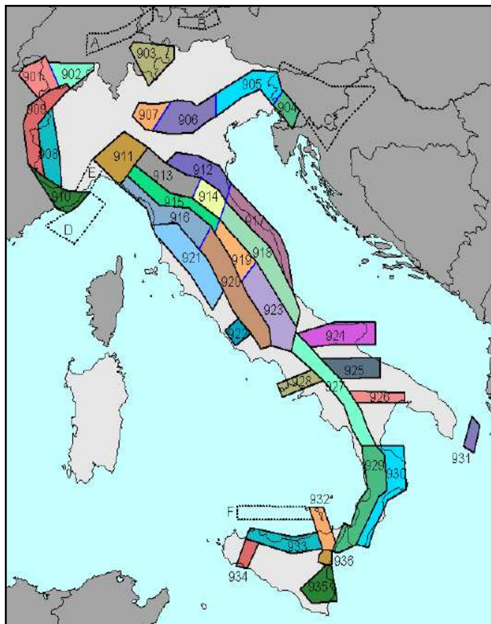
Figura 5 - Zonazione Sismogenetica ZS9
