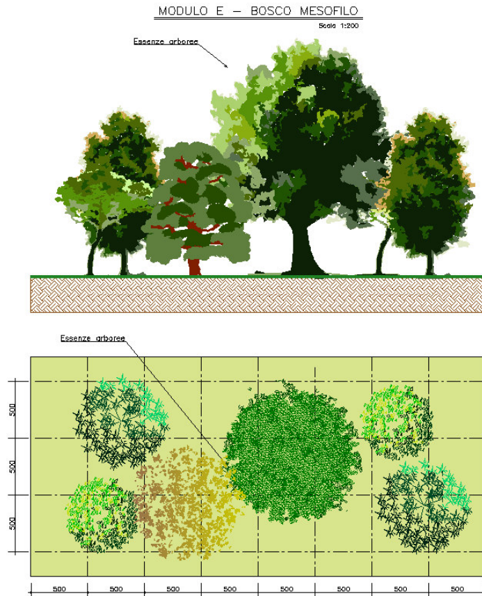
Figura 4-6 – MODULO E – Bosco mesofilo: sesto d'impianto e sezione tipologica
