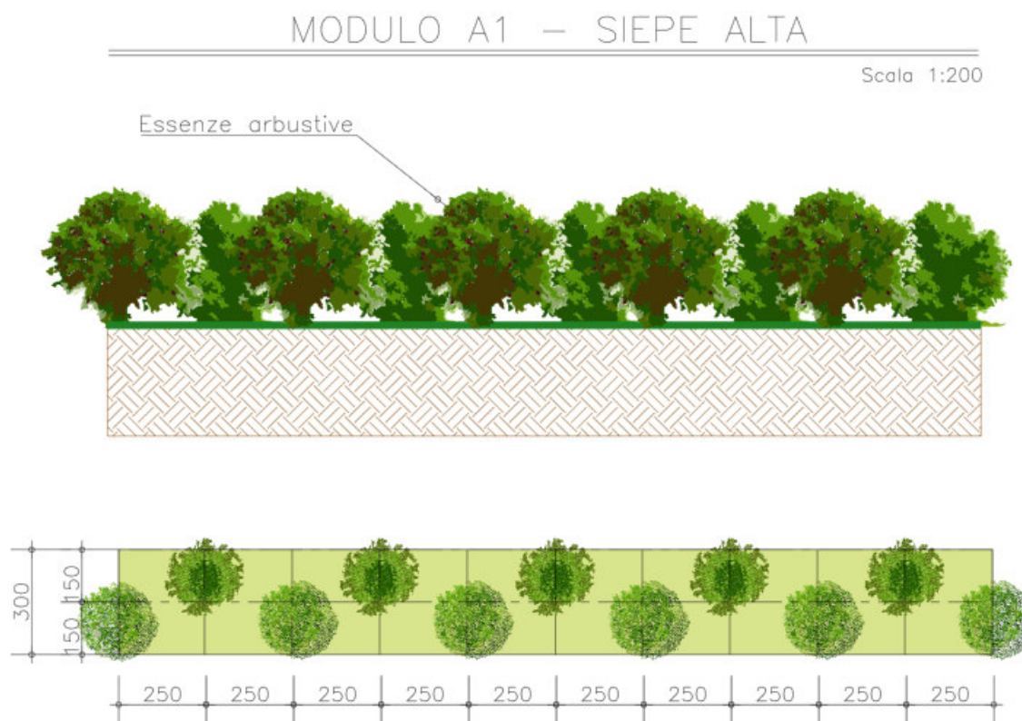
Figura 4-2 – MODULO A1 – Siepe alta: sesto d'impianto e sezione tipologica
