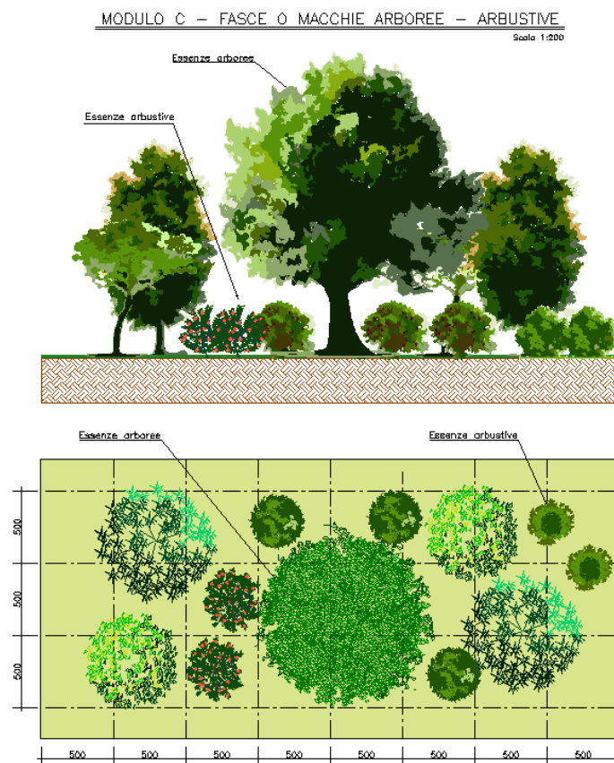
Figura 4-4 – MODULO C – Fasce o macchie arboreo-arbustive: sesto d'impianto e sezione tipologica
