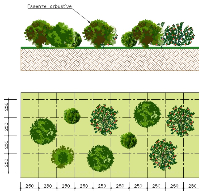
Figura 4-3 – MODULO B – Fasce o macchie arbustive: sesto d'impianto e sezione tipologica
