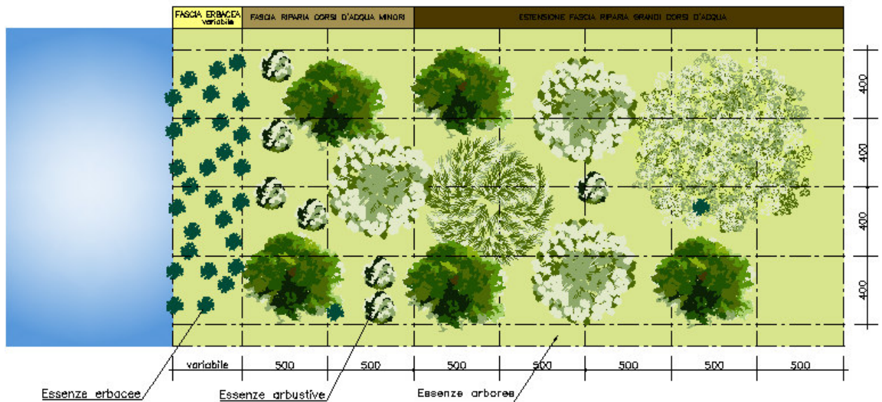
Figura 4-5 – MODULO D – Sistemazione vegetazione spondale: sesto d'impianto e sezione tipologica
