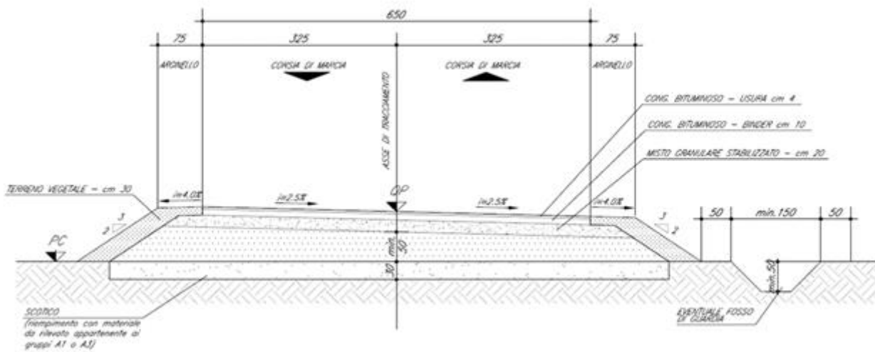
Estratto planimetria IN0R11EE2PZGA1707001A – Sezione stradale
