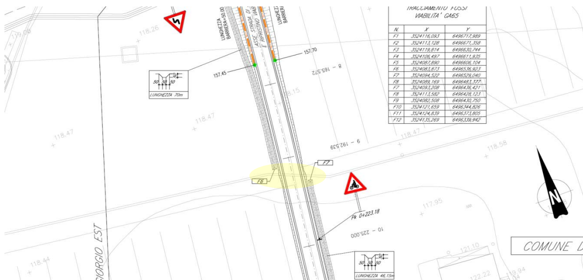
Estratto planimetria INOR11EE2PZGA1707001A – Canale irriguo interrato già passante sotto la strada sterrata esistente Via Calvisana
