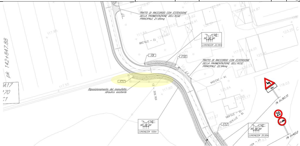
Estratto planimetria IN0R11EE2PZGA1707001A – Riposizionamento del manufatto idraulico esistente del canale irriguo interrato passante lungo la traversa della strada sterrata esistente Via Calvisana
