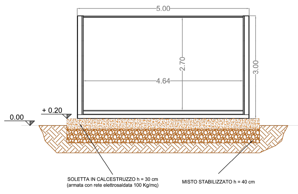
SEZIONE TRASVERSALE
