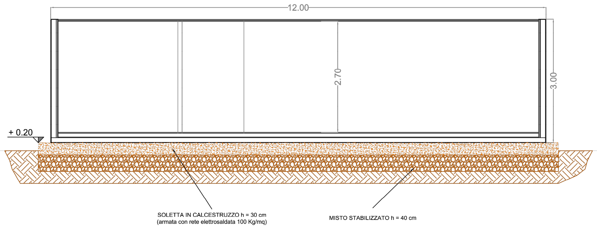
SEAZIONE LONGITUDINALE
