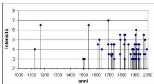
Fig. 3 - Storia sismica di Enna, rappresenta le intensità calcolate al sito mediante una legge di attenuazione cubica dalle intensità epicentrali tratte dal catalogo parametrico dei terremoti italiani (GRUPPO DI LAVORO CPTI, 1999).
