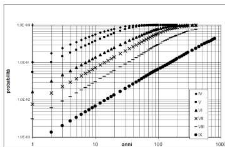
Fig. 4 – Probabilità di occorrenza calcolata con il metodo di MAGRI et alii (1994).
