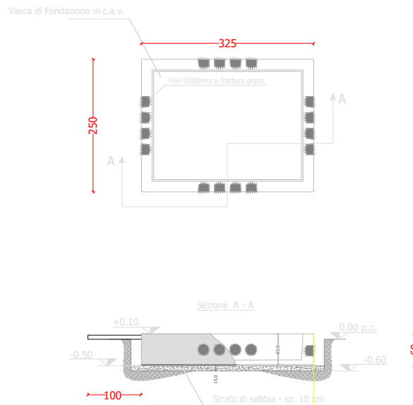
PARTICOLARE VASCA
