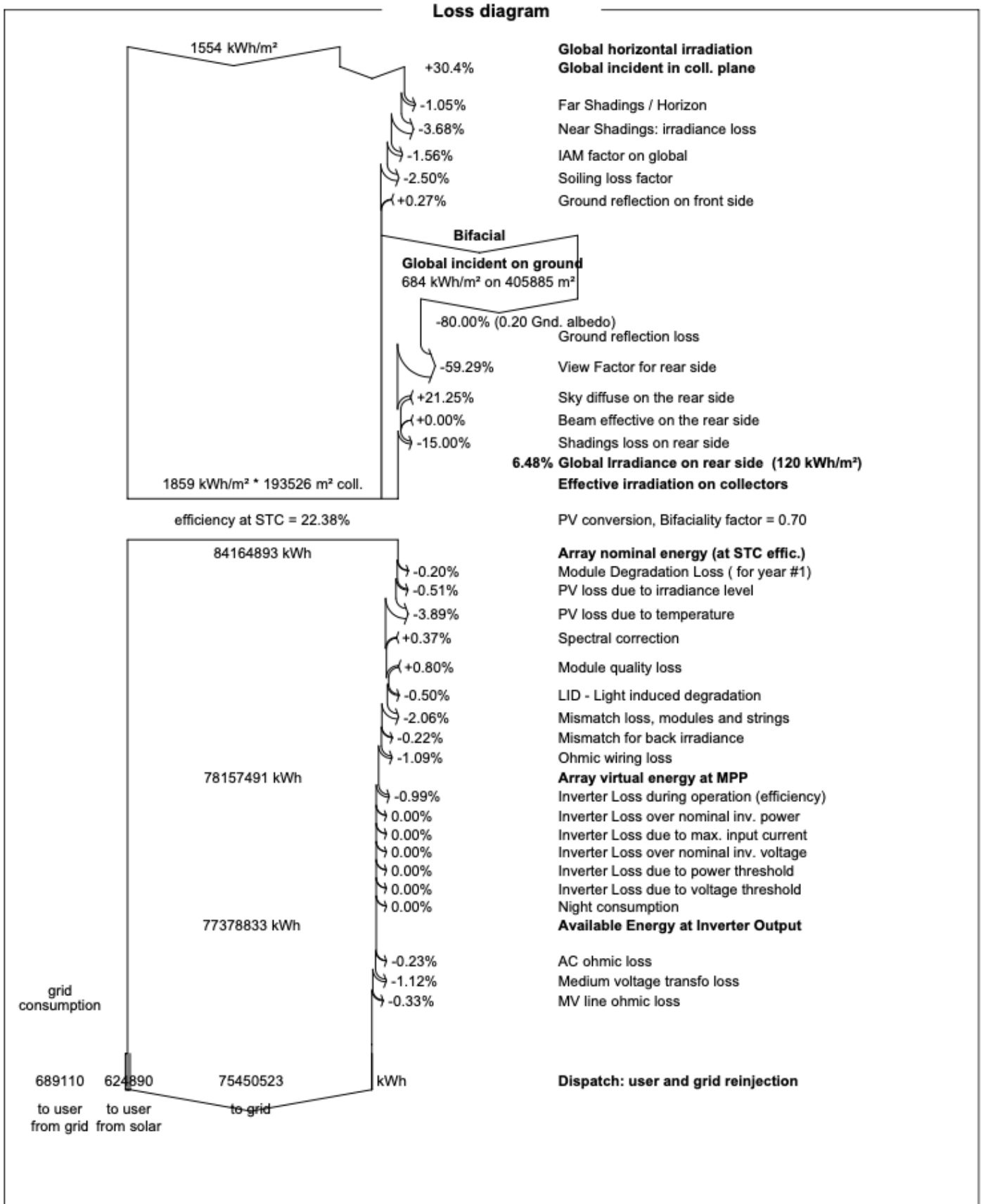
Fig. 3: Perdite
