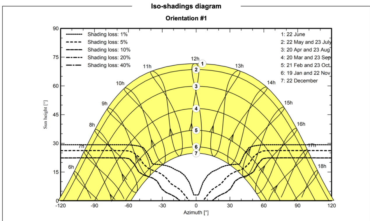
Fig. 2: Diagramma solare
