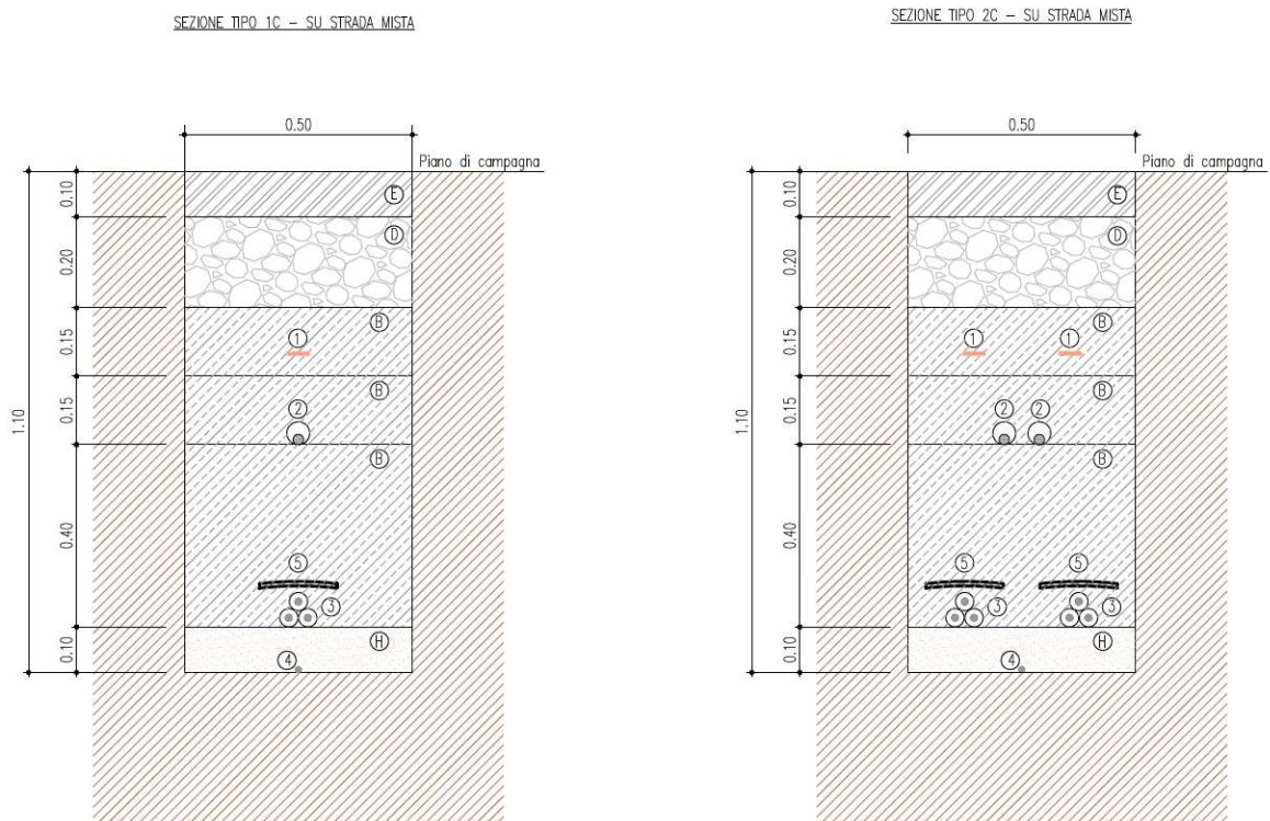
Figura 3: Tipologico cavidotto sez.: 1C e 2C
