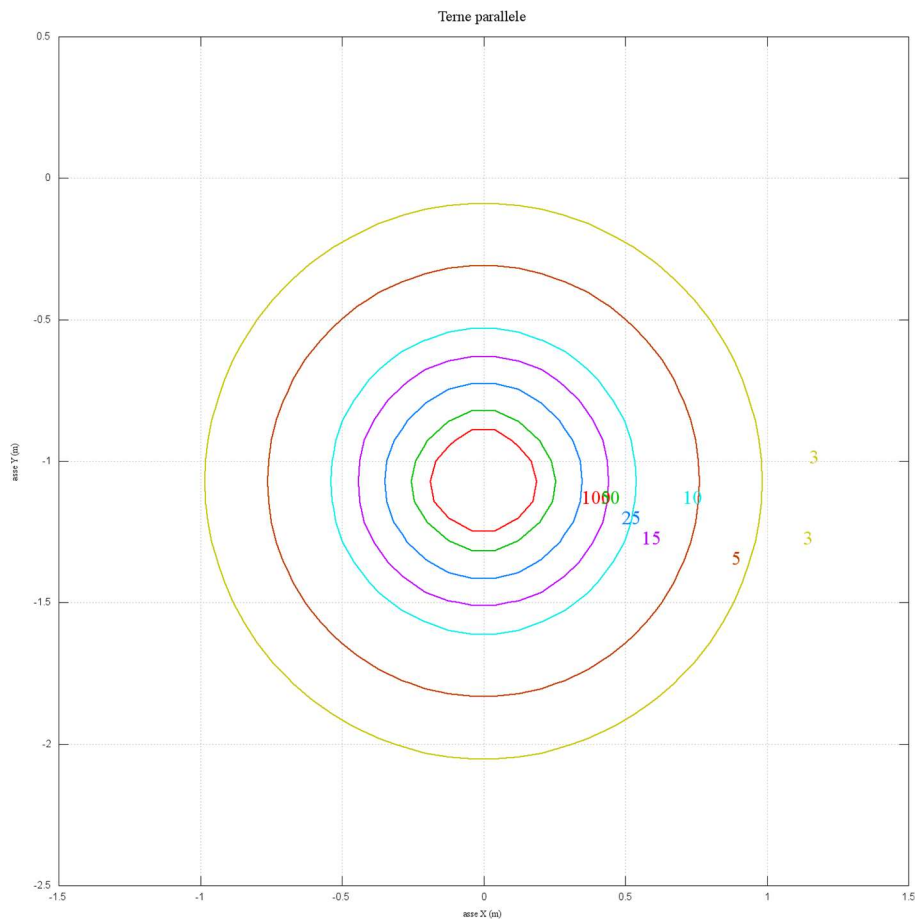
Figura 5: DPA tratto MA01 – MA05 (valori calcolati con l'ausilio del software Magic)
