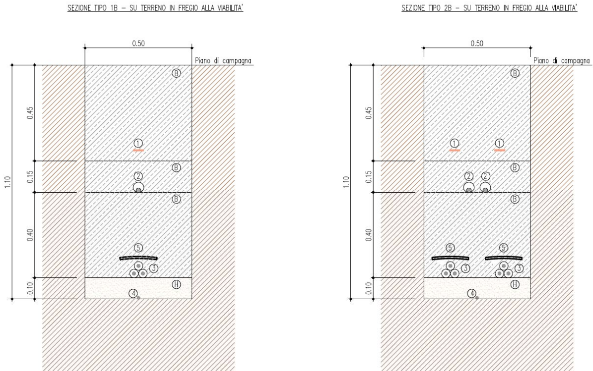
Figura 2: Tipologico cavidotto sez.: 1B e 2B
