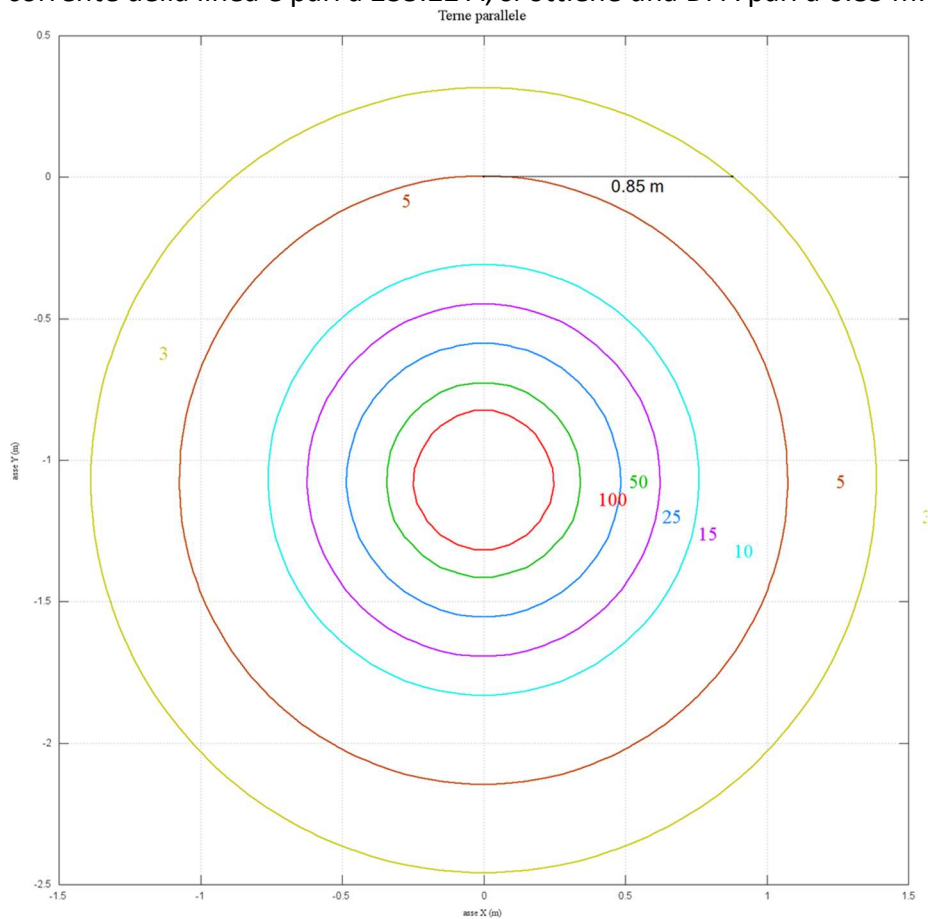
Figura 6: DPA tratto MA05 - MA02 (valori calcolati con l'ausilio del software Magic)
