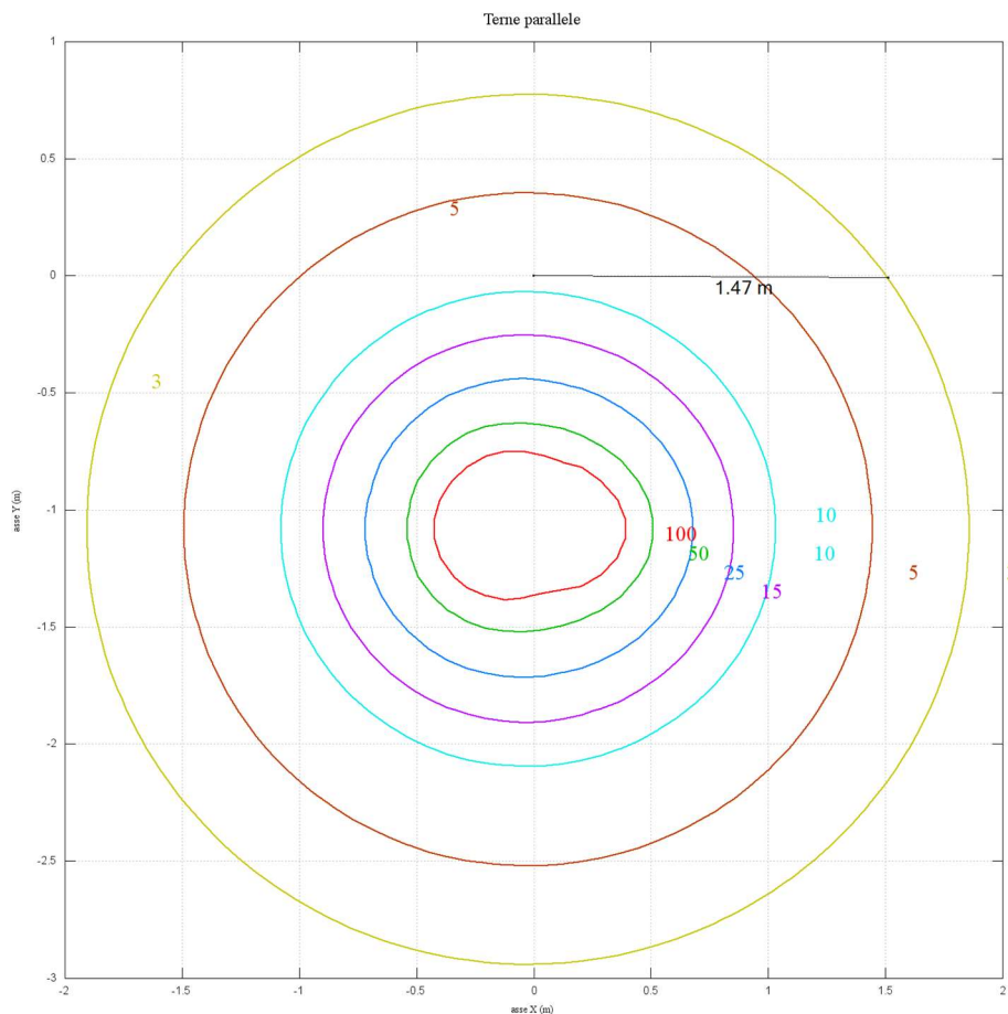
Figura 9: DPA tratto MA04-cavidotto esterno (valori calcolati con l'ausilio del software Magic)
