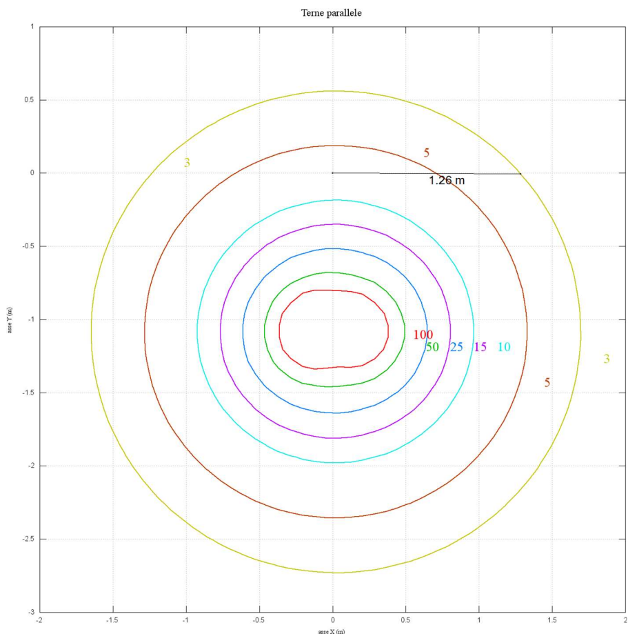
Figura 8: DPA tratto MA03 – MA04 (valori calcolati con l'ausilio del software Magic)
