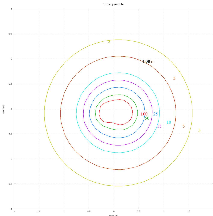
Figura 7: DPA tratto MA02-MA03 (valori calcolati con l'ausilio del software Magic)
