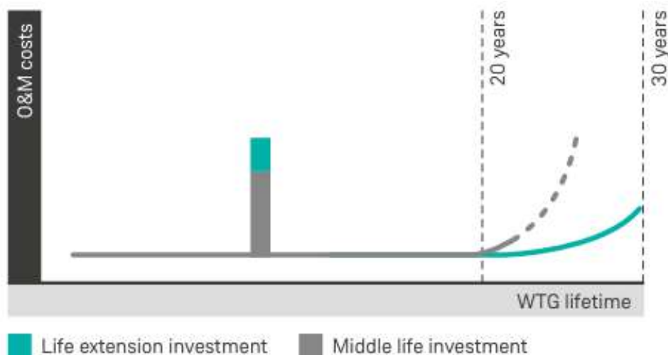
Figura 3: Incremento della vita utile degli impianti
