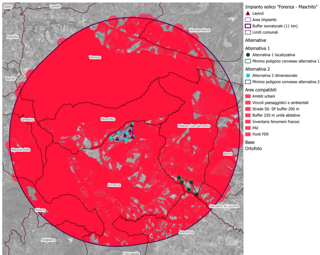
Figura 4. Localizzazione del layout di progetto e dei layout alternativi su base ortofoto
