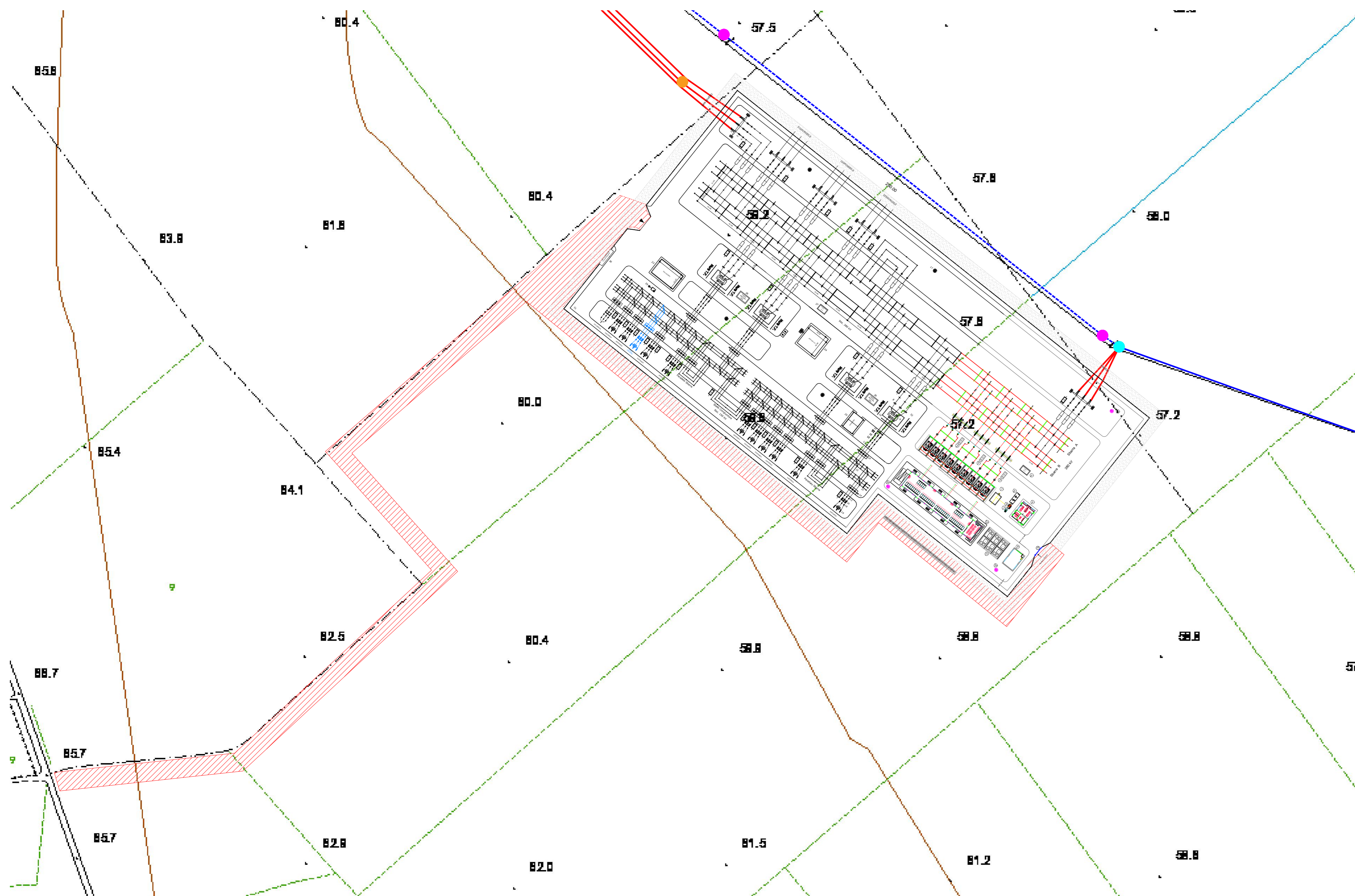
PLANIMETRIA DI INQUADRAMENTO SU CARTOGRAFIA (CTR)
