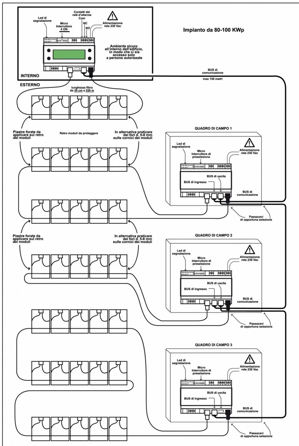
Figura 11 - Sistema di antifurto dei moduli FV
