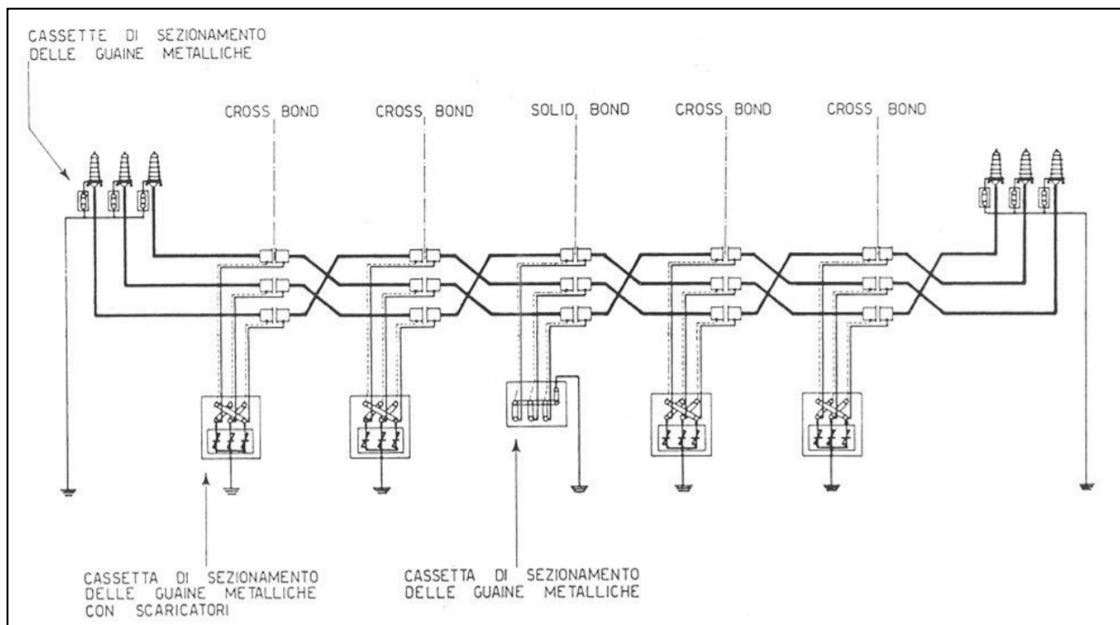
Figura 14 – Tipico di collegamento "cross bonding" per un cavo in AT
