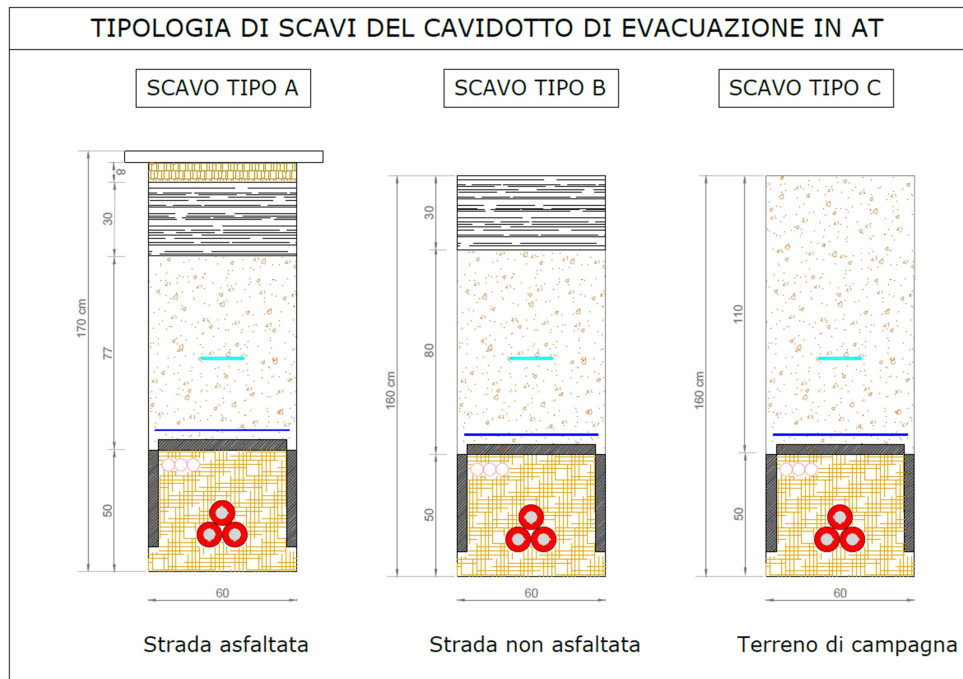
Figura 15 – Sezioni tipiche di scavo e di posa per il cavo in AT a 132 kV
