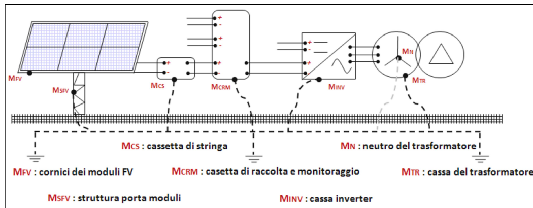
Figura 10 – Schema della messa a terra a monte del trasformatore
