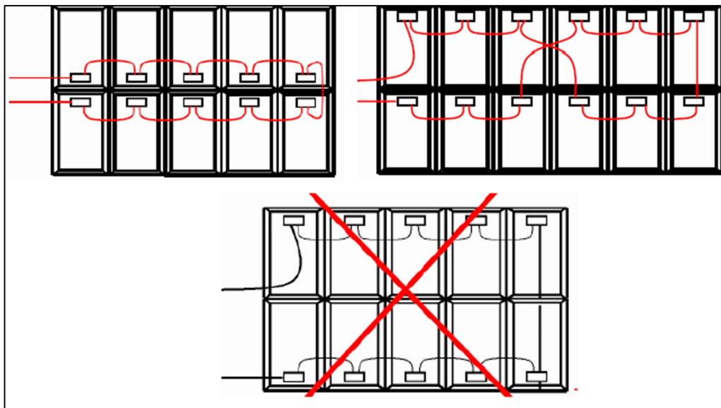
Figura 12 – Tipico di collegamento tra i moduli contro le fulminazioni
