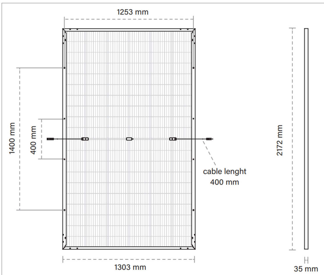
Figura 2 - Tipologia di modulo utilizzato nel progetto P=680 \text{ Wp}
