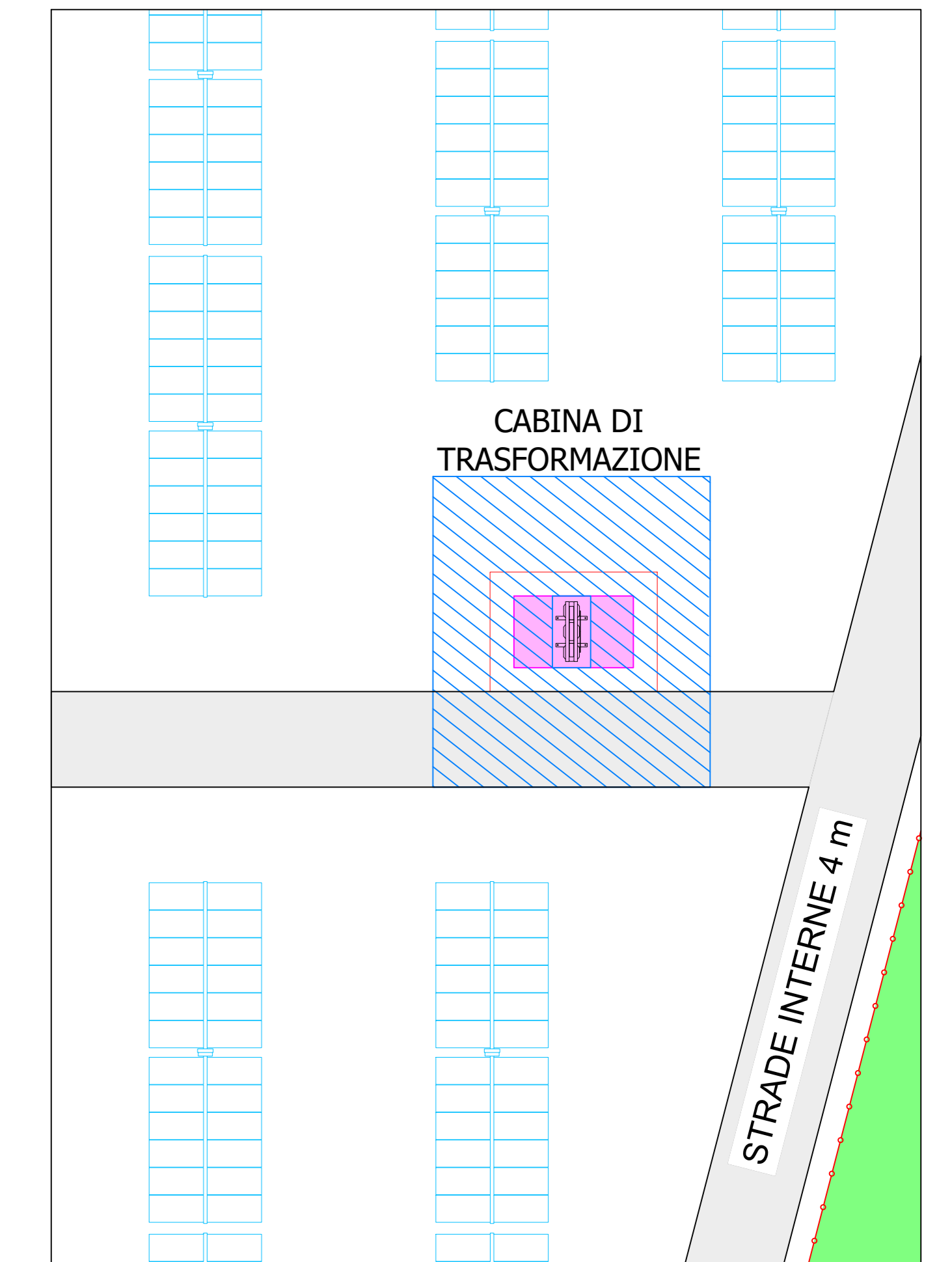
DPA CABINA TRASF. Scala 1:200
