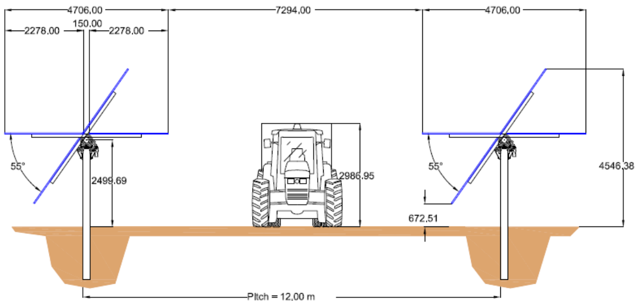
Figura 3-4. Schema dell'ingombro di una trattrice all'interno dell'impianto.
