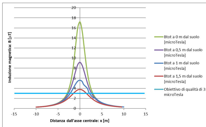
Figura 3: Andamento del campo magnetico generato composto da cinque terne da 630 mm 2
