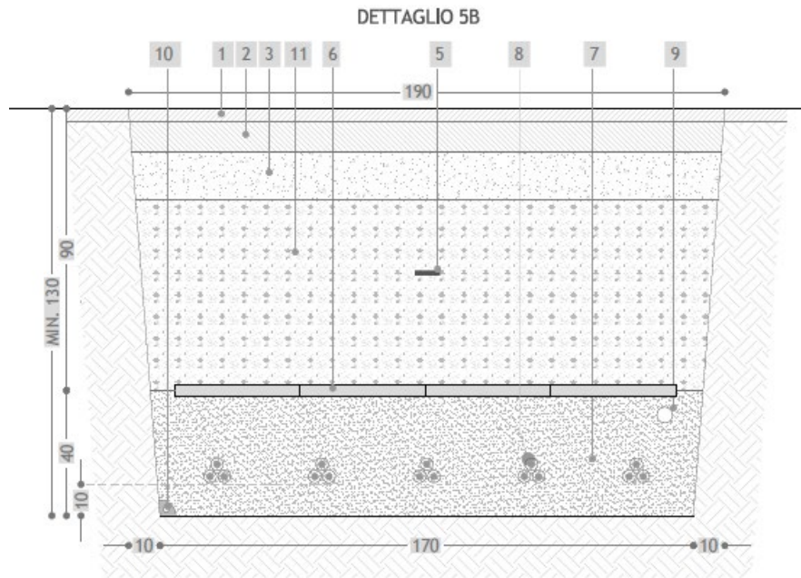
Figura 2: Sezione tipo cavidotto composto da cinque terne da 630 mm 2
