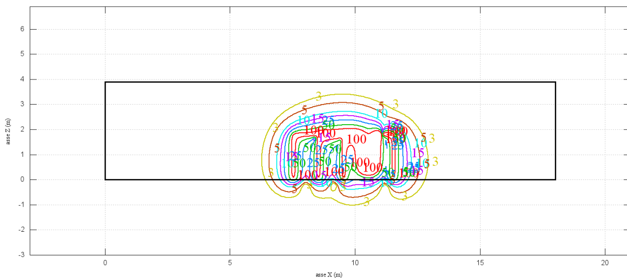
Cabina - calcolo su piano xz - quote Y=2,69 m
