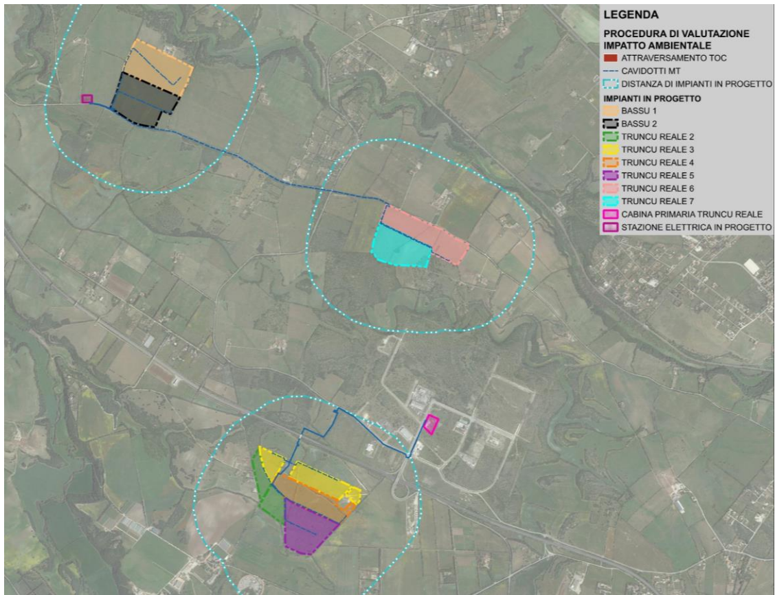
Figura 1 - Suddivisione impianti in progetto
