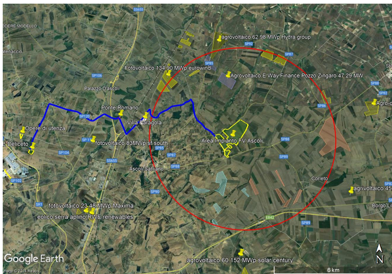
Fig. 4.14. Area di intervento (gialla), linea NT interrata e buffer 10 km (rosso), per la verifica degli impianti che ricadono interamente o parzialmente nell'area buffer
