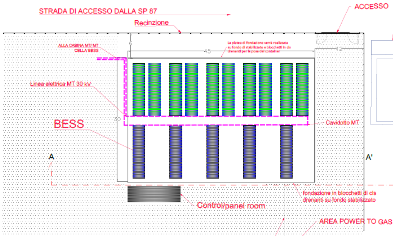
Fig. 3.21 – Layout BESS
