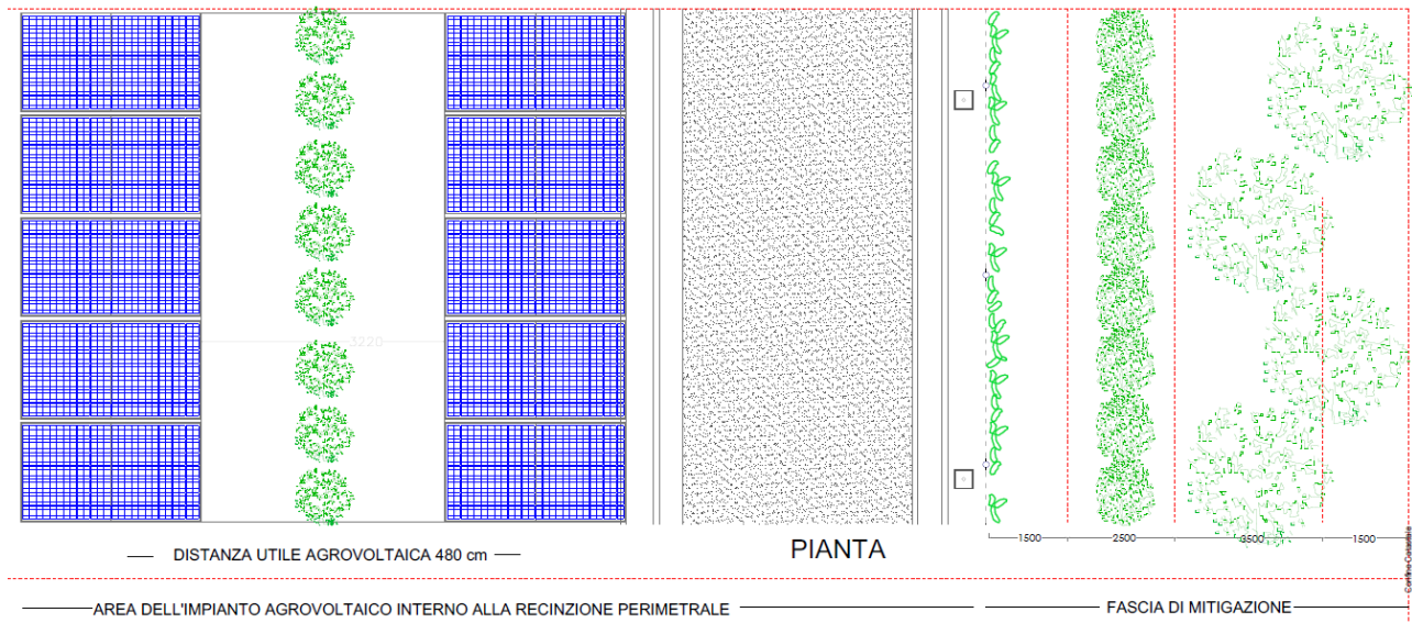
Fig. 3.17 – Pianta del modulo Agrovoltaico tipico
