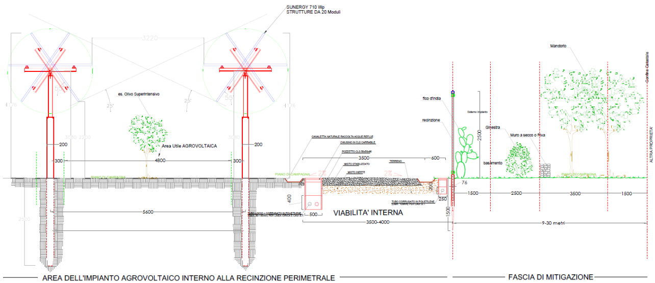
Fig. 3.16 – Sezione del modulo Agrovoltaico tipico
