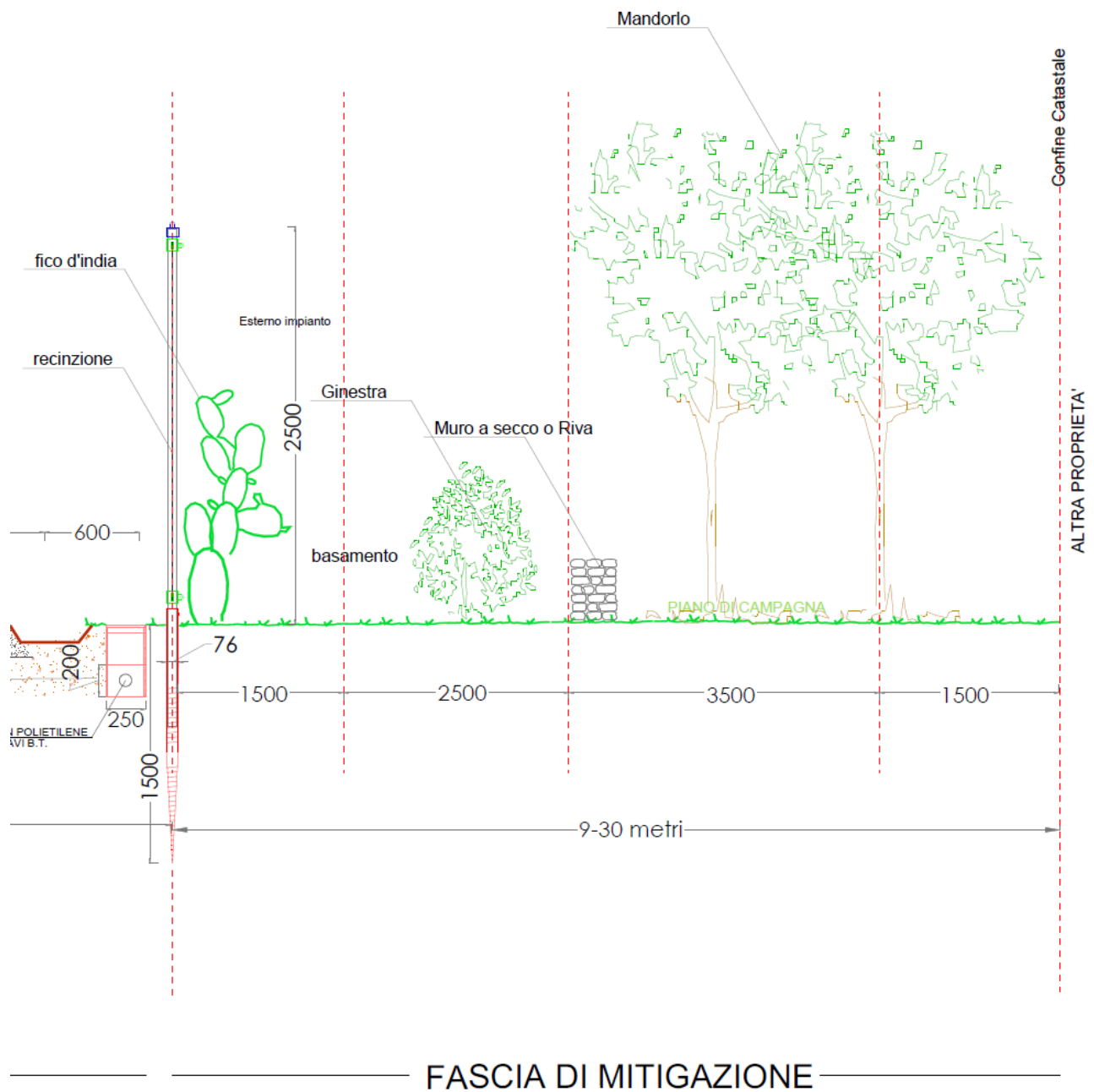
Fig 3.19 – Sezione della Fascia di Mitigazione tra la recinzione e il confine catastale o strada (min 9, max 30 m)
