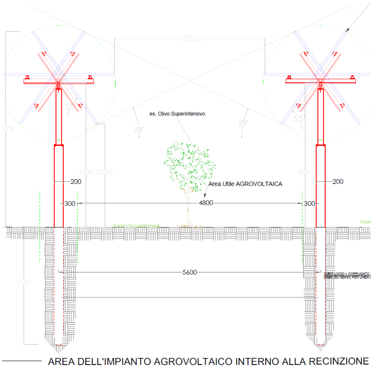
Fig 3.18 – Sezione dell'area agricola interposta tra i filari FV
