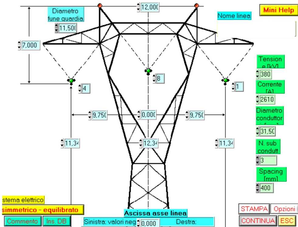
Fig. disposizione attacco dei conduttori
