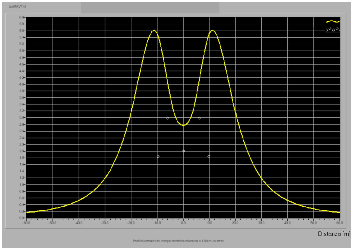
Fig. Profilo Laterale CAMPO ELETTRICO
