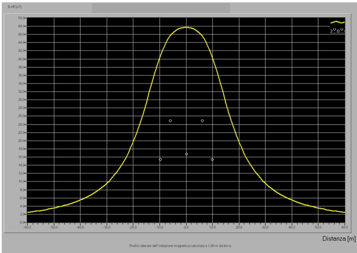
Fig. Profilo Laterale INDUZIONE MAGNETICA
