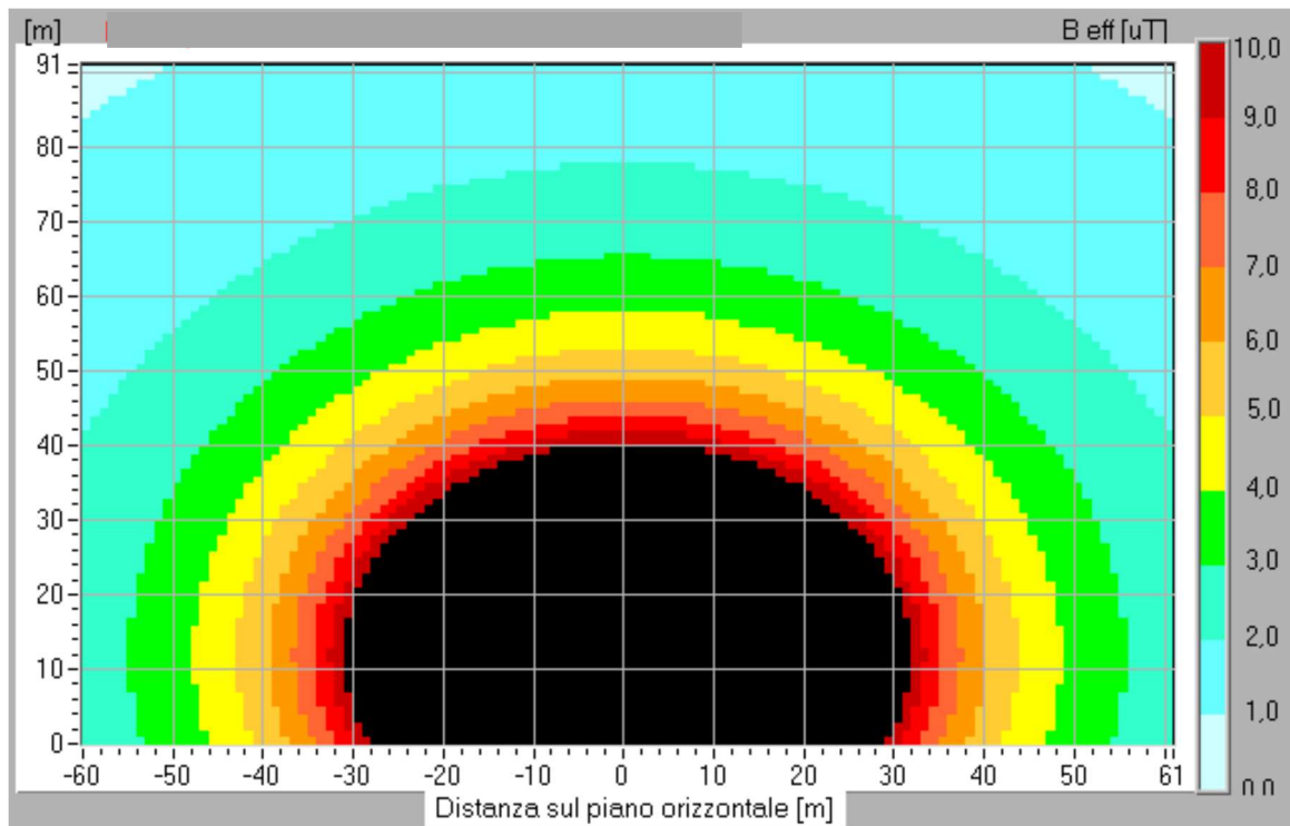
Fig. Mappa Verticale INDUZIONE MAGNETICA
