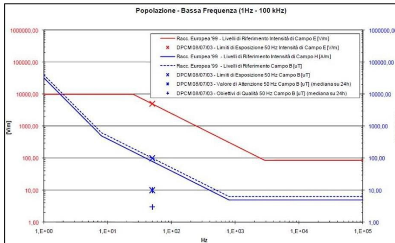
Figura 3.9. – Livelli esposizione Bassa Frequenza (1Hz – 100 kHz).
