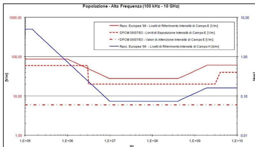
Figura 3.10. – Livelli esposizione Alta Frequenza (100kHz – 10 GHz).
