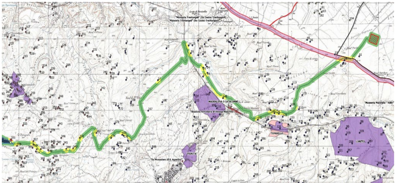
Figura 3.17 - Cavidotto: siti classificati a RISCHIO ALTO (in rosso) e RISCHIO MEDIO (in giallo)
