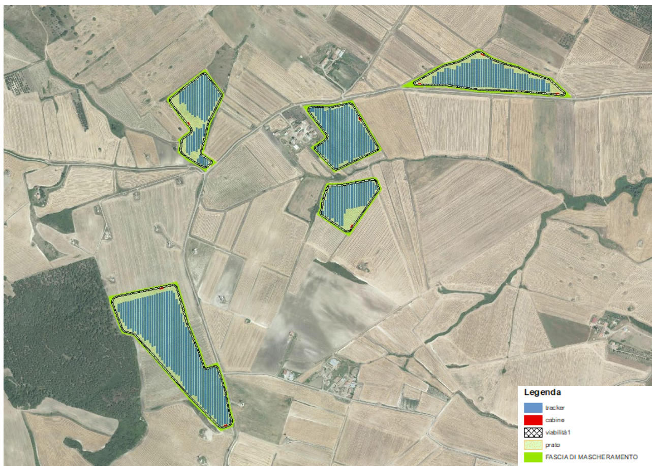
Figura 3.3 - Stralcio impianto su base Ortofoto
