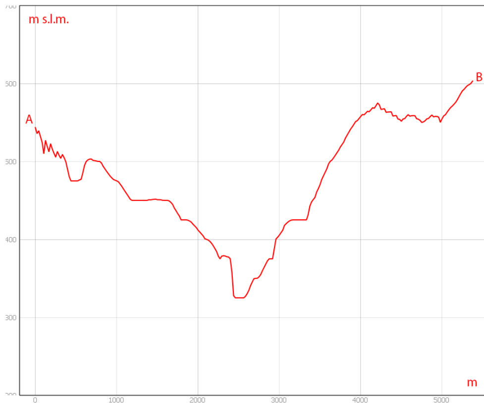
Sezione morfologica del terreno- Punto di presa n°16
