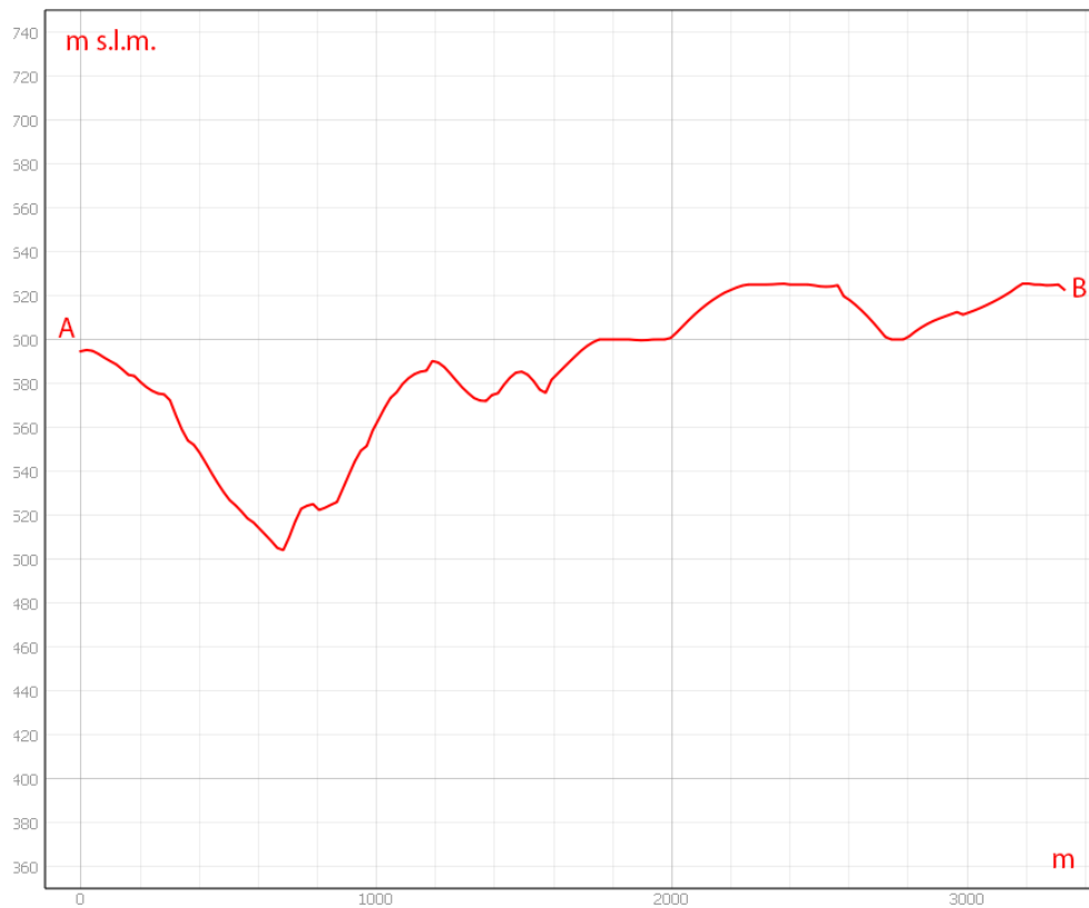
Sezione morfologica del terreno- Punto di presa n°17
