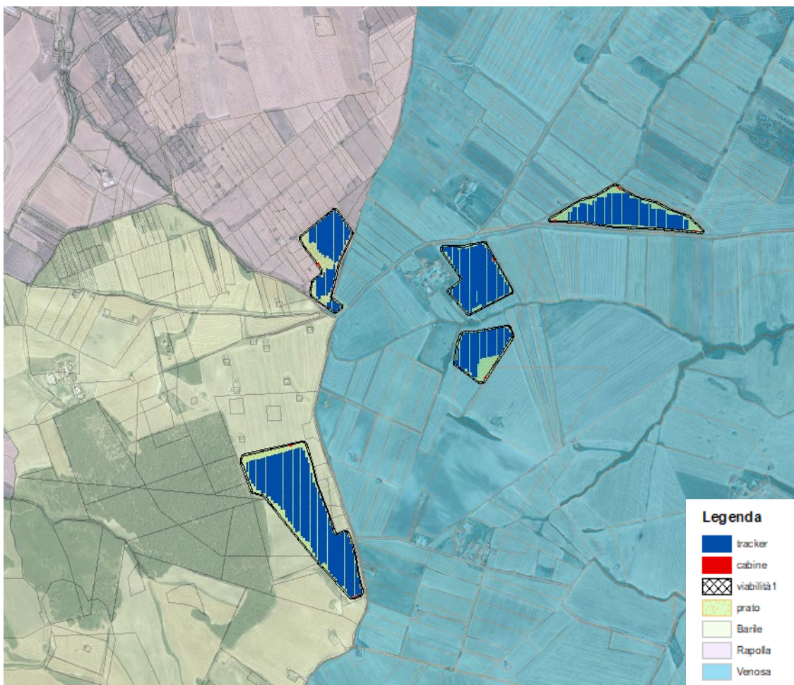
Figure 3.6 Progetto dell'impianto FV su ortofoto e catastale
