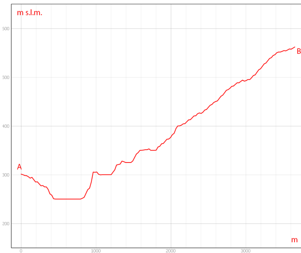
Sezione morfologica del terreno- Punto di presa n°4
