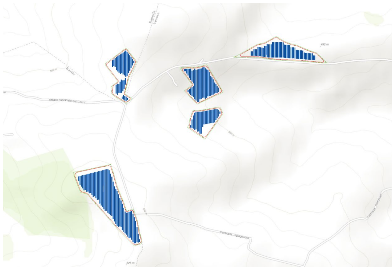
Figura 3.10 Cavidotto e viabilità esistente - dettaglio
