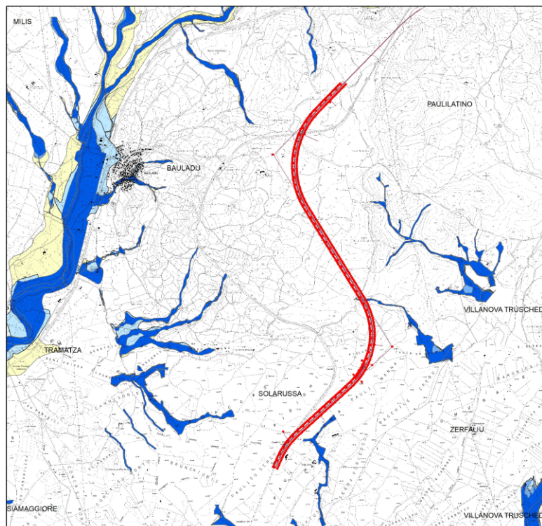
Figura 15 - Stralcio della carta del pericolo idraulico lungo il tracciato di progetto.
