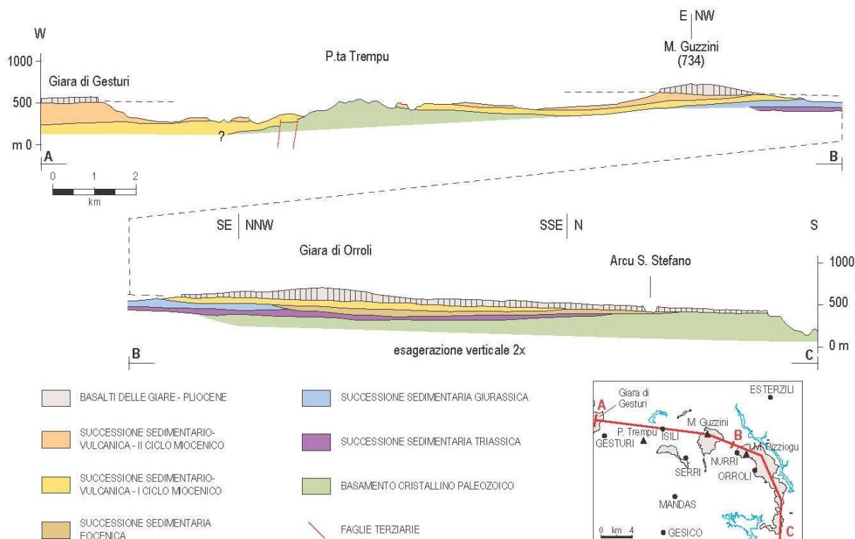
Figura 10 – Sezione geologica schematica attraverso le giare basaltiche dell'area di Mandas, che evidenzia la presenza della estesa superficie di spianamento al di sotto delle colate plio-pleistoceniche (da Funedda et al. 2012).
