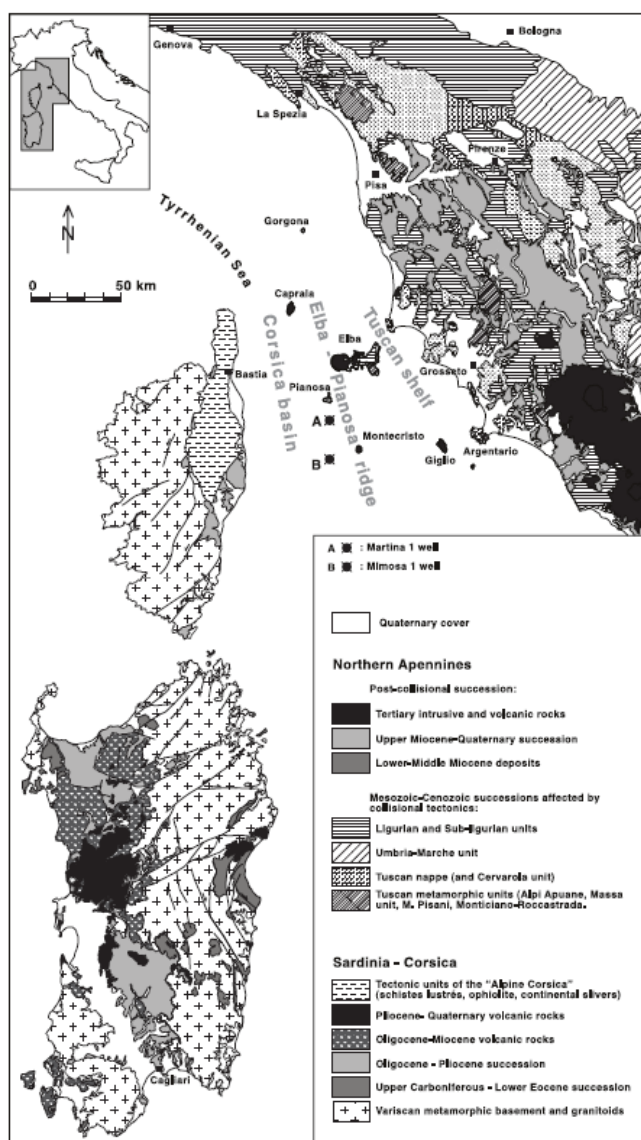
Figura 4 – Schema stratigrafico-strutturale dell'Appennino settentrionale, del Blocco Sardo-Corso e del Bacino Tirrenico settentrionale (da Carmignani et al. 2004).
