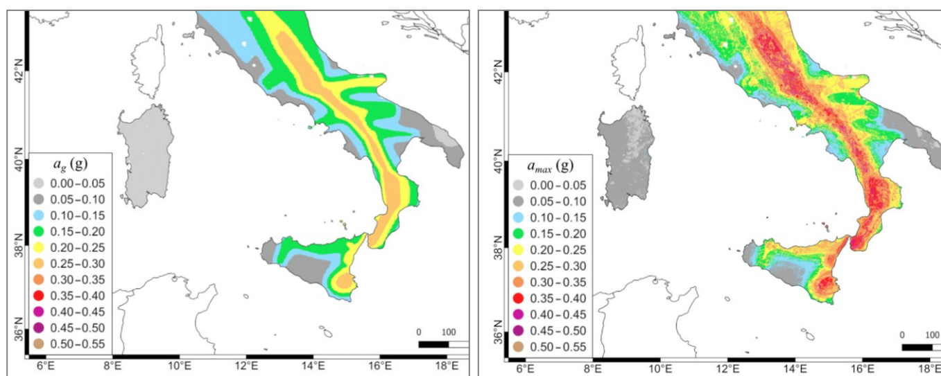
Figura 17 – Mappa della pericolosità associata all'accelerazione di picco orizzontale su substrato roccioso e topografia pianeggiante corrispondente a un periodo di ritorno di 475 anni ( a_g hazard map) - Mappa della pericolosità associata all'accelerazione di picco orizzontale in superficie corrispondente a un periodo di ritorno di 475 anni ( a_{max} hazard map).
