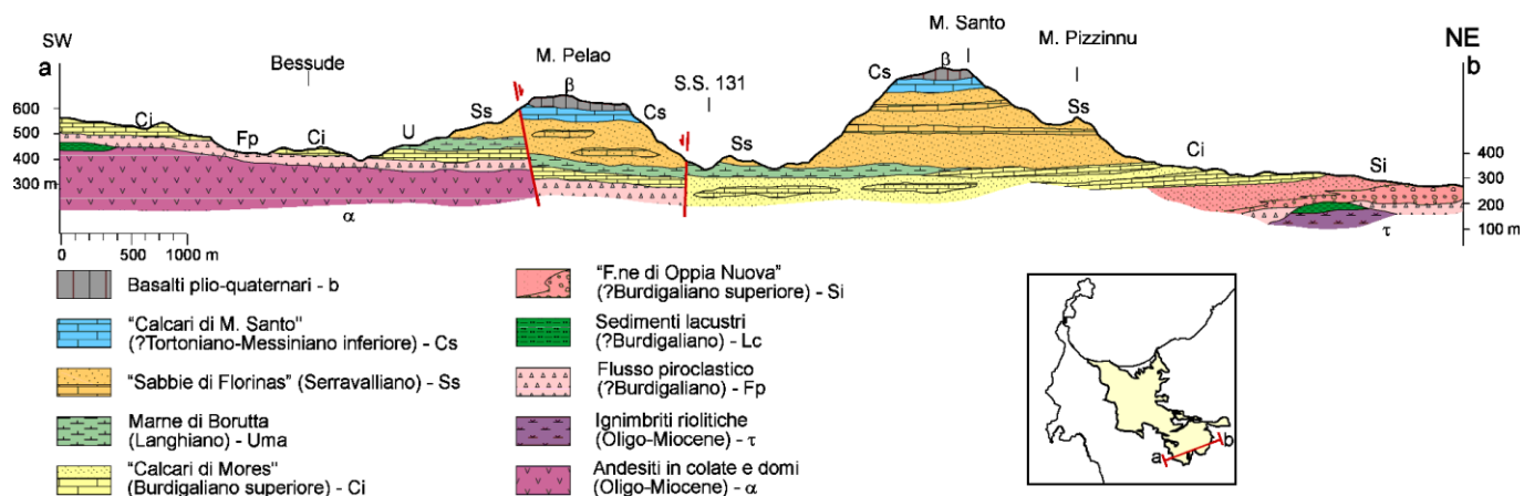
Figura 9 – Sezione geologica della successione sedimentaria miocenica del Logudoro (da Funedda et al. 2000).
