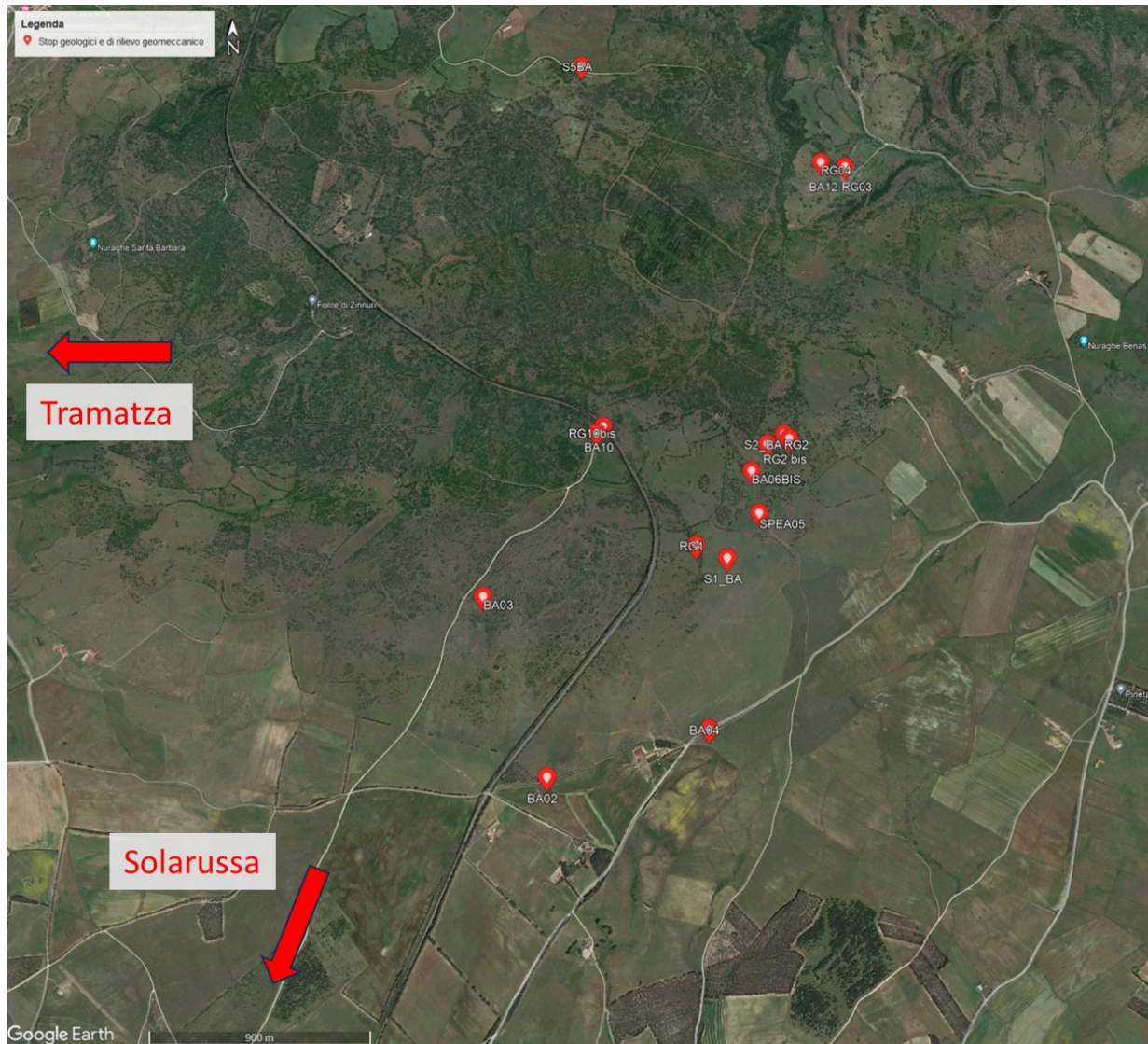
Figura 3 – Stop geologici e di rilievo nell'area di studio
