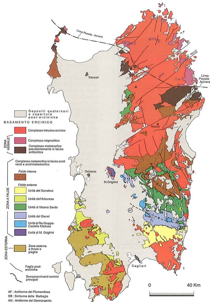
Figura 11 - Schema dei principali elementi strutturali del basamento ercinico sardo (da Carmignani et al. 2001)
