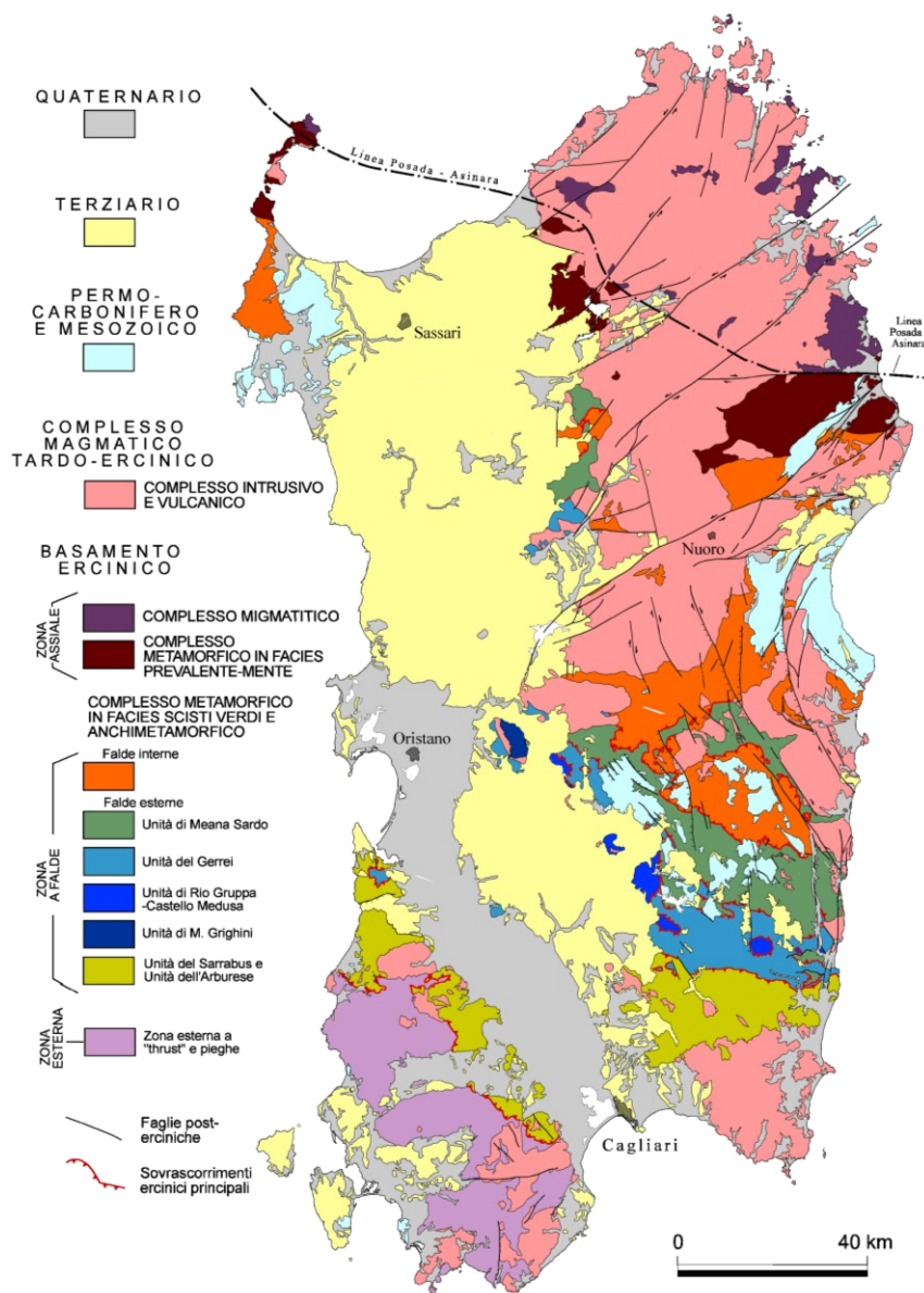
Figura 6 – Schema stratigrafico-strutturale della Sardegna, con relativa legenda (da Carmignani et al. 2001).
