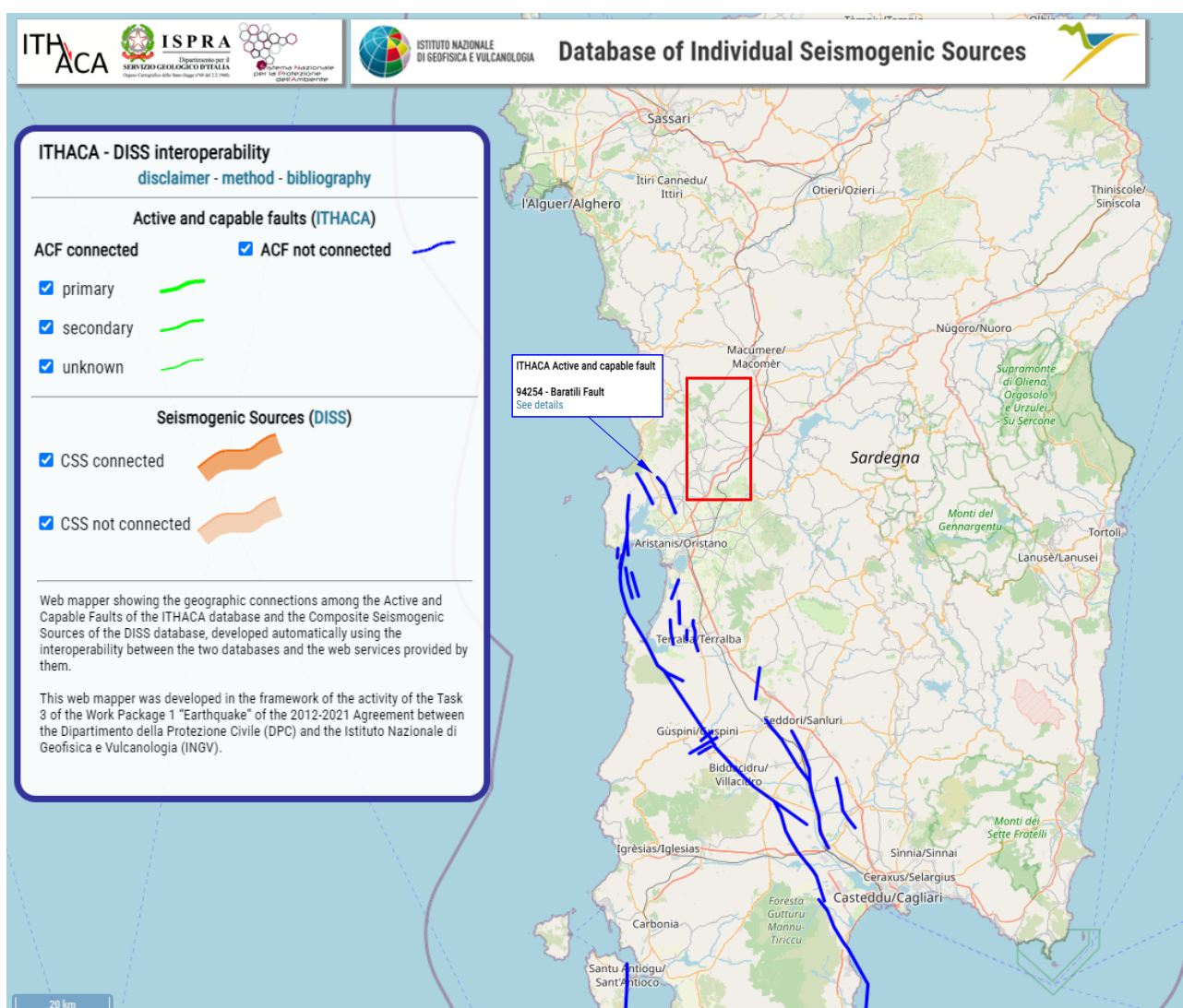
Figura 12 - Localizzazione delle potenziali sorgenti attive e capaci nell'area di studio (da ITHACA - DISS).
