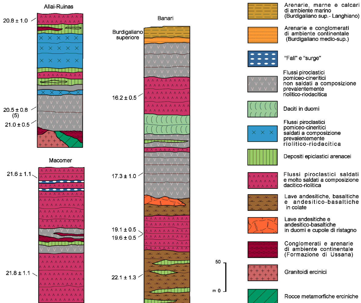
Figura 8 – Colonne stratigrafiche schematiche delle successioni vulcaniche oligo-mioceniche (da Lecca et al. 1997).
