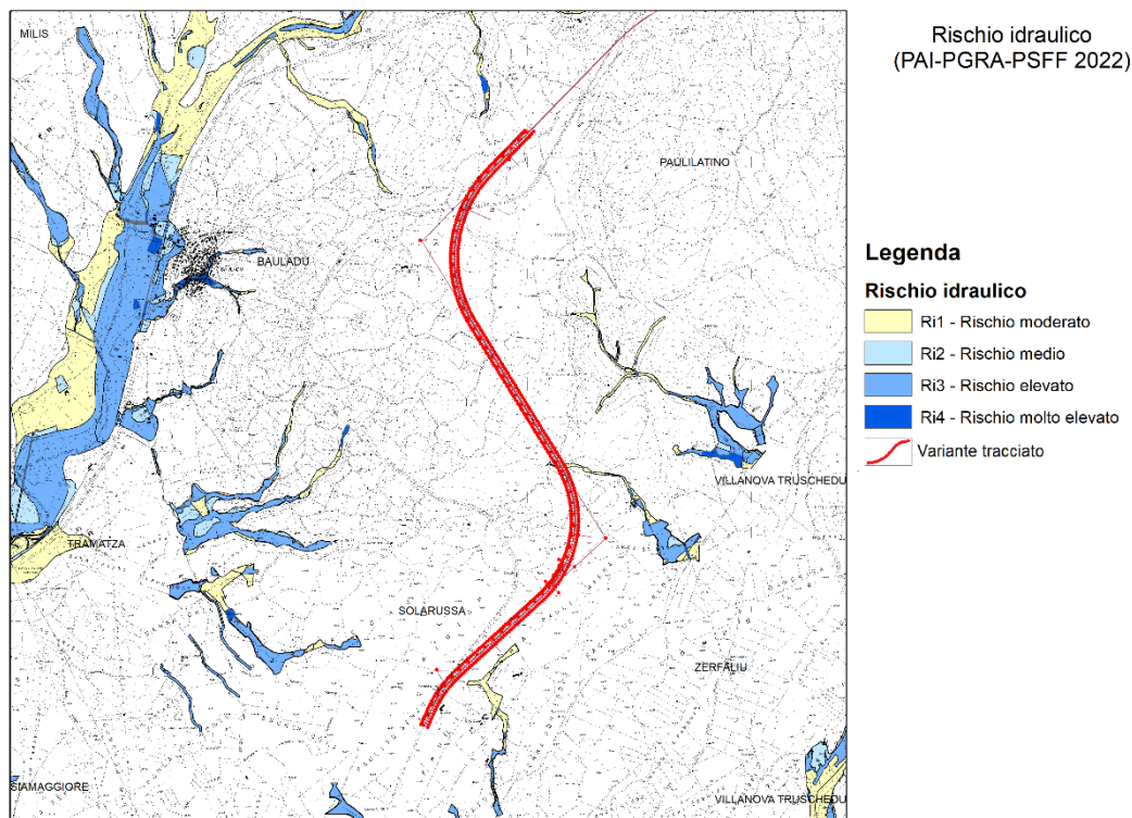
Figura 16 - Stralcio della carta del rischio idraulico lungo il tracciato di progetto.
