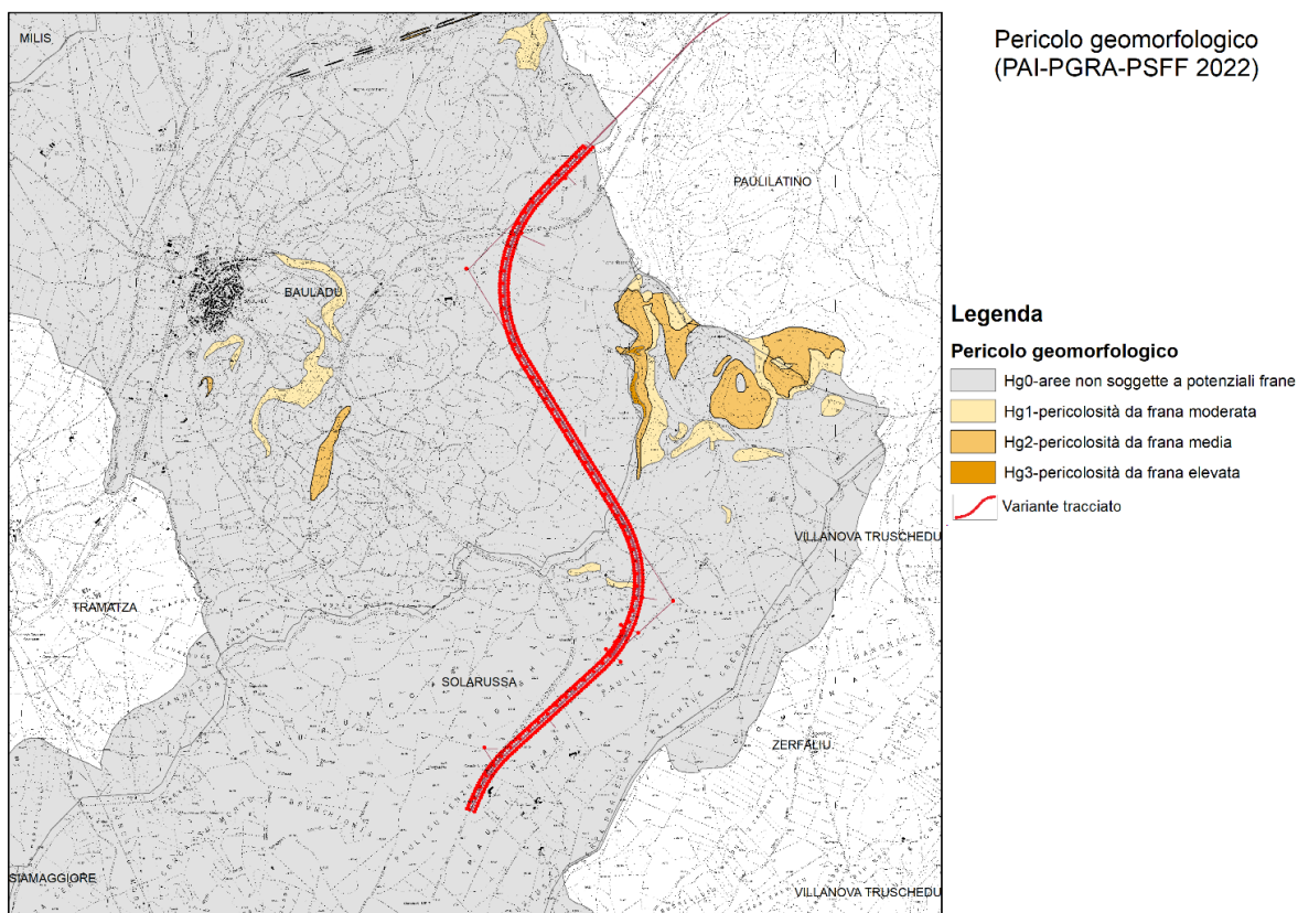
Figura 13 - Stralcio della carta della pericolosità geomorfologica lungo il tracciato di progetto.
