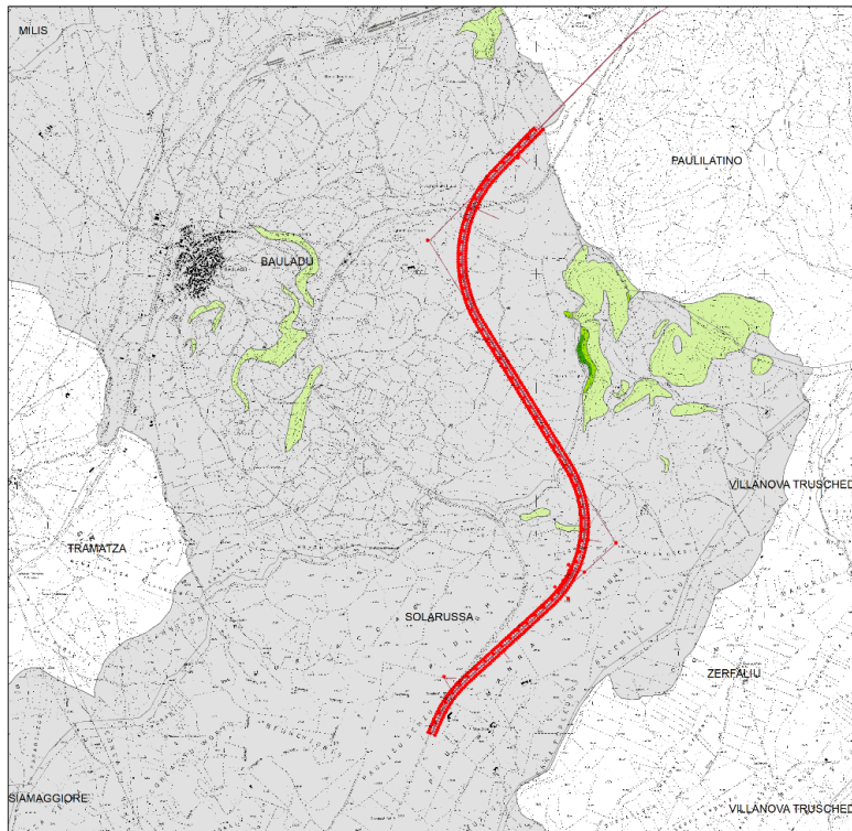
Figura 14 - Stralcio della carta del rischio geomorfologico lungo il tracciato di progetto.
