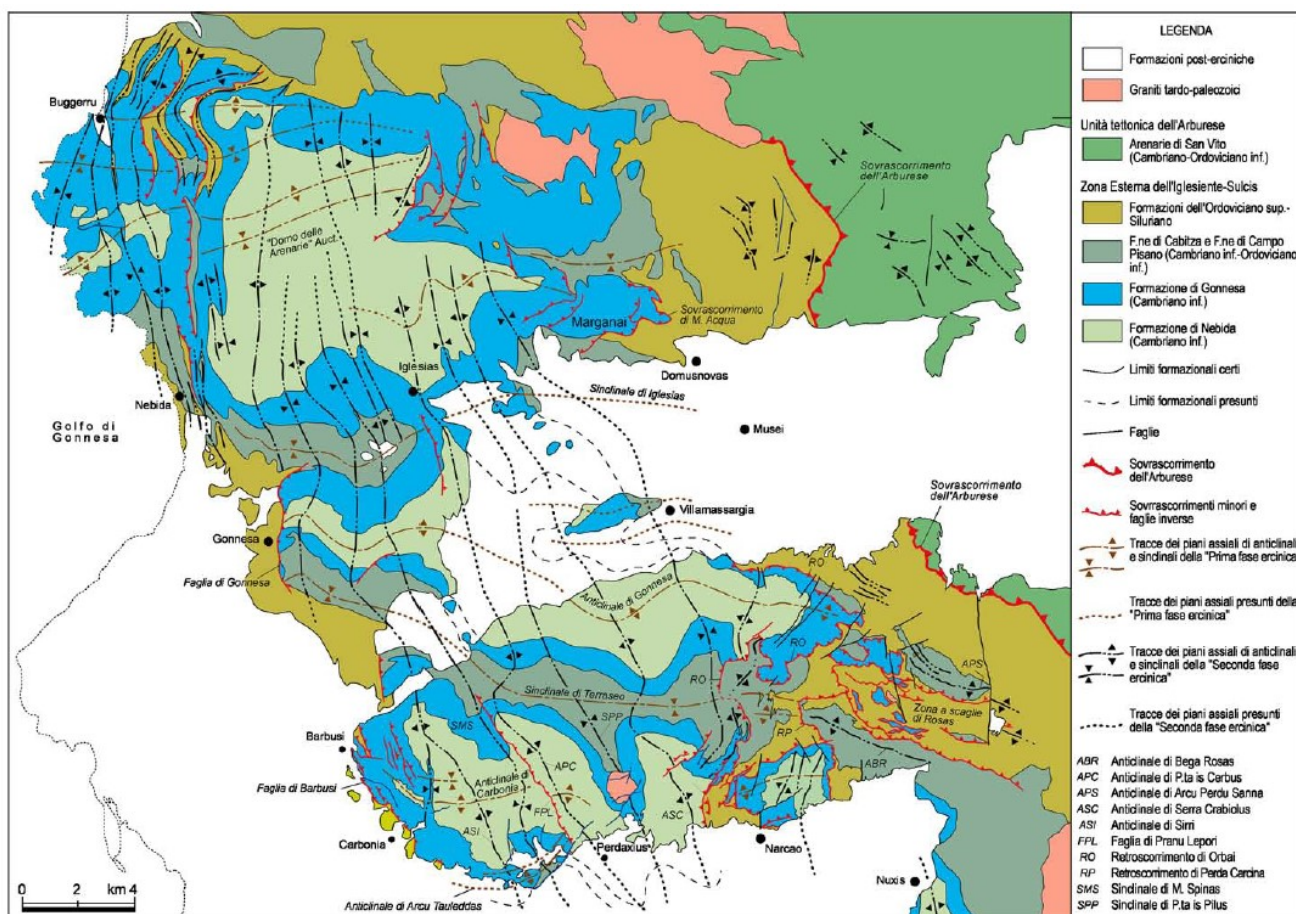
Figura 7 – Schema geologico-strutturale del basamento metamorfico del Sulcis-Iglesiente (da Carmignani et al. 1982).
