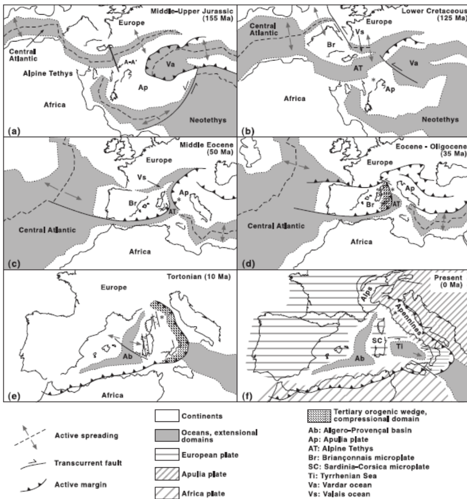
Figura 5 – Evoluzione geologica del Mediterraneo occidentale e del Blocco Sardo-Corso (da Carmignani et al. 2004).
