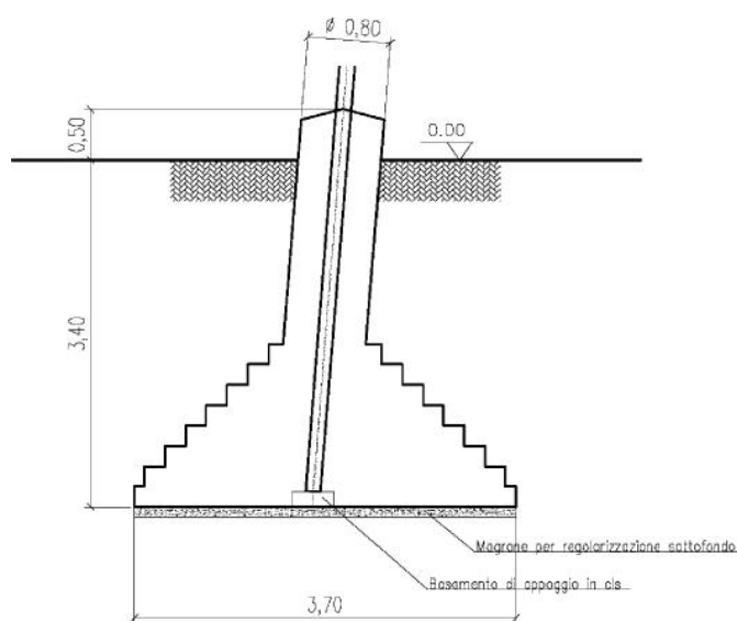
Esempio di realizzazione di una fondazione a plinto con riseghe. Nell'immagine di sinistra di può osservare un disegno di progetto mentre nell'immagine di destra la fase di casseratura della fondazione
