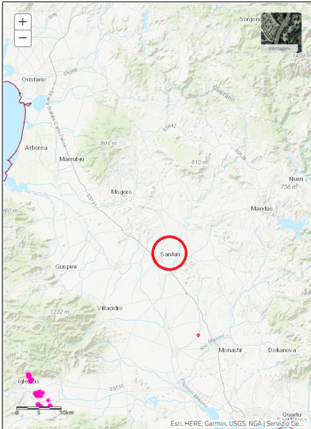
Estratto dal "Database Nazionale Sinkholes" dell'ISPRA. In viola sono evidenziate le aree interessate dal fenomeno dei sinkholes, mentre nel cerchio rosso è evidenziata l'area in progetto.
