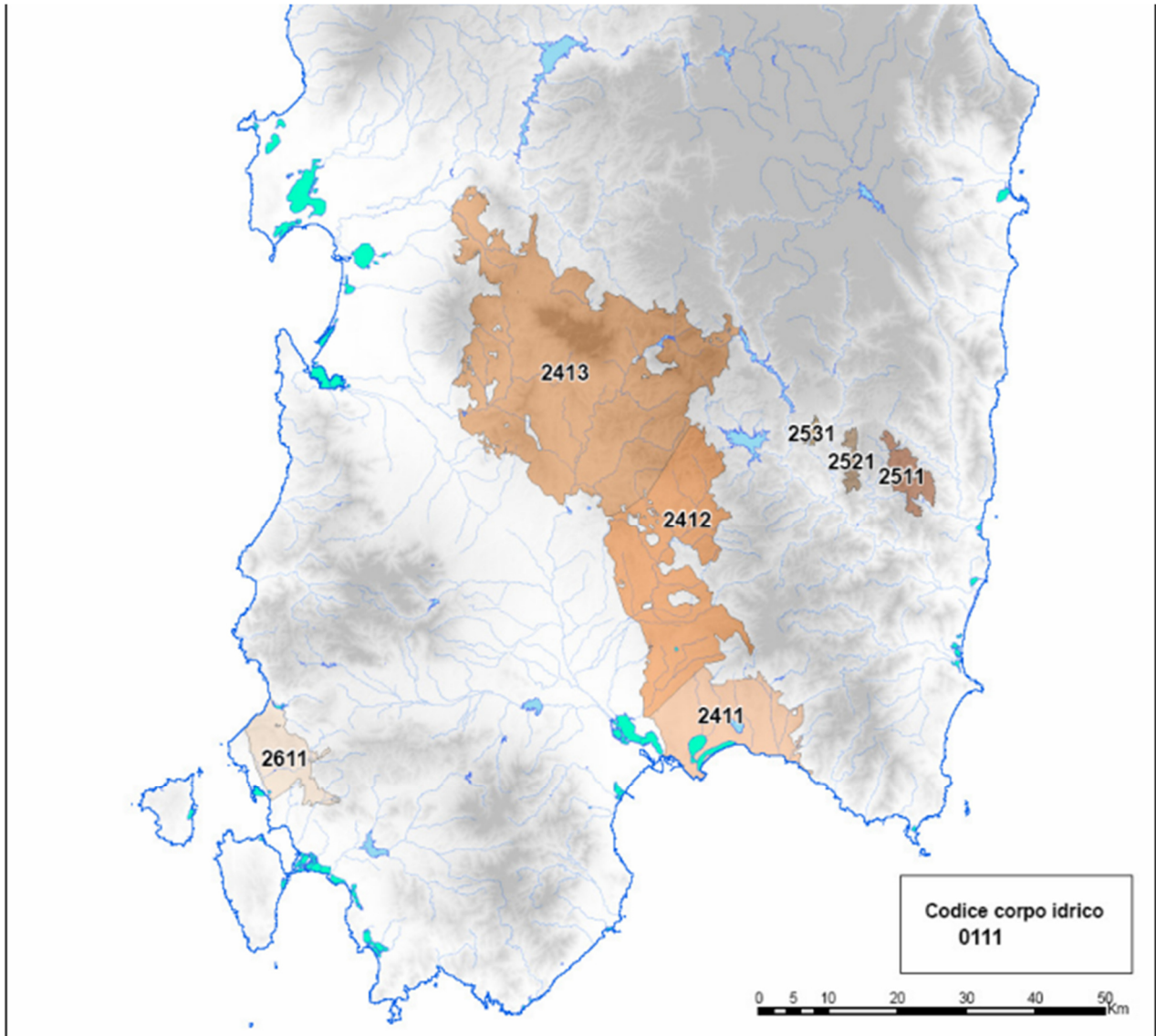
Figura 1 Corpi idrici sotterranei degli acquiferi sedimentari terziari. L'acquifero della Marmilla-Sarcidano è identificato con il numero 2413. (Img. Da CARATTERIZZAZIONE, OBIETTIVI E MONITORAGGIO DEI CORPI IDRICI SOTTERRANEI DELLA SARDEGNA).
