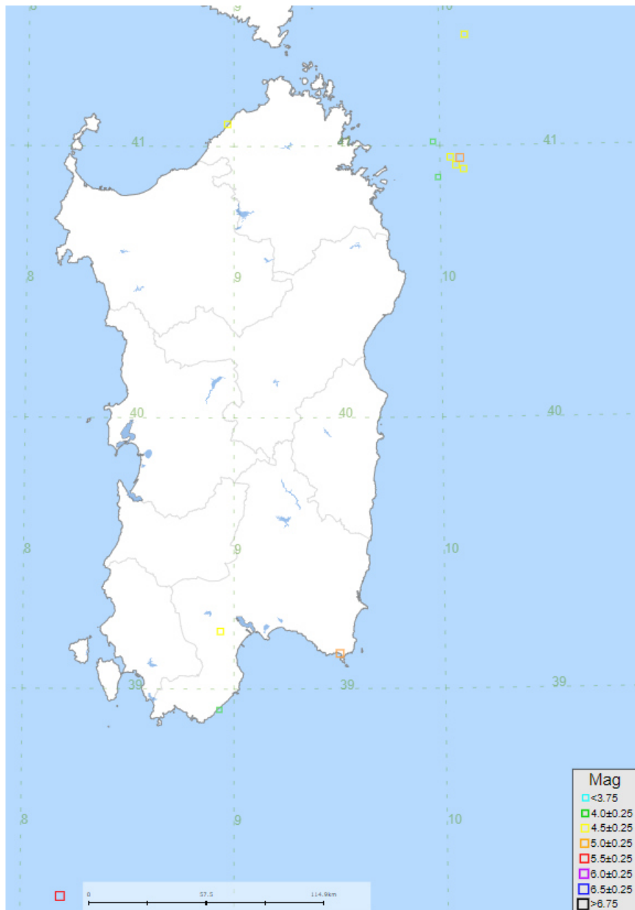
Epicentri dei maggiori sismi nell'area sarda negli ultimi 1000 anni. I dati sono stati desunti dal sito internet: https://emidius.mi.ingv.it/CPT115-DBMI15 .
