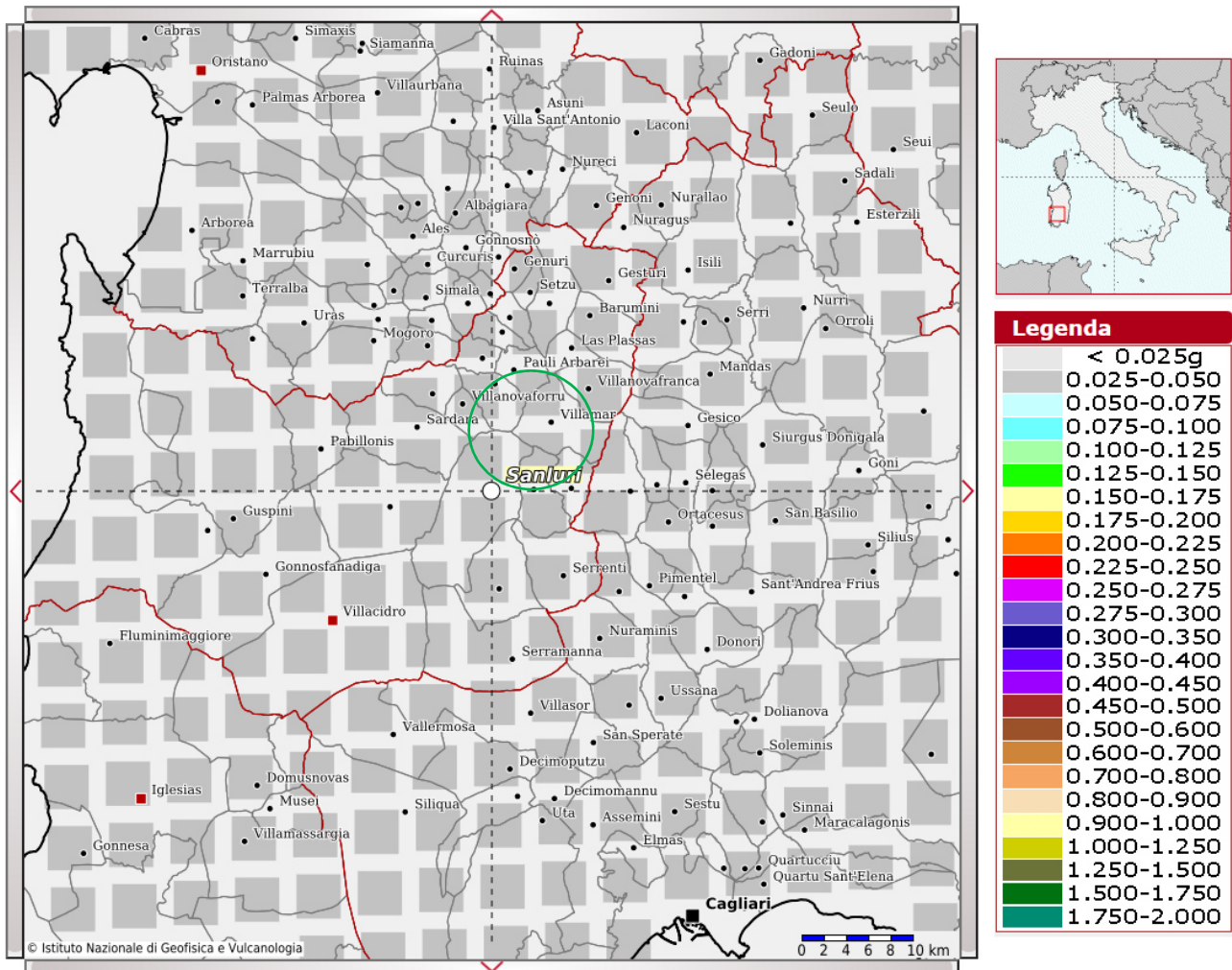
Estratto riferito all'area in oggetto della Mappa Interattiva di Pericolosità Sismica redatta dall'Istituto Nazionale di Geofisica e Vulcanologia (INGV). In verde è evidenziata l'area oggetto della presente relazione.
