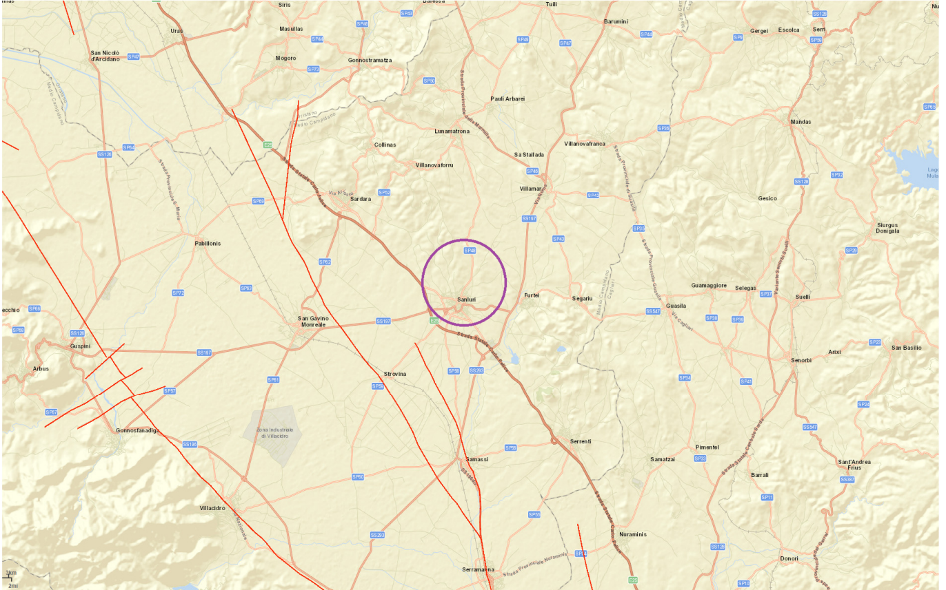
Estratto della carta delle faglie capaci individuate dal progetto ITHACA. In viola è cerchiata l'area interessata dalle nuove opere.
