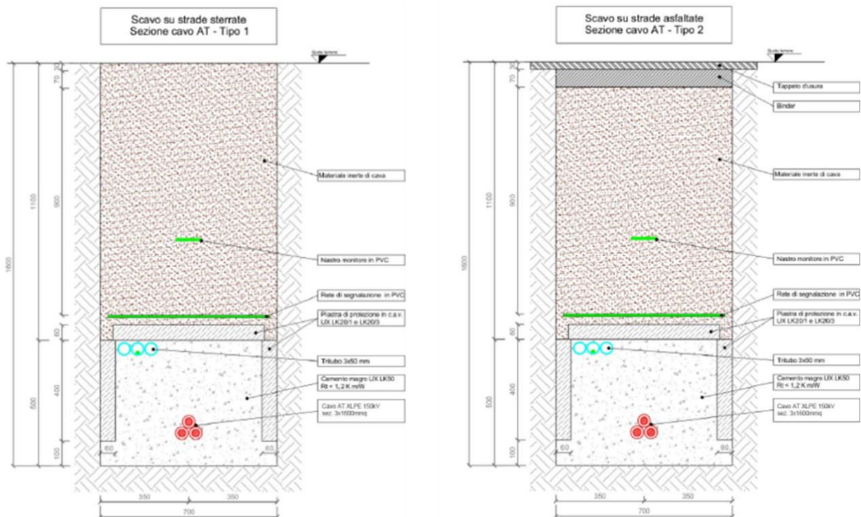
Figura 18. Sezioni tipo cavidotto AT
