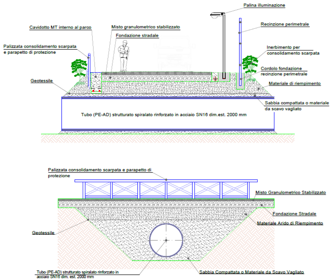
Figura 24. Attraversamenti del reticolo idrografico interni alle aree d'impianto
