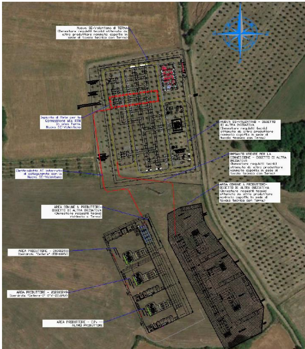
Figura 16. Planimetria della nuova "SE-Valentano" e delle opere utente per la connessione alla RTN
