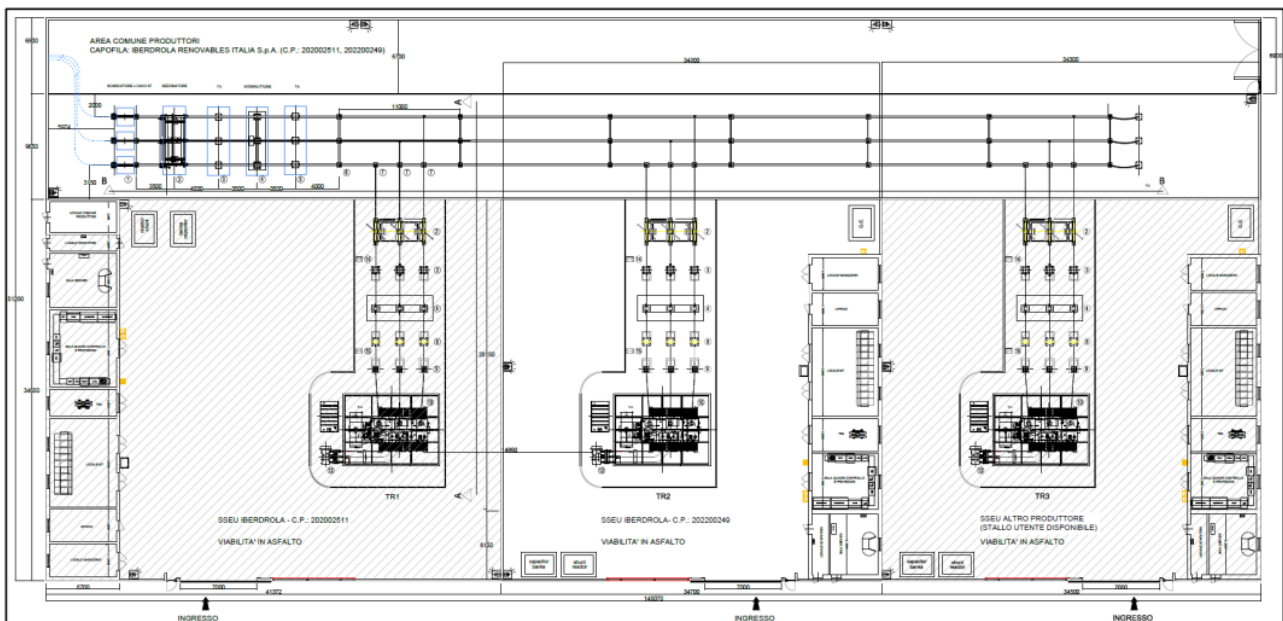
Figura 17. Planimetria della SSEU in progetto e dell'Area Comune Produttori
