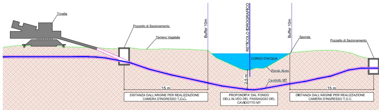
Figura 25. Attraversamenti del reticolo idrografico mediante Trivellazione Orizzontale Controllata (T.O.C.)
