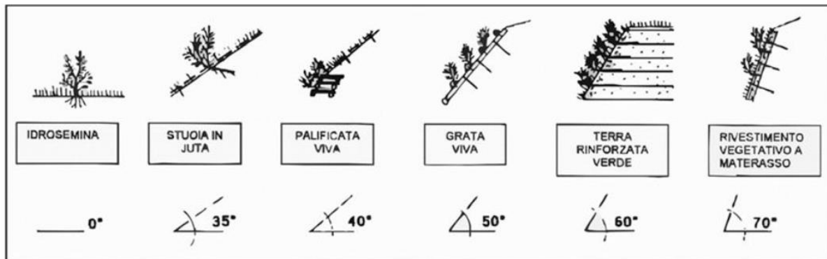
Figura 21. Schematizzazione delle opere di copertura.
