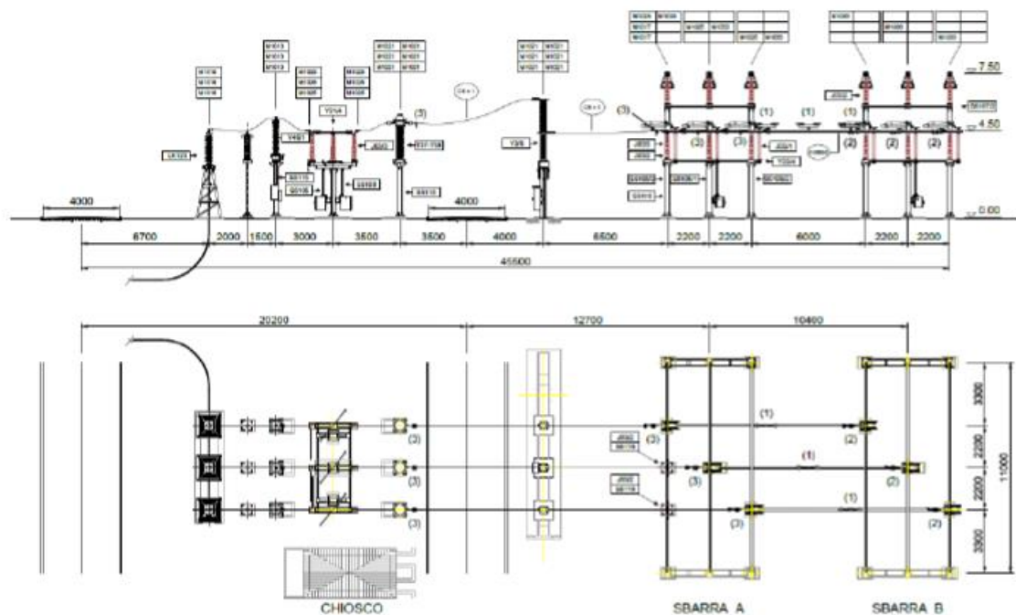
Figura 19. Stallo a 150 kV ubicato all'interno della SE Terna
