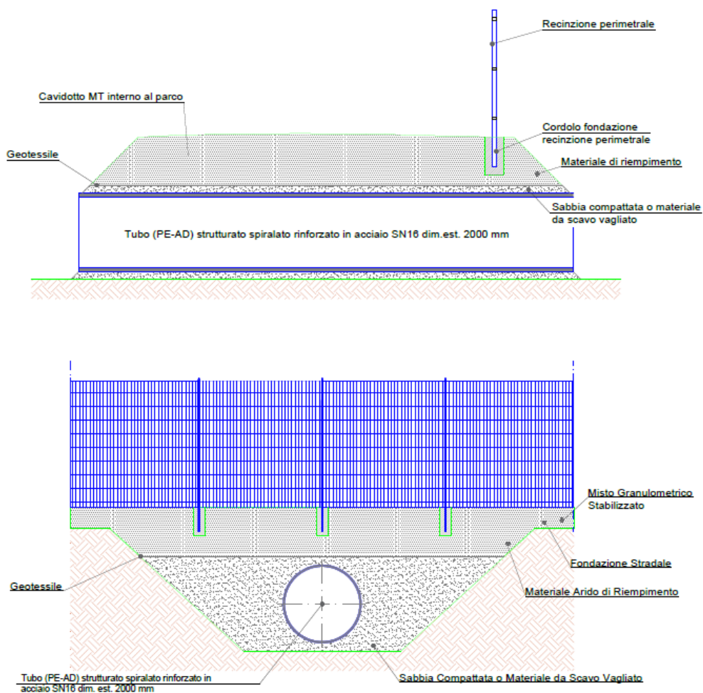
Figura 23. Attraversamenti del reticolo idrografico interni alle aree d'impianto
