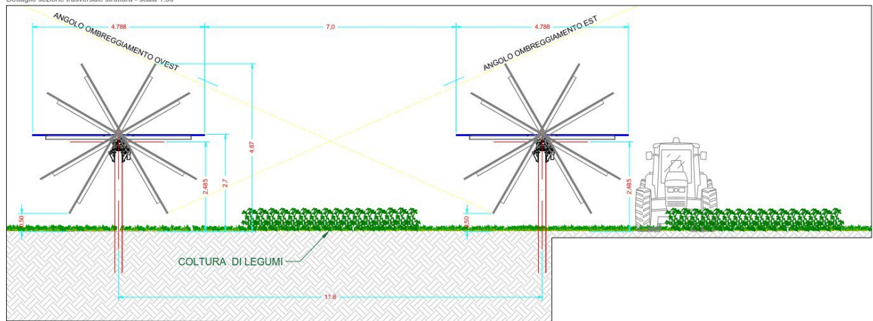
Figura 4: Tipico struttura di sostegno
