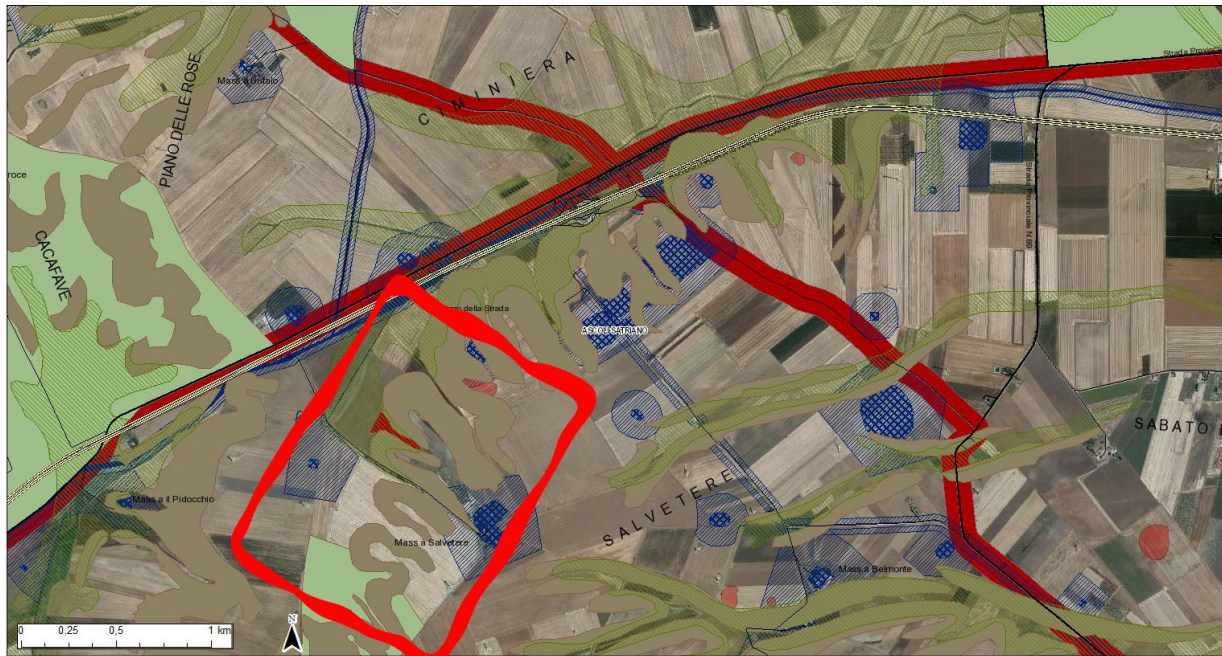
Figura 3 - Area dell'impianto con buffer di 500 m rispetto a beni sottoposti a tutela (PPTR)
