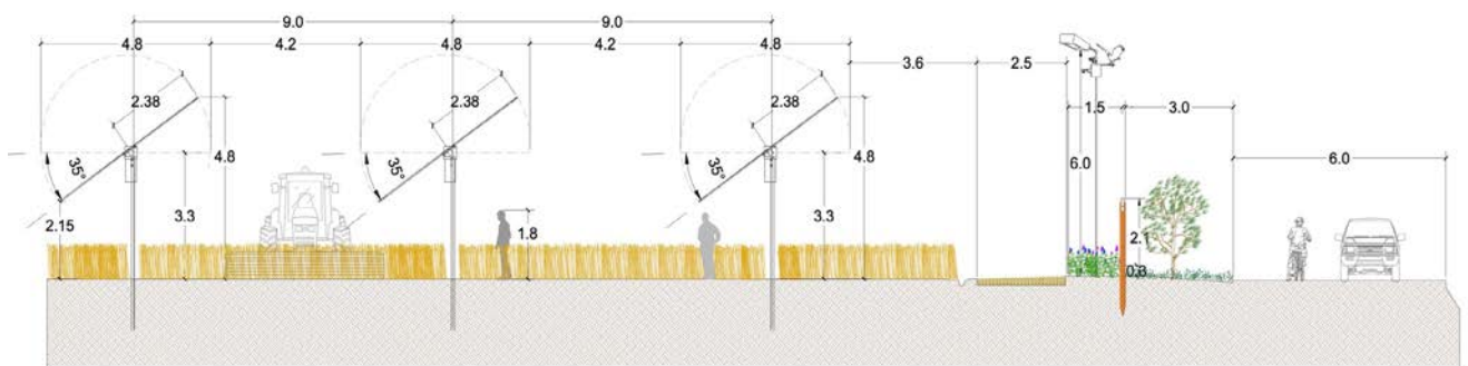
Figura 13 - Sezione dell'impianto agrivoltaico
