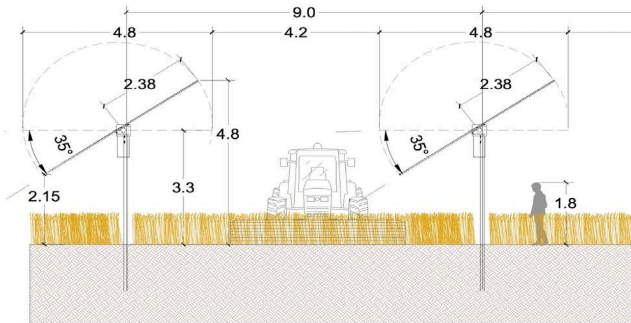
Figura 10 - Sezione dell'impianto agrivoltaico con pannelli tracker.
