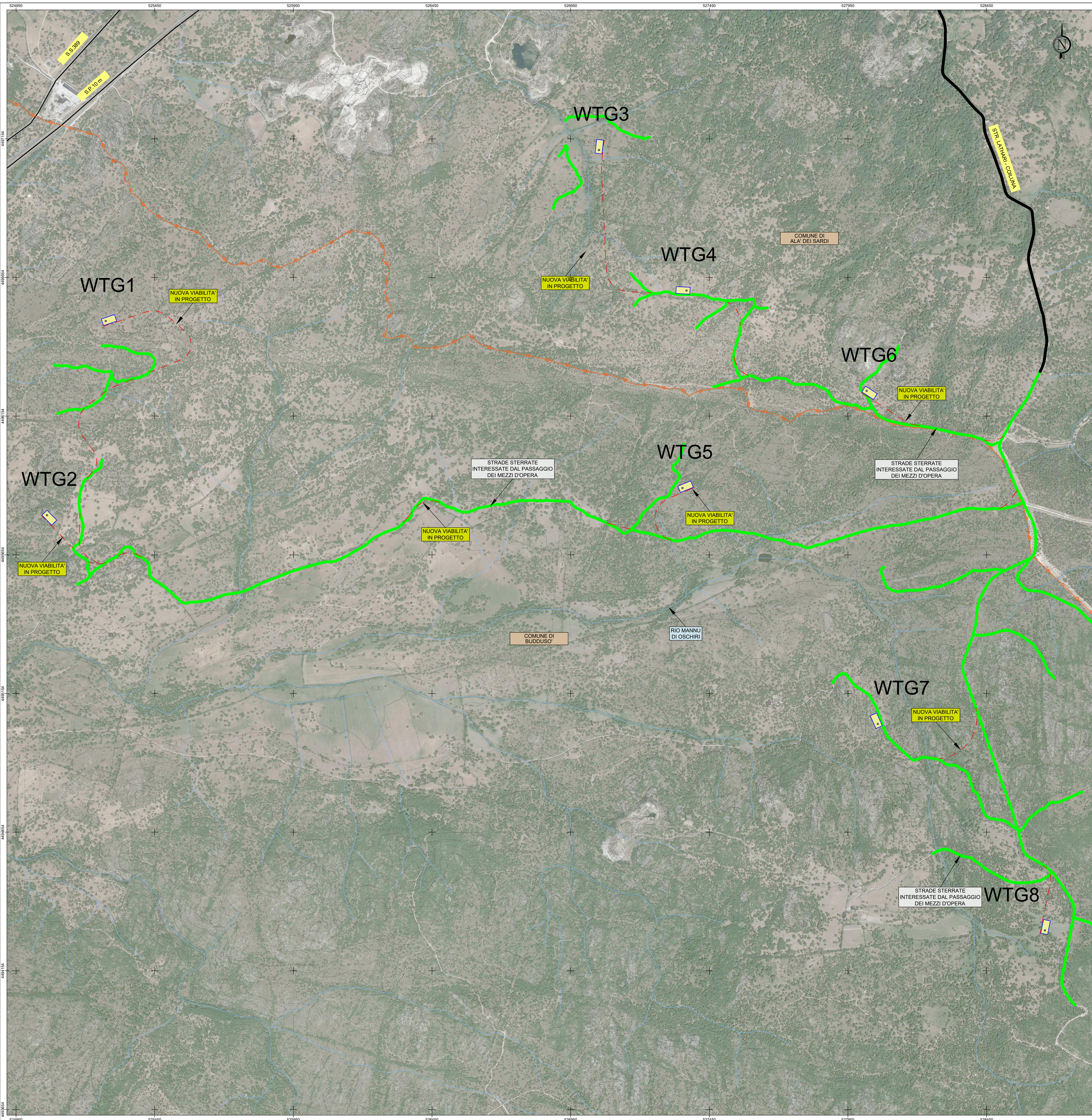
PLANIMETRIA STATO DI FATTO: TAVOLA B Base carta: Carta Tecnica Regionale 1:10.000 e Ortofoto Google Map
