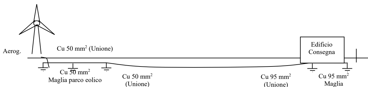
Figura 3 Particolare rete di terra
