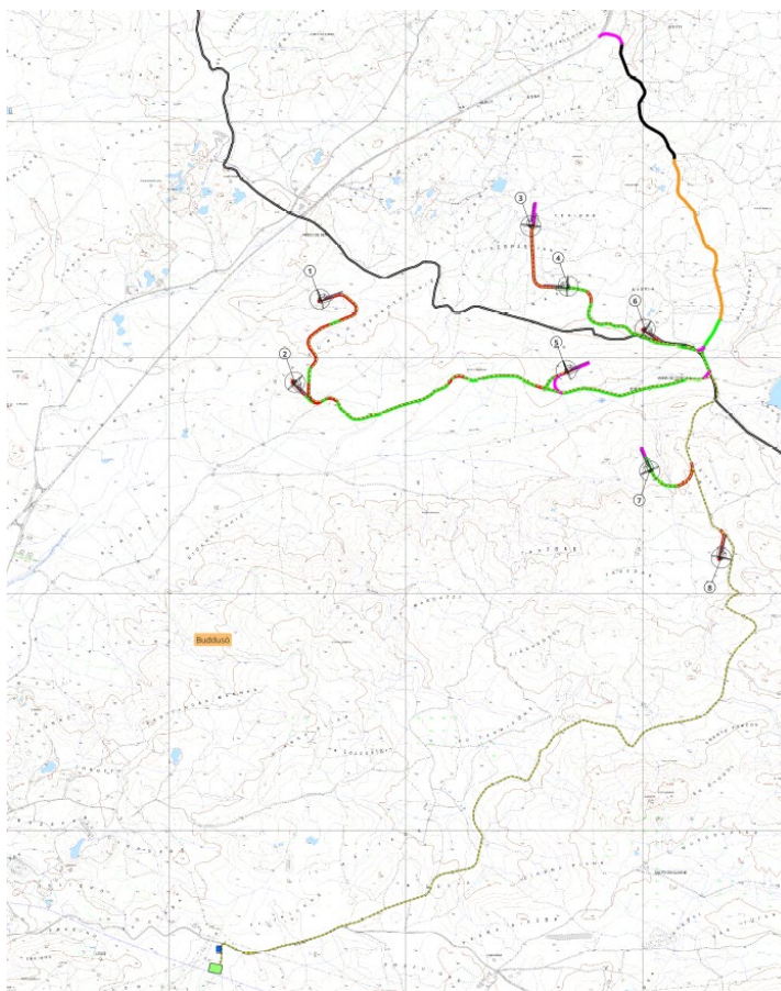
Figura 2 Layout impianto
