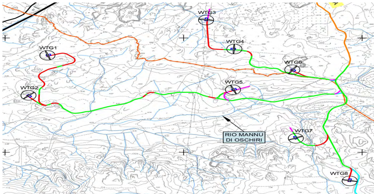
Figura 8 – Viabilità interna parco eolico “Buddusò Sud I” per l’accesso agli aerogeneratori (in arancione strada solo da allargare, in verde le piste esistenti oggetto di solo adeguamento e in rosso i tratti di pista di nuova viabilità; in magenta tratti di pista di cantiere da rimuovere a fine lavori per ripristinare paesaggio presente)
