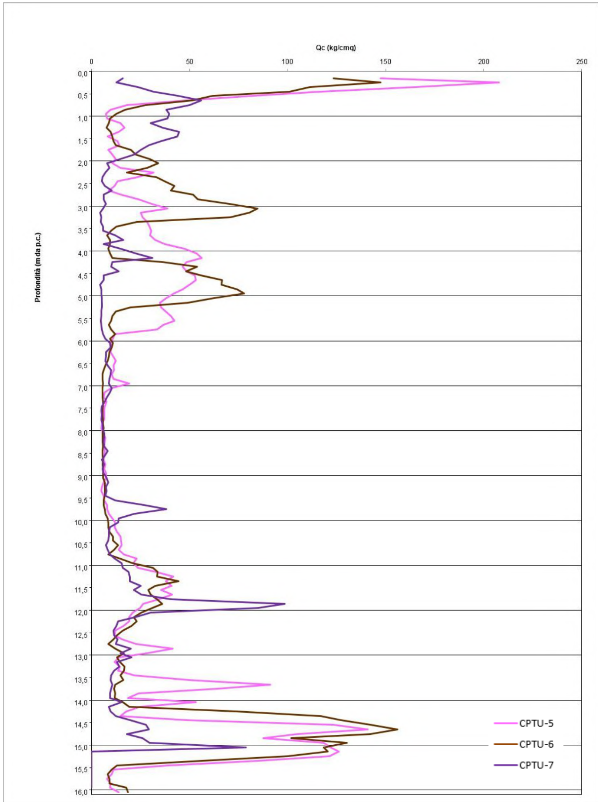
Figura 6-3 - Andamento dei valori di resistenza alla punta Q_c rispetto alla profondità, Area Sud (CPTU-5÷7)
