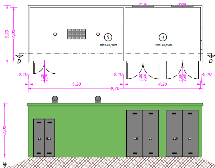
Figura 3-3 – Pianta e profilo delle cabine MT/BT
