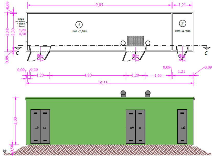
Figura 3-4 – Pianta e profilo della cabina di consegna CHIRON FTV
