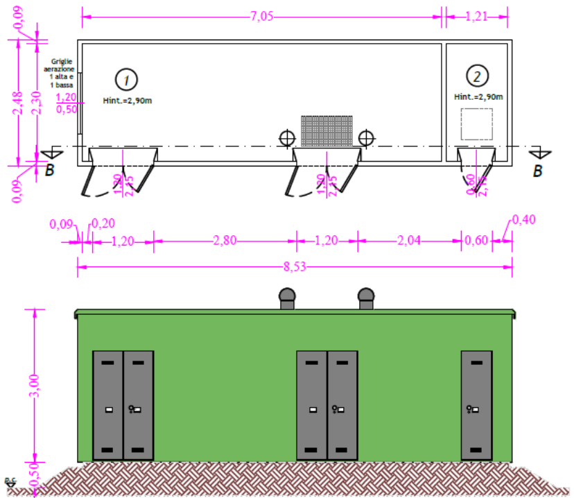
Figura 3-5 – Pianta e profilo della Cabina di consegna PAVIA
