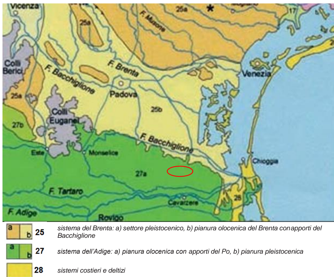
Figura 4-1 – Schema dei sistemi deposizionali della pianura veneto-friulana (Fonte: APAT, Note illustrative della Carta Geologica di Italia alla scala 1:50.000, foglio 148-149, Chioggia-Malamocco)
