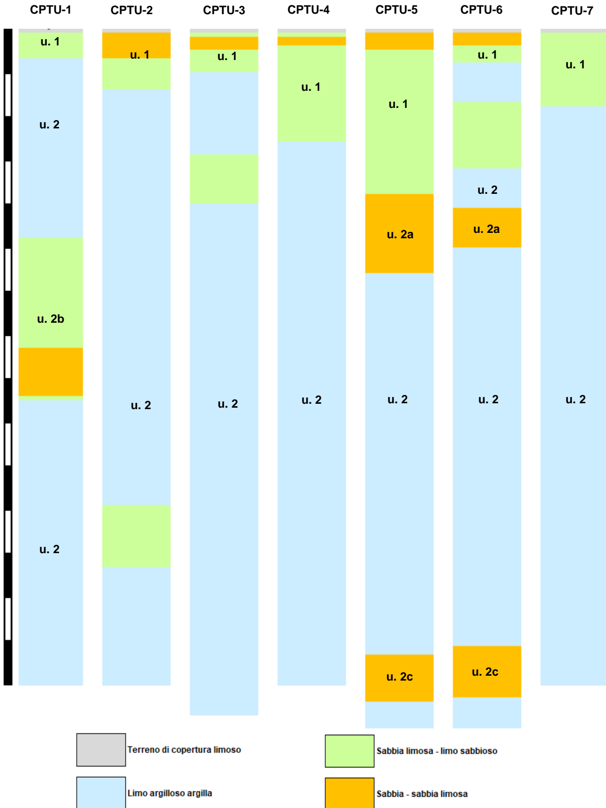
Figura 6-1 – Schema delle unità litologiche riconosciute nel sottosuolo investigato
