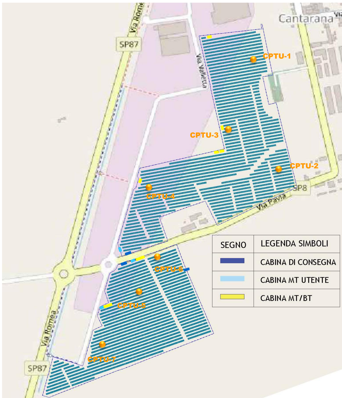
Figura 8-1 - Ubicazione delle cabine e delle indagini geognostiche eseguite
