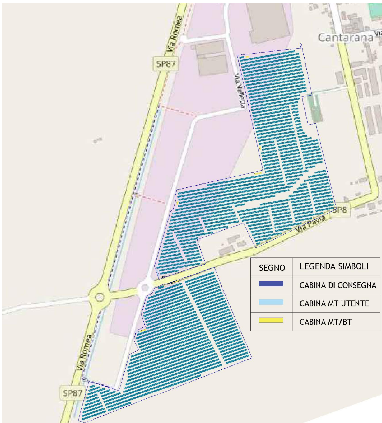
Figura 3-1 - Ubicazione del campo fotovoltaico in progetto
