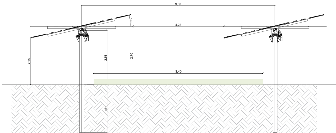
Figura 2 – Prospetto impianto agrivoltaico
