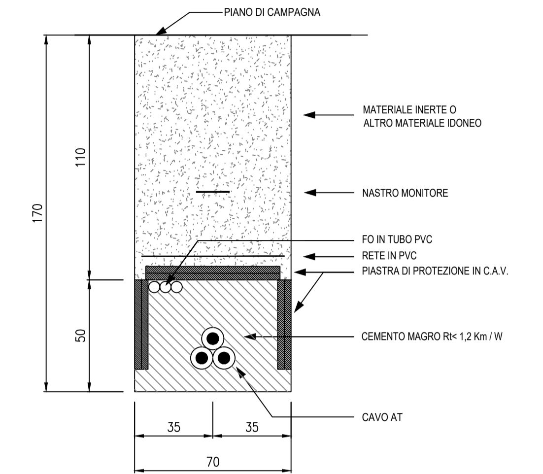
SEZIONE TIPO Posa su TERRENO
