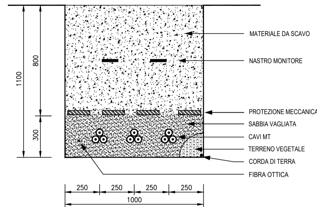
SEZIONE TIPO 3 Terne su TERRENO
