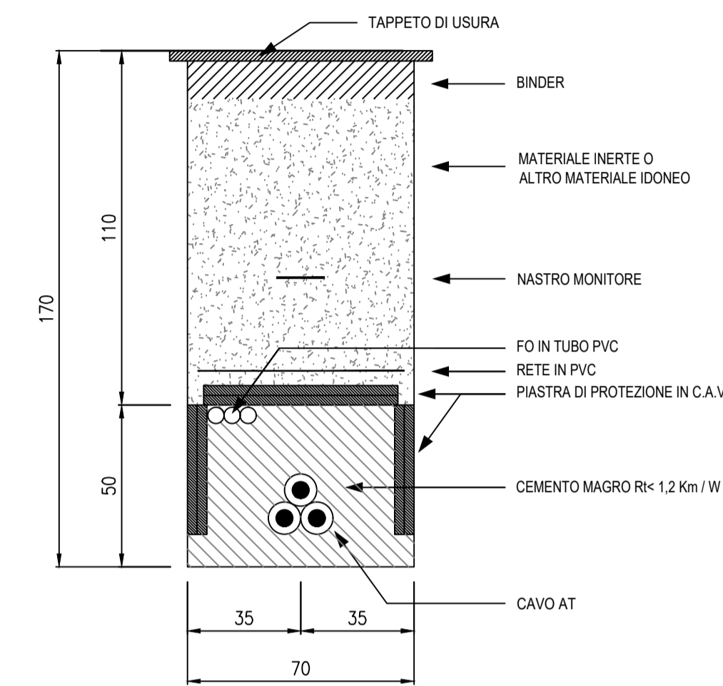
SEZIONE TIPO Posa su STRADA
