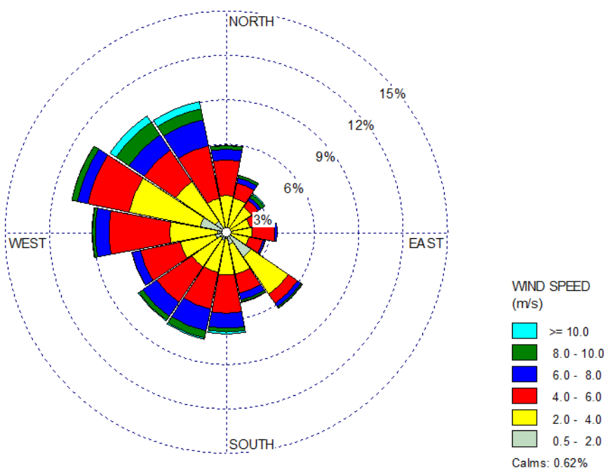
Figura 2 – Rosa venti annuale risultante dall'elaborazione dei dati meteo del modello WRF
