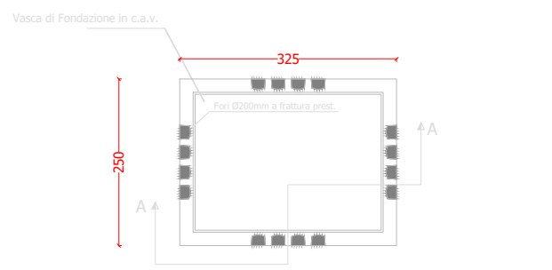
PARTICOLARE VASCA
